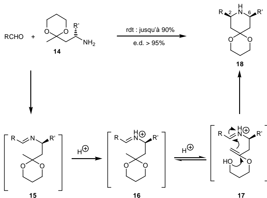
Schéma 1. Synthèse stéréosélective de pipéridines cis -2,6-disubstituées par réaction de Mannich intramolécule.
