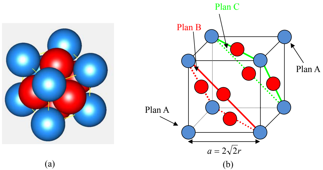
Fig 2.5 (a) Vue compacte d'une maille cube face centrée , (b) vue éclatée d'une maille élémentaire cubique faces centrées ; les billes situées sur les arêtes du cube (billes bleues) comptent pour 1/8 bille, et celles positionnées sur le centre de chaque face (billes rouges) pour 1/2)
