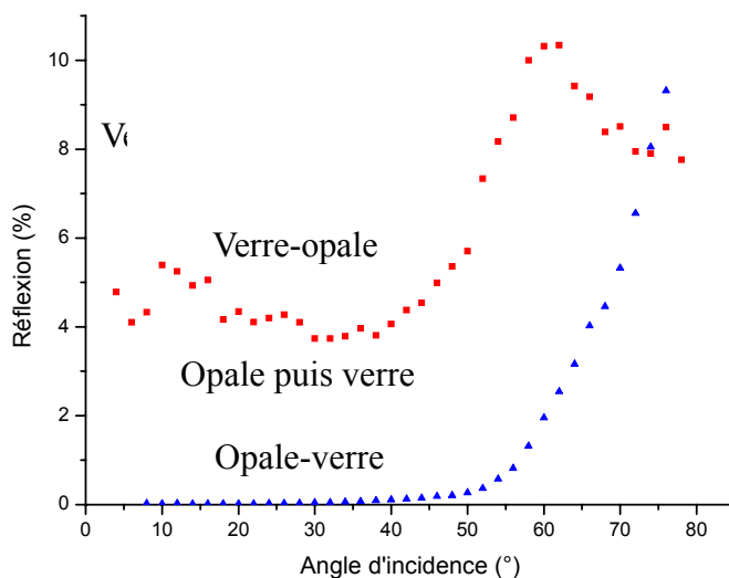
Fig 2.12 Evolution de la réflexion en fonction de l'angle pour une interface air-opale-verre, ou air-verre-opale (conditions expérimentales : \lambda=894 nm, opale de 10 couches de billes de 1 \mu\text{m} de diamètre, polarisation TE) [échantillon différent de celui mis en cellule présenté au chap. 5 et 6] (courbe réalisée par E. Moufarej).
