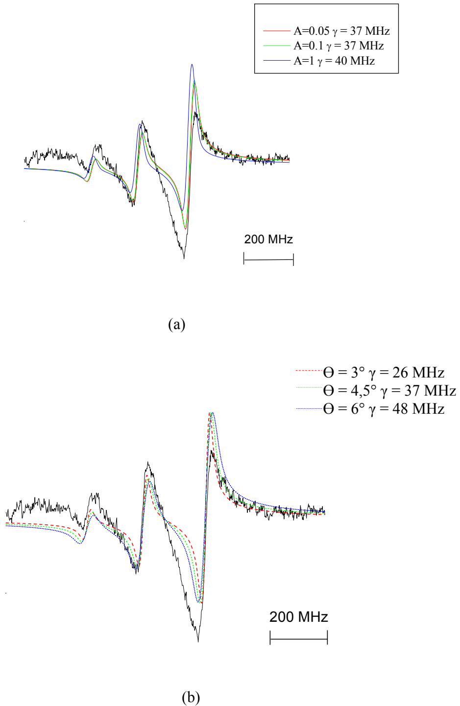
Fig 5.15 Spectre de la réflexion sélective sur l'opale de la raie D_2 ( F=4 ) en incidence normale et fits d'un spectre de réflexion sélective : (a) pour différents paramètres de van der Waals A (pour \Theta_{fi}=4,5^\circ ) (b) pour différents angles d'incidence (pour A=0,05 ).
