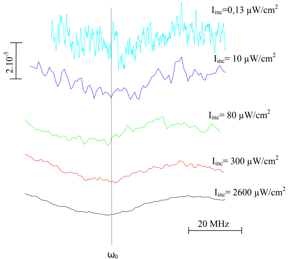
Fig 5.27 : Observation de la structure sub-Doppler ( S_{R_{FM}}/I_R ) pour différentes intensités du faisceau incident, opale composée de billes de 1\mu\text{m} de diamètre et de 20 couches d'épaisseur (transition 3-4 de la raie D_1 du césium, polarisation TM , pour une incidence de 40^\circ ).
