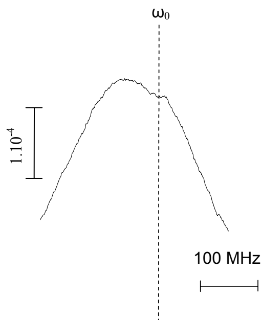
Fig 5.22 Spectre de réflexion sélective ( SR_{FM}/I_R ) pour \lambda = 894 \text{ nm} et \Theta = 40^\circ , sur une opale de 10 couches de billes de 1 \mu\text{m} (transition 3-4 de la raie D_1 du césium en polarisation TE).
