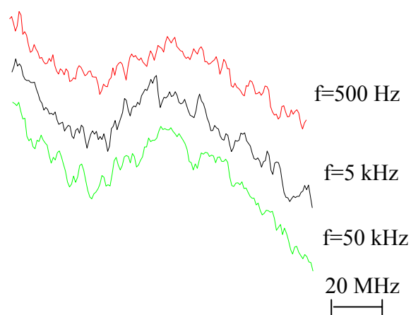
Fig 5.25 Evolution du spectre de réflexion sélective avec la fréquence de modulation, opale de 20 couches de billes de 1 \mu\text{m} de diamètre, pour une incidence de 40^\circ .
