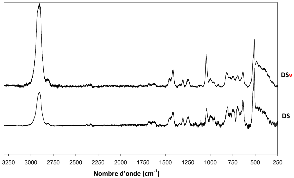
Figure 8 – Spectres Raman de la charge DS avant et après 21h30 de vieillissement
