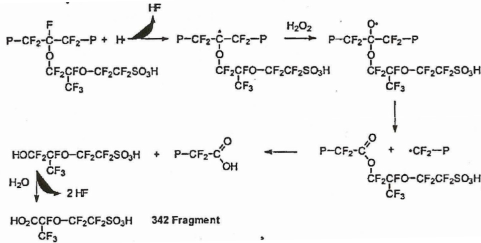
Schéma 2 – Coupure possible de la chaîne principale suite à l'attaque d'un radical H\cdot 40
