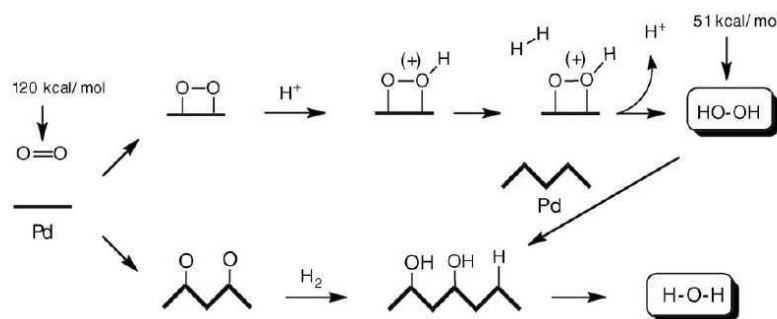
Figure 5 – Mécanisme probable de la synthèse de H 2 O 2 catalysée sur palladium 34
