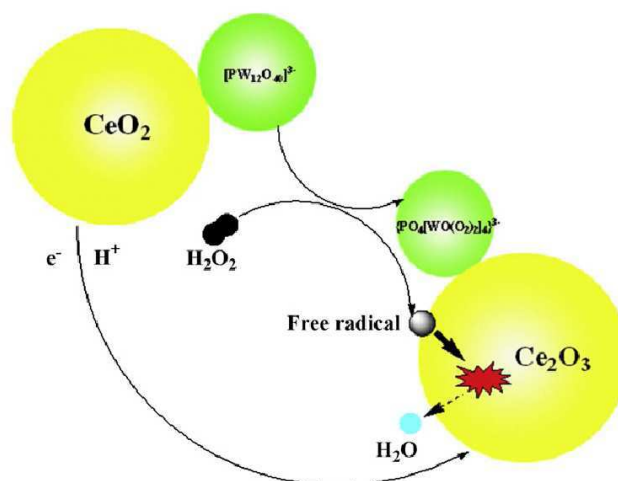
Schéma 12 – Mécanisme de production de radicaux Hydroxyles et hydroperoxydes à partir des ions [PW_{12}O_{40}]^{3-} 80
