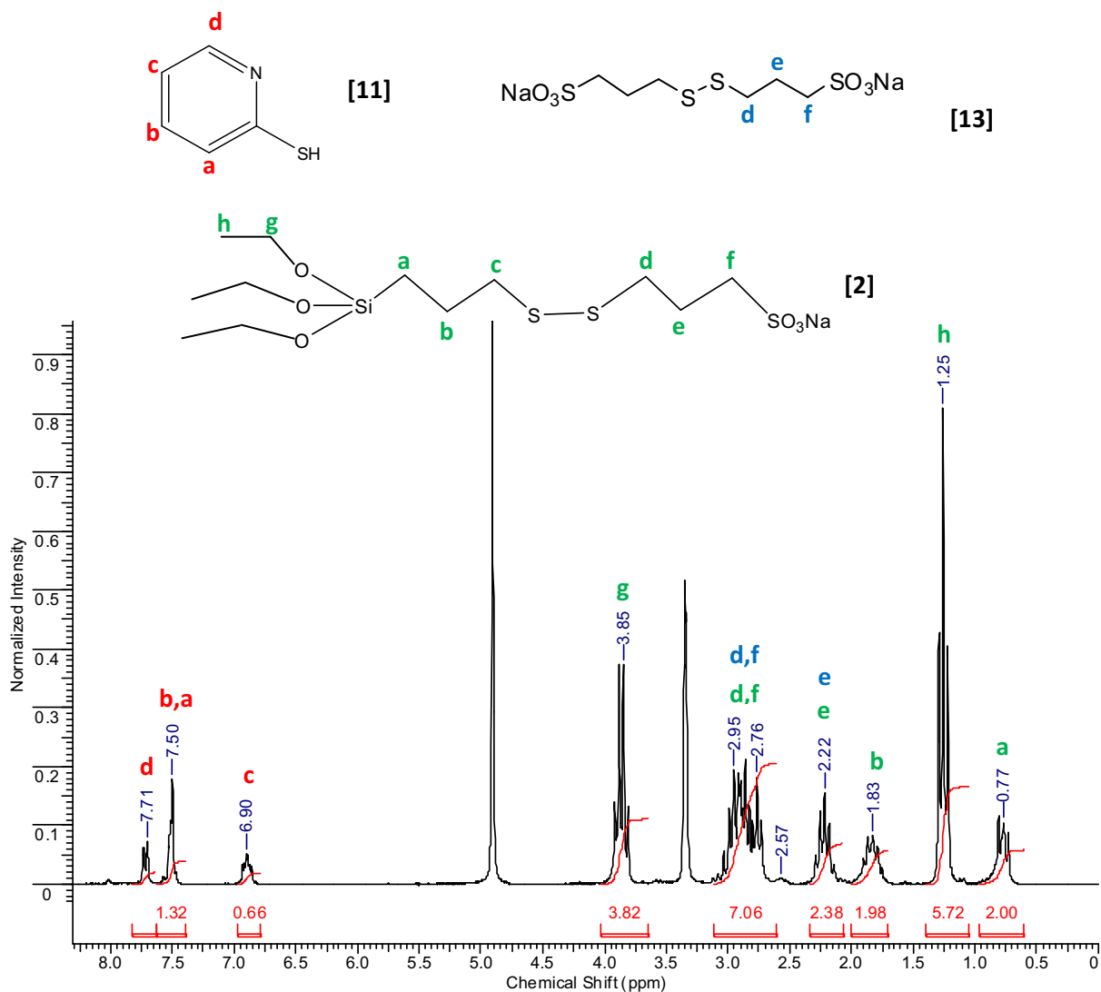
Figure 7 – Spectre RMN 1 H du synthon DSs dans le Méthanol d4 à 25°C
