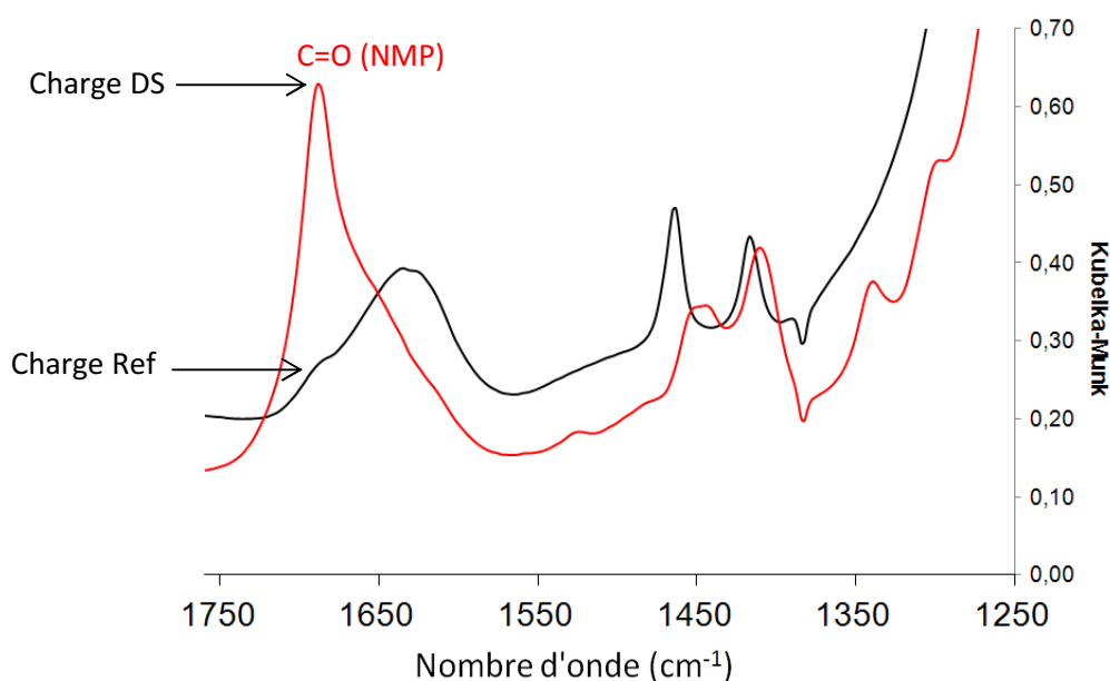
Figure 19 – Superposition de la région 1750-1250 cm -1 des spectres DRIFT des charges Ref (noir) et DS (rouge)
