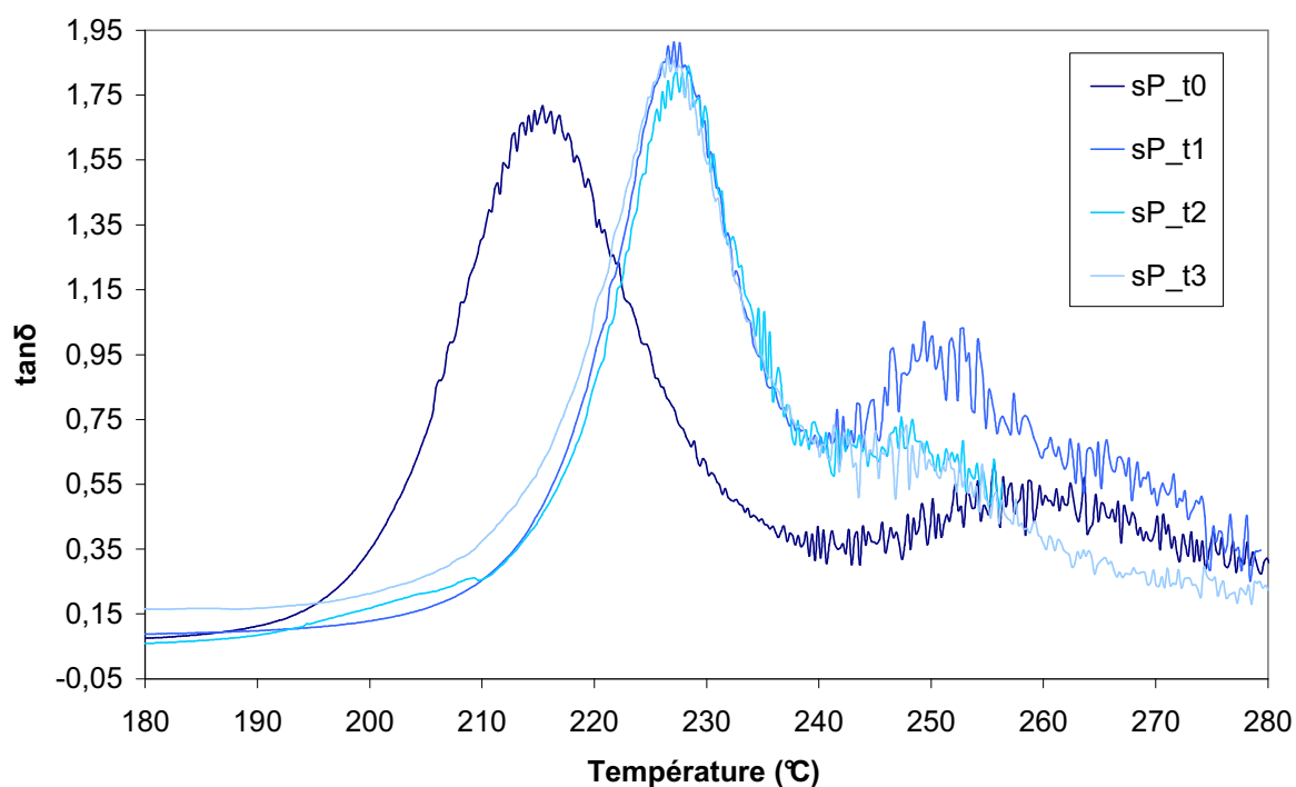
Figure 16 – Superposition des courbes de \text{tan}\delta , obtenues par DMA, de la membrane sP à différents temps de vieillissement
