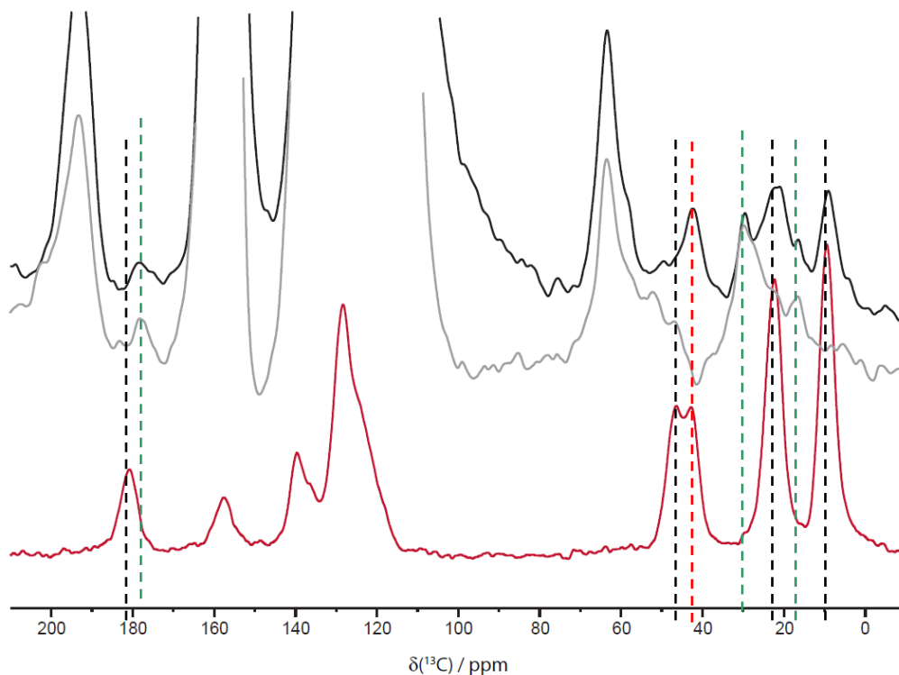
Figure 5 – Spectres RMN solide ^{13}\text{C} CPMAS de la charge THP (rouge), spectre RMN ^{13}\text{C} SELTICS des membranes sP (gris) et THP (noir). (-----) pics de THP (-----) pic d'oxydation de THP (-----) pic de NMP
