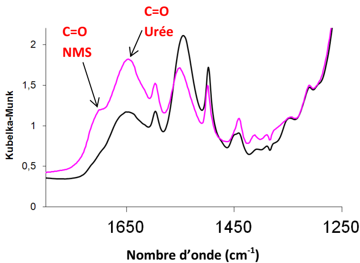
Figure 10 – Région 1750\text{-}1250\text{ cm}^{-1} du spectre DRIFT de la charge THP avant (noir) et après vieillissement (rose). Spectre complet Annexe C6
