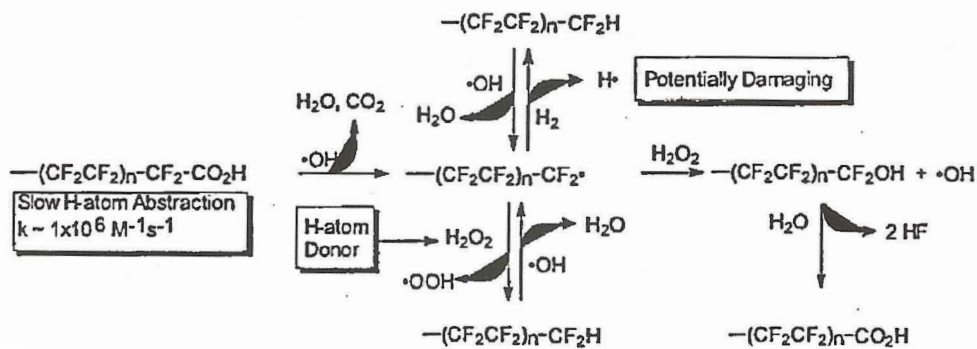
Schéma 3 – Révision du mécanisme de dépolymérisation de la chaîne principale du Nafion® 40
