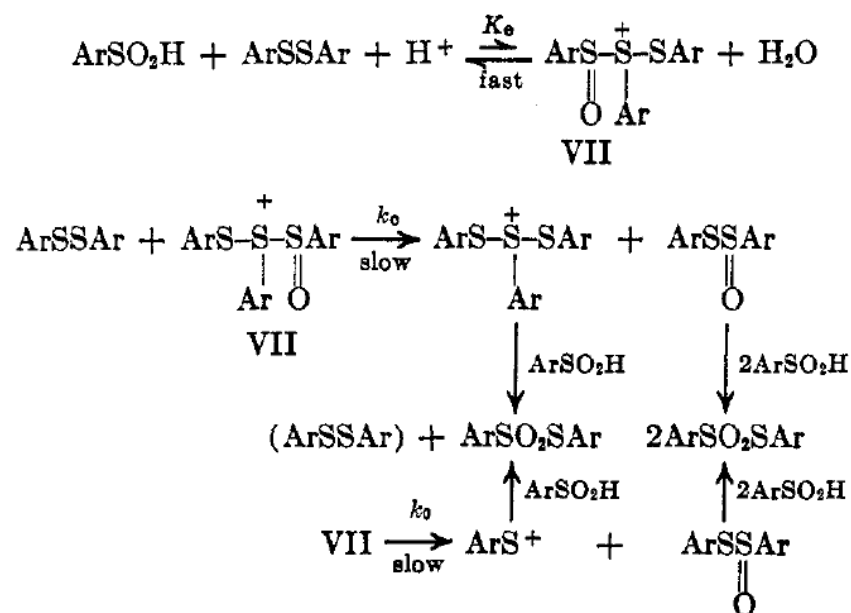
Schéma 16 – Réaction d'un acide sulfinique avec un disulfure catalysée par un acide fort 93
