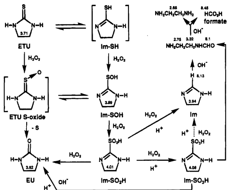
Schéma 19 – Voies d'oxydation de l'éthylène thiourée dans H_2O_2 à 30^\circ C et à différents pH (5, 7 et 9) 97
