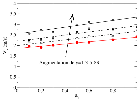
FIGURE 6.73 – Vitesse selon ( Ox ) relative en fonction du frottement particule/particule ( x = 33R , \Omega = 500\text{tours/min} , t = 0.015\text{s} , \mu = 0.2 , y = 1-3-5-8R ).
