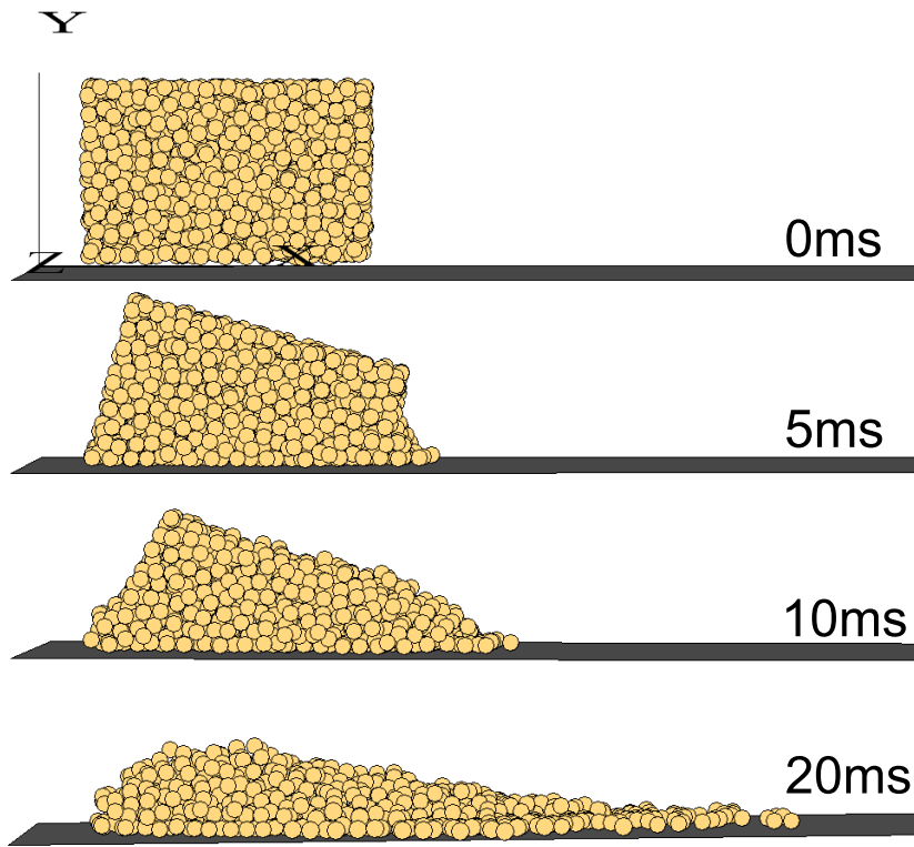
FIGURE 6.3 – Ecoulement de l'amas granulaire à différents temps (500tours/min, \mu = 0.1 , \mu_b = 0.2 ).
