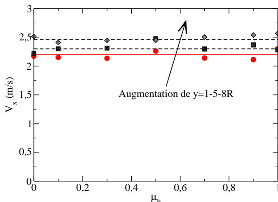
FIGURE 6.52 – Vitesse selon ( Ox ) relative en fonction du frottement particule/particule ( x = 33R , \Omega = 500\text{tours/min} , t = 0.015\text{s} , \mu = 0.2 , y = 1-5-8R ).
