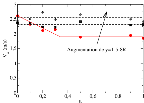
FIGURE 6.51 – Vitesse selon ( Ox ) relative en fonction du frottement particule/pale ( x = 33R , \Omega = 500\text{tours/min} , t = 0.015\text{s} , \mu_b = 0.2 , y = 1-5-8R ).
