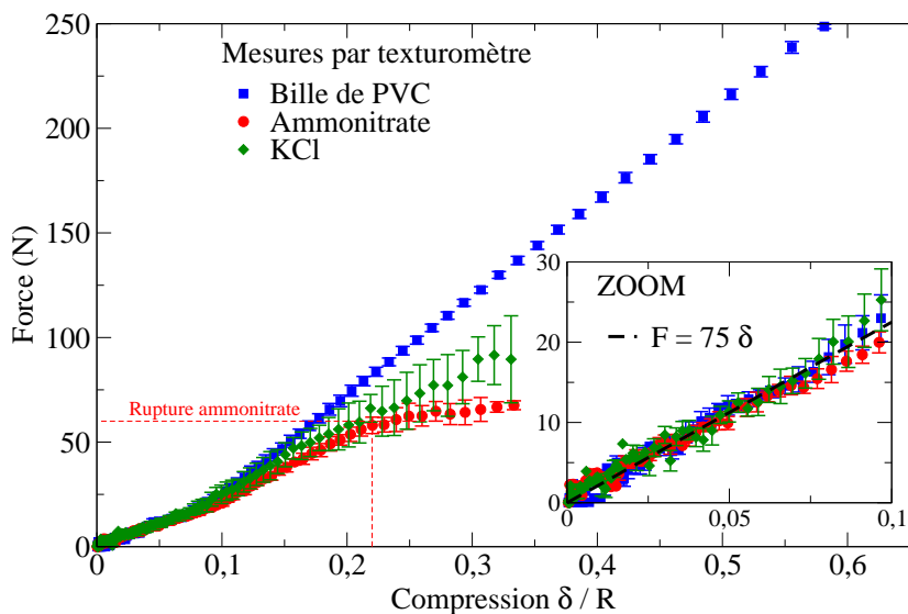
FIGURE 2.6 – Force appliquée en fonction de la compression résultante. Comparaison des particules plastiques, d’Ammoniate et de KCl. Zoom sur les faibles déformations ( \delta < 0.1R , R=3\text{mm} ) et interpolation par une loi linéaire.
