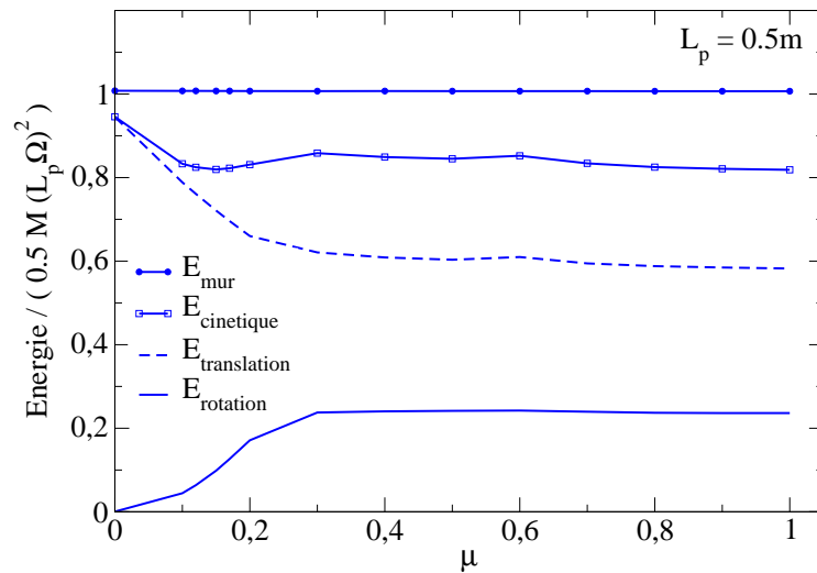
FIGURE 6.30 – Énergie cinétique et ses deux composantes (translation + rotation) en fonction du frottement particule/pale à une distance x de 0.5\text{m} ( \mu_b = 0.4 ).
