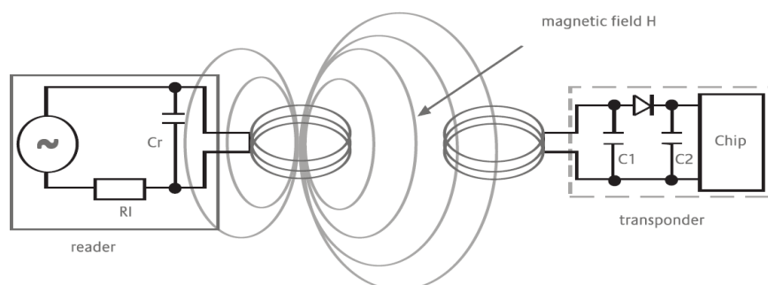
Figure I-6 – Le couplage inductif vu par Klaus Finkenzerler [FIN2003]
