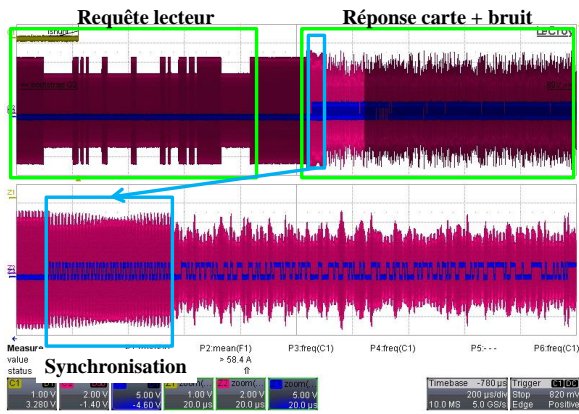
Figure V.34 – Effet du bruit sur le champ magnétique
