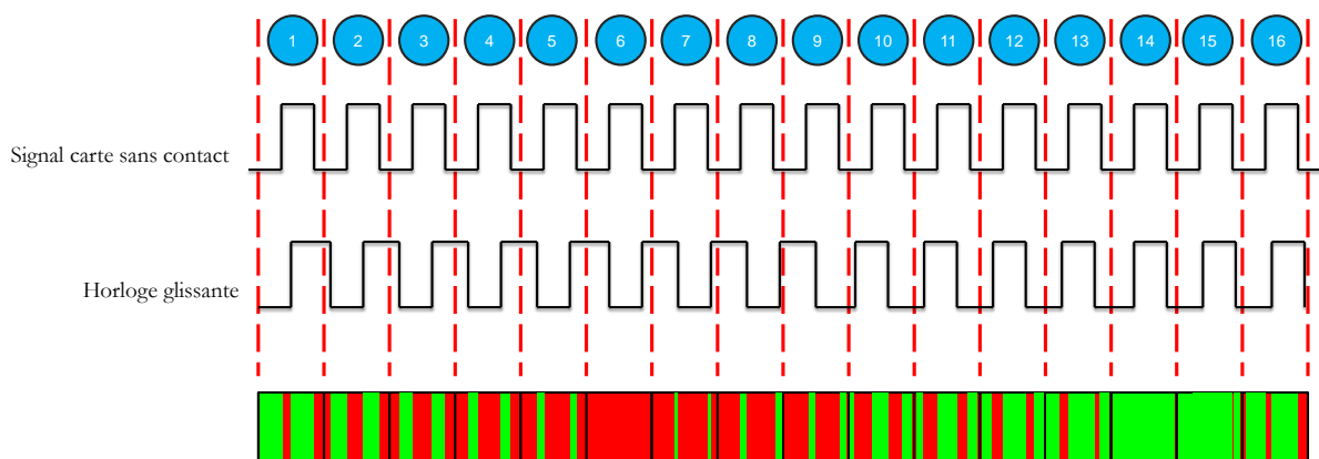
Figure V.22 – Phase de synchronisation sur 16 périodes
