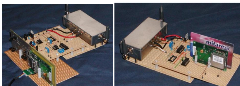
Figure I-14 – Attaque relais selon Hancke
