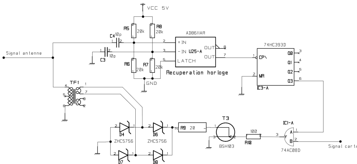
Figure Annexes-22 – Proxy : voie descendante
