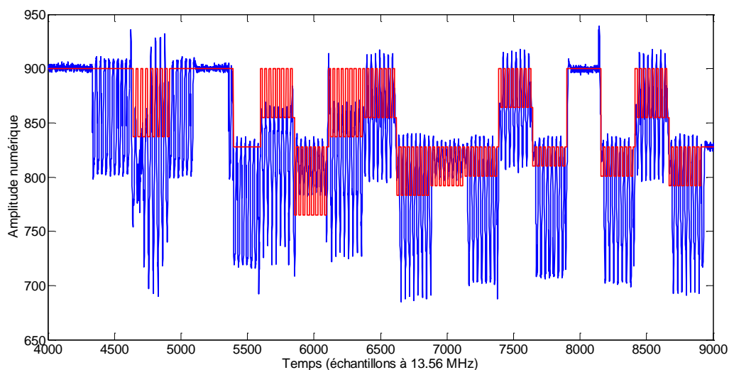
Figure V.45 – Résultats obtenus (bleu : échantillons en sortie du CAN ; rouge : consigne de bruit)
