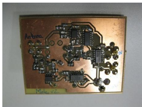
Figure II.47 – Le proxy : circuit et topologie du circuit électronique
