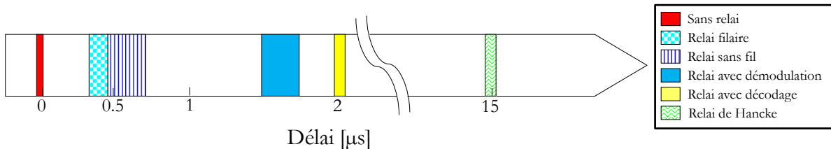
Figure II.57 – Délai introduit par les différents relais
