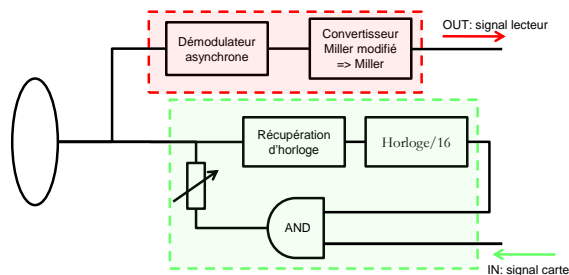
Figure II.47 – Le proxy : circuit et topologie du circuit électronique
