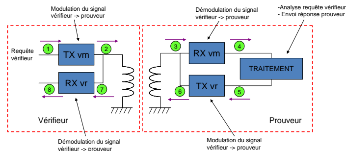
Figure III-2 – Système de transmission entre le prouveur et le vérifieur
