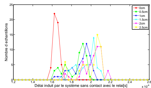
Figure III-40 – Délais obtenus pour le scénario relais filaire en fonction de la distance entre l'antenne 2 du relai et la carte
