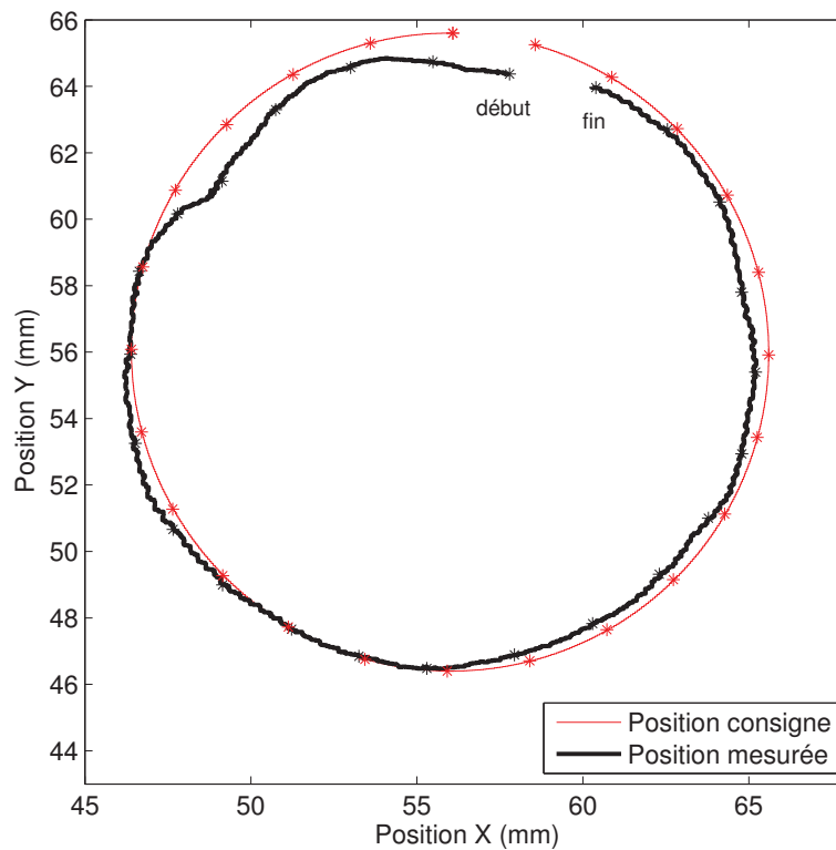
FIGURE 4.19 – Trajectoire de l'objet RAE sous un contrôle PID, en réponse une trajectoire circulaire de consigne. Entre deux instants marqués par un astérisque, une demi-seconde s'est écoulée.
