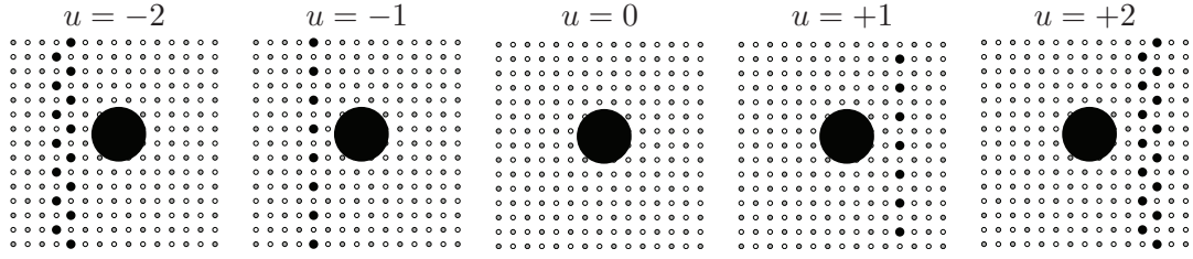
FIGURE 3.12 – Le signal de commande u est un entier qui représente le nombre de colonnes de jets d’air à activer. Il peut être positif ou négatif suivant la position relative entre les jets d’air et l’objet. Un rond gris représente un trou de lévitation, un petit rond noir représente un jet d’air de traction actif et un petit rond blanc représente un jet d’air de traction inactif. Le gros rond noir représente l’objet à convoier.
