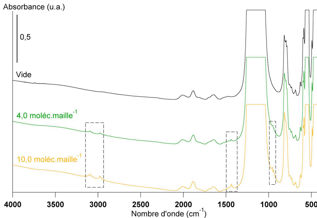
Figure 8.2 : Spectres infrarouges obtenus avec le second dispositif expérimental dans le cas de l'adsorption de l'éthylène sur la silicalite-1 à 298 K, aux remplissages de 0, 4 et 10 moléc.maille -1 (zones encadrées : bandes de l'éthylène adsorbé).
