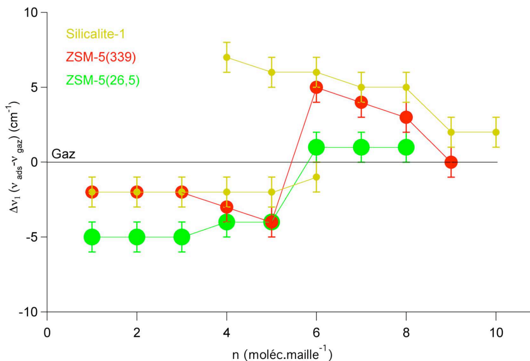
Figure 8.35 : Evolution de la position de la bande \nu_1 ( \nu_{CH} ) du trichloroéthylène en fonction du remplissage dans le cas des zéolithes ZSM-5 de rapport Si/Al 26,5 et 339 et sur la silicalite-1.
