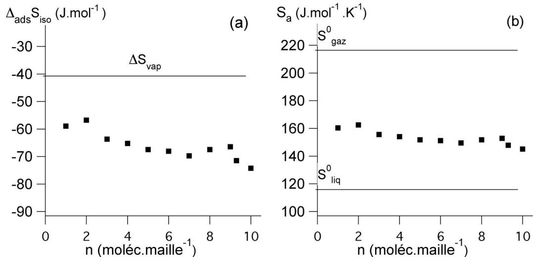
Figure 7.3 : Courbes de variation (a) de l'entropie isostérique d'adsorption de l'éthylène sur la silicalite-1 et (b) de l'entropie molaire de la phase adsorbée, en fonction du remplissage.
