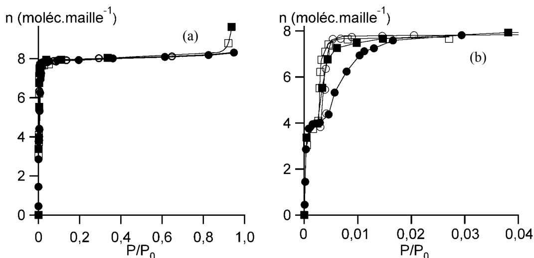
Figure 7.9 : Isothermes d'adsorption / désorption du p-xylène sur la silicalite-1 à 298 K, (a) dans tout le domaine de pression relative exploré et (b) dans le domaine des basses pressions relatives (● : échantillon en poudre, ■ : échantillon pastillé, symboles pleins : données expérimentales d'adsorption, symboles évidés : données expérimentales de désorption).
