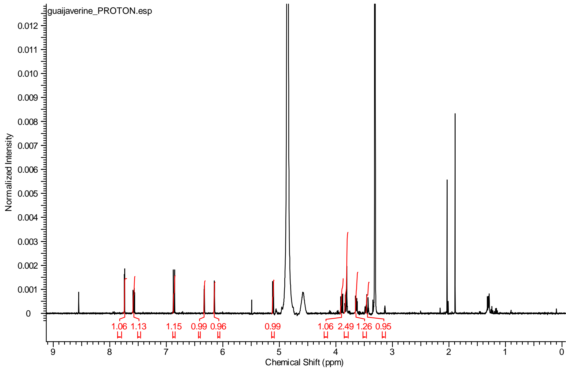
Spectre de RMN ^1\text{H} de la guajaverine (quercitine-3- O - \alpha -L-arabinopyranoside) (5) dans le \text{CD}_3\text{OD}
