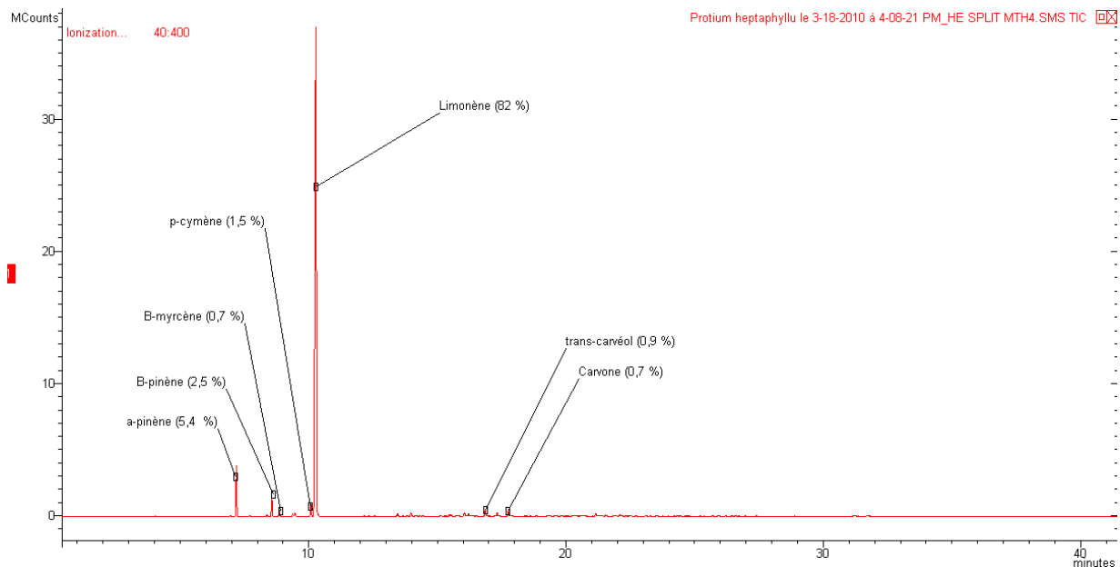
Figure 58 : Chromatogramme en phase gazeuse et molécules majoritaires de l'huile essentielle de fruits verts de Protium heptaphyllum (colonne VF-5ms)
