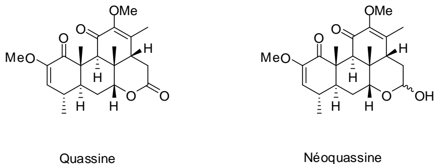
Figure 24 : Structure de la quassine et de la néoquassine, premiers quassinoïdes isolés de Q. amara
