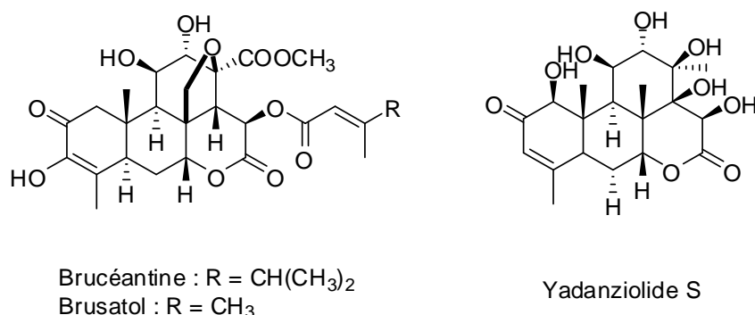
Figure 25 : Structures de la brucéantine, du brusatol et du yadanzolide S
