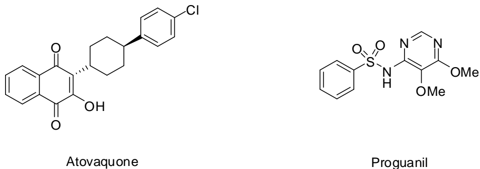
Figure 19 : Structures de l'atovaquone et du proguanil, molécules utilisées en combinaison dans la Malarone ®
