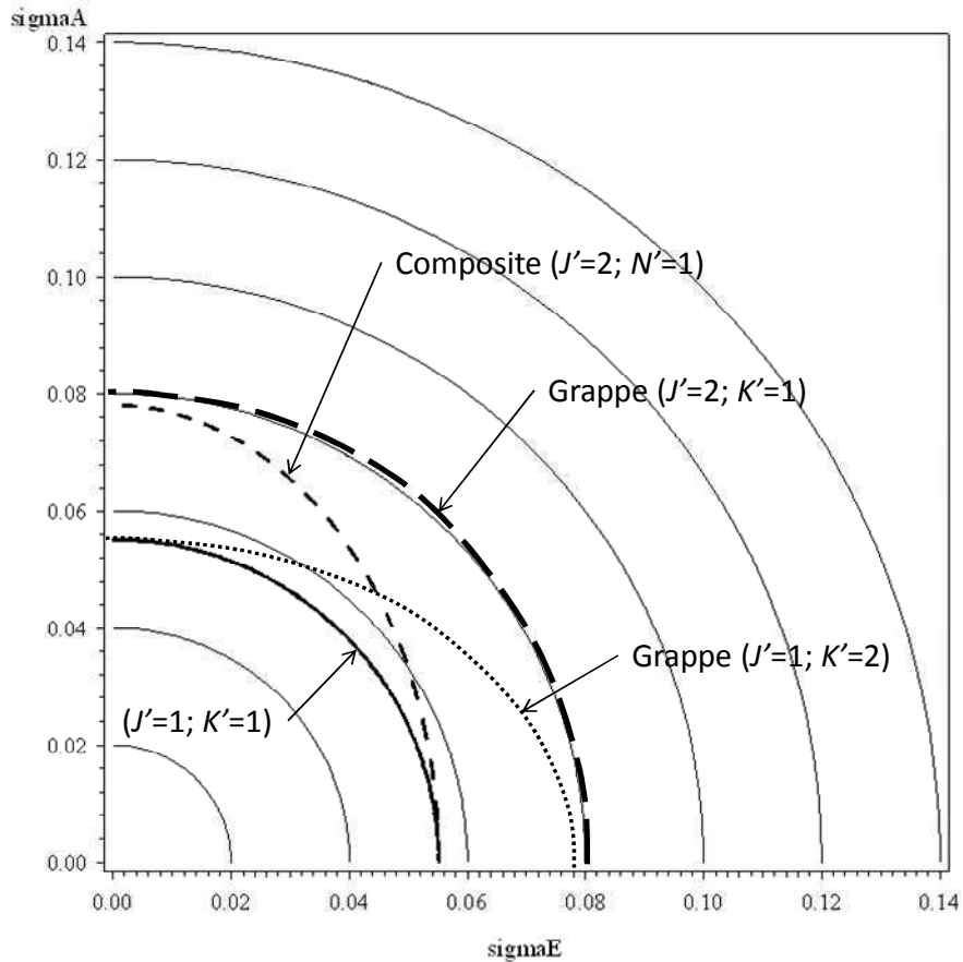
Figure IV-5 : Les différents types de courbe d'iso-variances ayant permis de déterminer le mode opératoire optimum.
