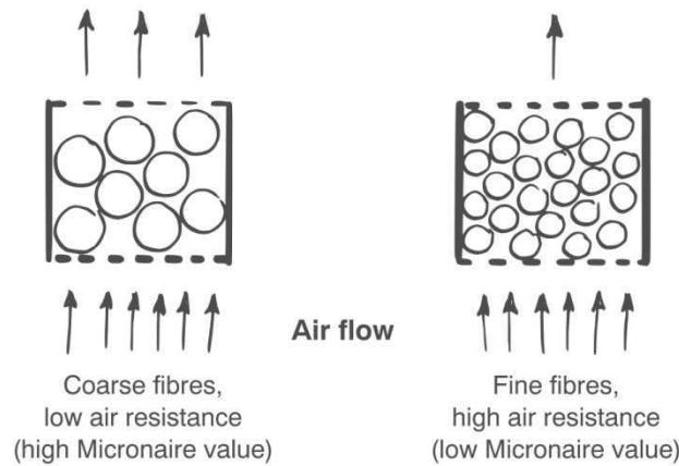
Figure III-7 : Principe de mesure du micronaire.
