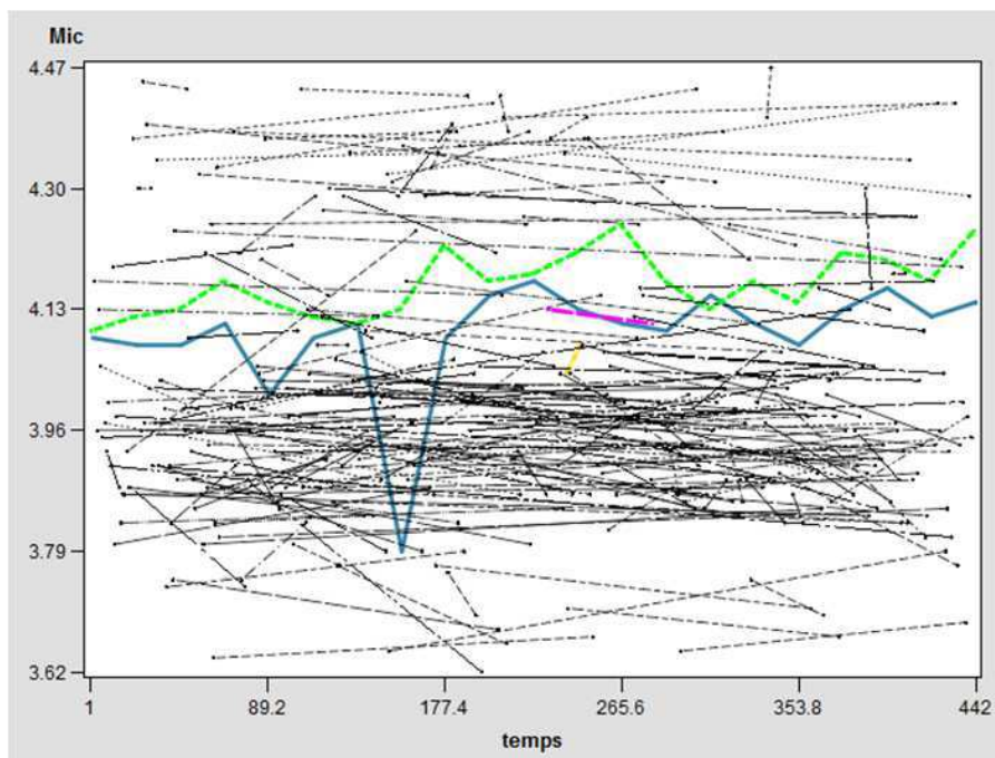
Figure V-4 : Mic des matières de références et des deux répétitions de mesures par échantillon dans la situation C2G3, saison 1.
