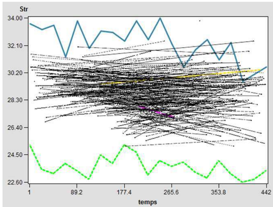
Figure V-2 : Str (g/tex) des matières de références et des deux répétitions de mesures par échantillon dans la situation C4G1, saison 1. Evolutions comparées des mesures obtenues sur les standards (LS en traits pleins épais, SW en pointillé épais) et sur les échantillons analysés. On ne note pas de parallélisme entre ces évolutions sur les trois figures de ce type.
