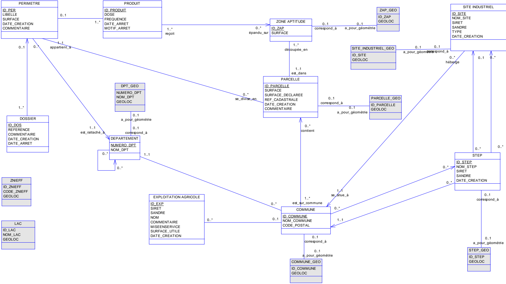
Figure 44. Extrait simplifié du diagramme de classe de SIGEMO
