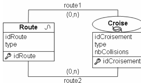
Figure 14. Schéma MADS d’une classe spatiale et spécification d’une contrainte topologique “TopoCross” réflexive sur cette classe [PAR06]
