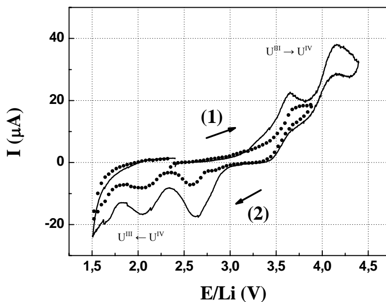
Figure II.21 : Voltampérogrammes du troisième et cinquième cycle d'une électrode composite \text{LiU}_4\text{F}_{16} / PVDF / noir de carbone (86/9/5 % en masse) (électrolyte PC- \text{LiClO}_4 1M).
