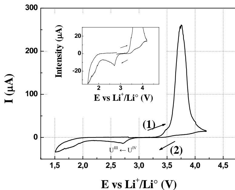
Figure II.20 : Voltampérogramme du premier cycle d'une électrode composite \text{LiU}_4\text{F}_{16} / PVDF / noir de carbone (86/9/5 % en masse) (électrolyte PC- \text{LiClO}_4 1M).
