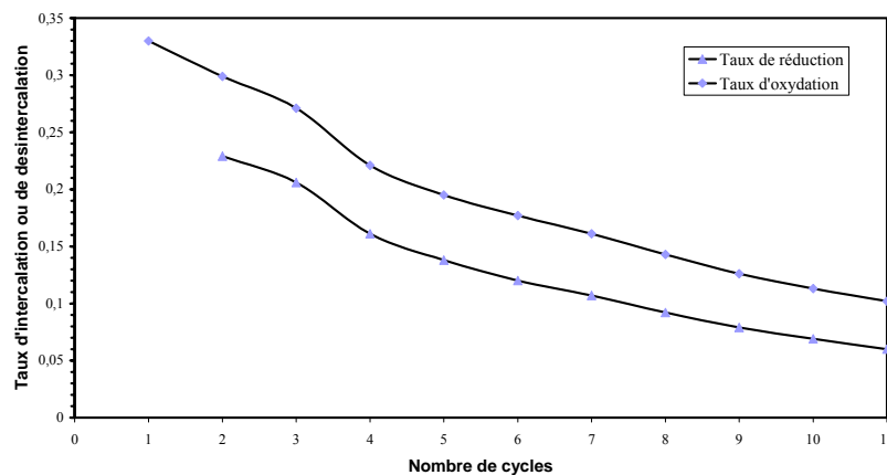
Figure III.16 : Evolution des taux d'intercalation ou de désintercalation en fonction de nombre de cycles.
