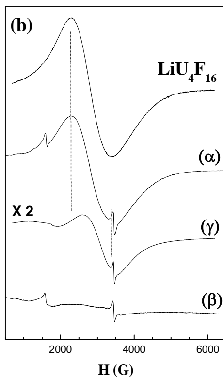
Figure II.24 : (a) Voltampérométrie de \text{LiU}_4\text{F}_{16} et (b) spectres RPE de \text{LiU}_4\text{F}_{16} , \text{LiU}_4\text{F}_{16} réduit ( \alpha ), \text{LiU}_4\text{F}_{16} oxydé à 3,72 V ( \gamma ) et à 4,4 V ( \beta ).
