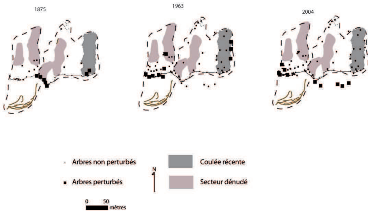
Figure 82. Les emprises spatiales des phases de réactivation du glissement de terrain du Bois Noir.
