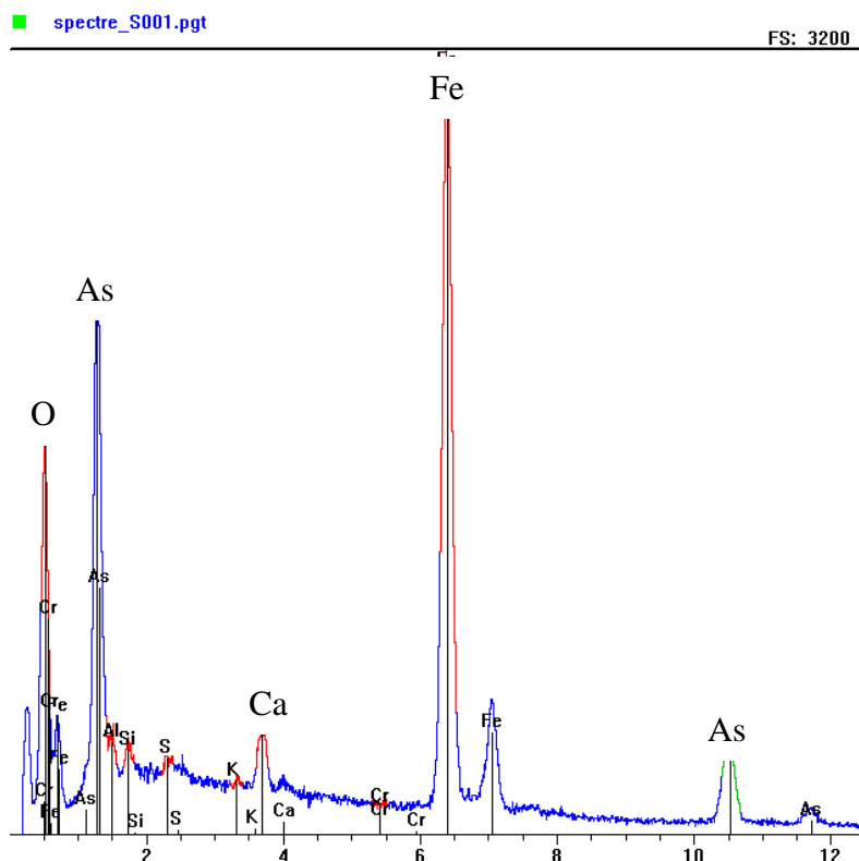
Figure 17 : spectre EDS obtenu par l'analyse ponctuelle (3 points) au niveau de la sous-zone II.
