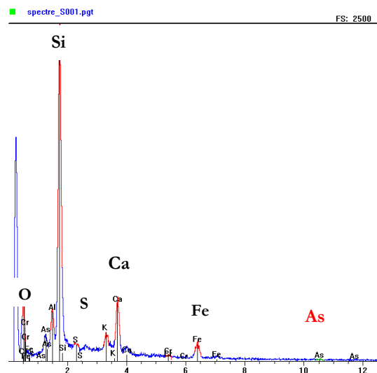
Figure 12 : spectre EDS de la poudre de sol
