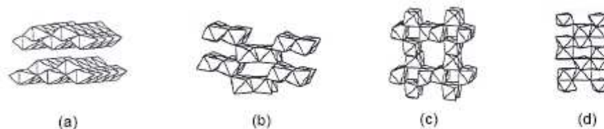
Figure 4 : les principales formes minérales des oxy(hydroxydes) et oxydes de fer (III). (a) lépidocrocite ( \gamma\text{FeOOH} ) ; (b) goethite ( \alpha\text{FeOOH} ) ; (c) akaganeite ( \beta\text{FeOOH} ) ; (d) hématite ( \alpha\text{Fe}_2\text{O}_3 ) d'après Manceau et Drits (1993)
