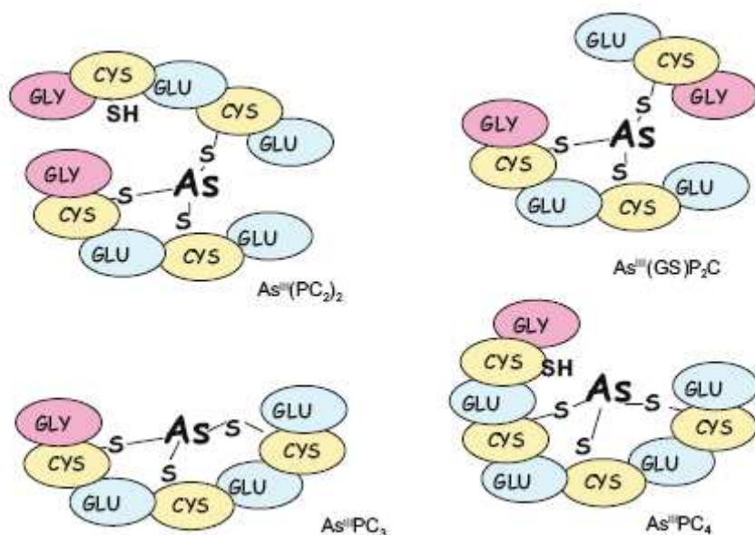
Fig. 7 Structures des complexes arsénites-phytochélatines. Il existe deux isoformes pour As^{III}(PC_2)_2 par contre il existe quatre pour As^{III}PC_4 . GLU, (glutamic acid); CYS, (cystéine); GLY, (glycine)
