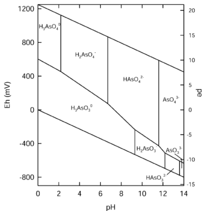
Figure 3 : diagramme Eh-pH pour les espèces aqueuses d'As du système As-O_2-H_2O à 25°C et une pression totale de 1 bar d'après Smedley et Kinniburgh (2002).
