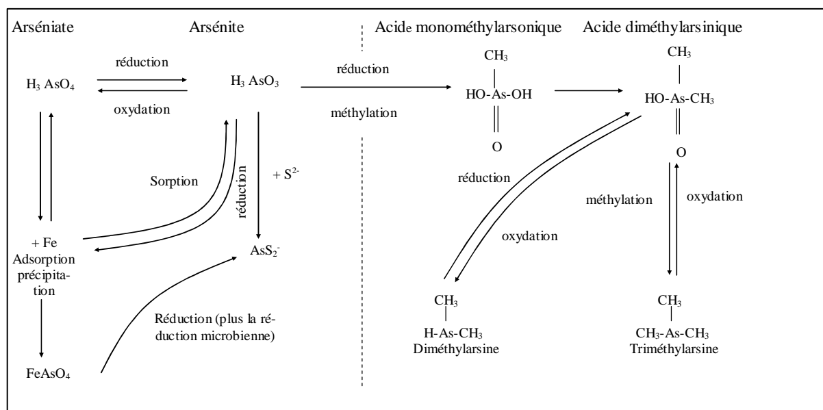
Figure 2 : les processus géochimiques de transformation des espèces arsénées dans les sols d'après Yamauchi et Yamamura (1983) et Adriano et al. (2001).
