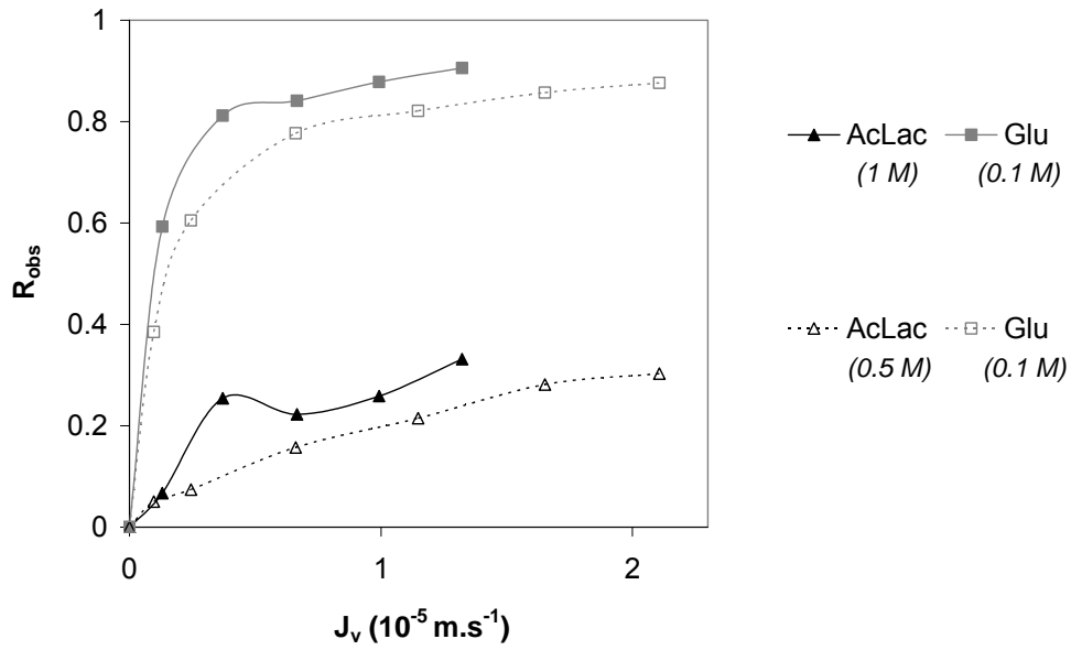
Figure IV-20 . Mélange glucose / acide lactique - Rétentions observées - v_t = 1.3 \text{ m}\cdot\text{s}^{-1} - Membrane DK15
