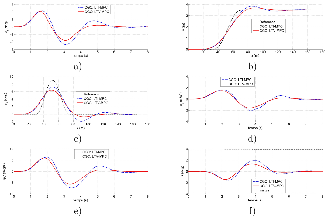
Figure 5.1: Comparaison LTI-MPC et LTV-MPC, changement de file à vitesse de 20 m/s : a) braquage avant ; b) trajectoire du véhicule x - y ; c) trajectoire du véhicule x - \psi_z ; d) accélération latérale ; e) vitesse de lacet ; f) angle de dérive du véhicule
