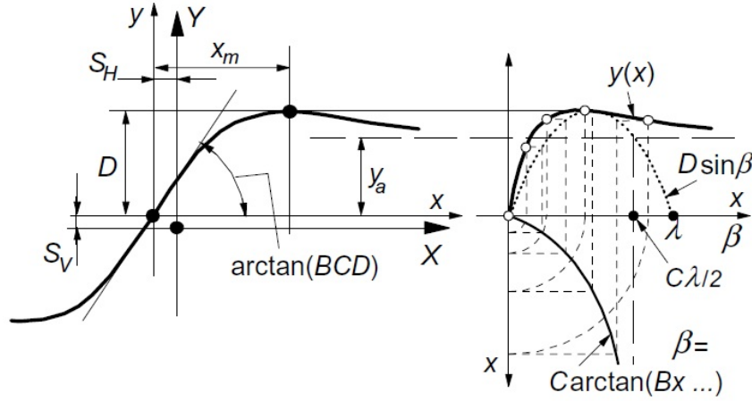
Figure 2.10: Courbe produite par le modèle "Magic Formula" de Pacejka [PAC 06]
