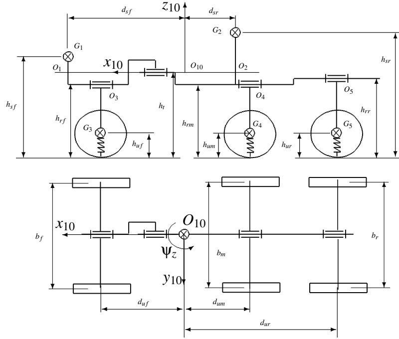
Figure 2.7: Paramétrage du modèle
