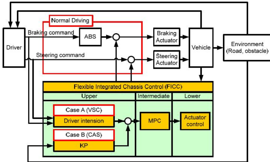
Figure 1.19: Structure de commande centralisée par commande prédictive [CHA 07]
