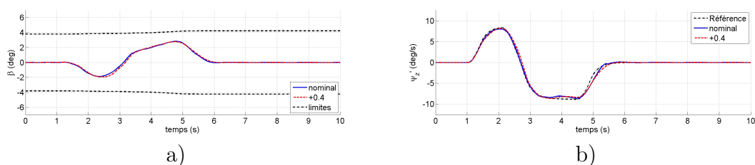
Figure 4.8: Etude de robustesse du contrôleur (CGC, allocation de contrôle) par rapport à la variation du coefficient d'adhérence : a) angle de dérive du véhicule ; b) vitesse de lacet
