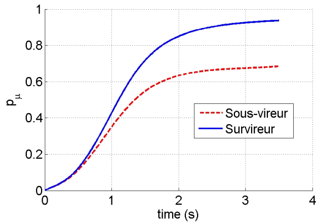
Figure 3.14: Potentiel d'adhérence comme réponse à une "rampe" de l'angle volant
