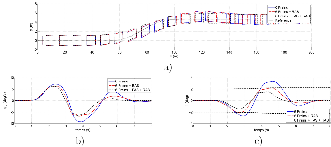
Figure 5.9: Résultats de simulation pour la manœuvre de type "changement de file" avec la vitesse initiale de 25 m/s, le déplacement selon y est de 4.7 m, \mu = 0.35 : a) trajectoire du véhicule ; b) vitesse de lacet ; c) angle de dérive
