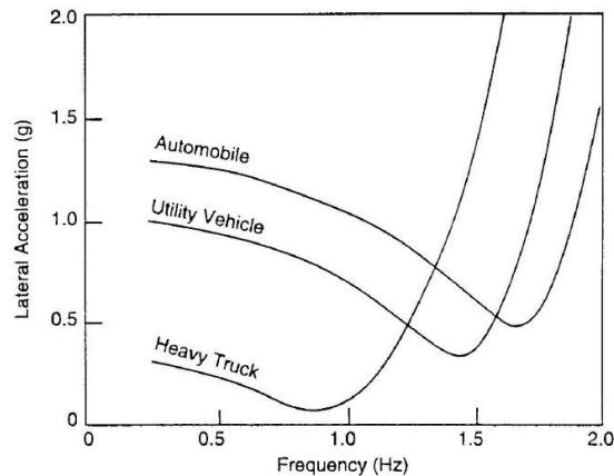
Figure 3.5: Le seuil du renversement en fonction de la fréquence de braquage des roues avant du véhicule [BER 89]
