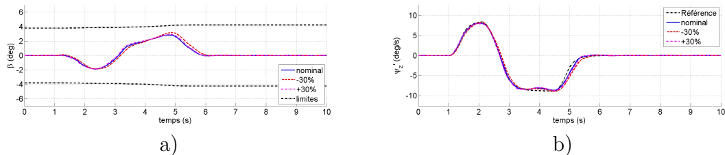
Figure 4.6: Etude de robustesse du contrôleur (CGC, allocation de contrôle) par rapport à la variation du moment d'inertie en lacet du véhicule : a) angle de dérive du véhicule ; b) vitesse de lacet
