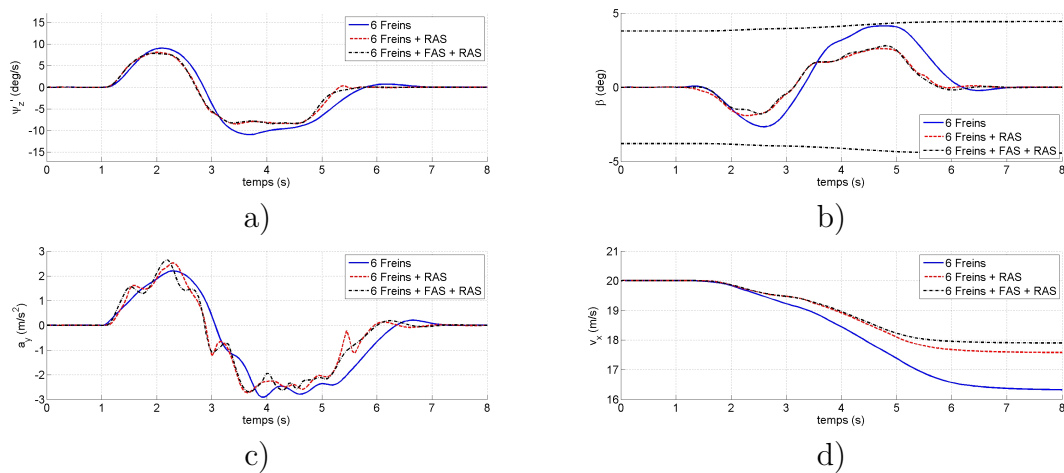
Figure 5.4: Résultats de simulation pour la manœuvre de type "sine with dwell" (amplitude commande braquage avant = 0.06 rad) avec la vitesse initiale de 20 m/s : a) vitesse de lacet ; b) angle de dérive ; c) accélération latérale ; d) vitesse longitudinal
