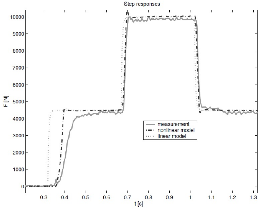
Figure 2.14: La réponse des modèles non-linéaire et linéaire de l'actionneur EMB à une série de signaux de type "step" [PET 03]
