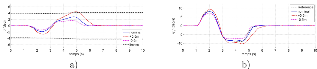
Figure 4.7: Etude de robustesse du contrôleur (CGC, allocation de contrôle) par rapport à la variation de la position longitudinale du centre de gravité du véhicule : a) angle de dérive du véhicule ; b) vitesse de lacet
