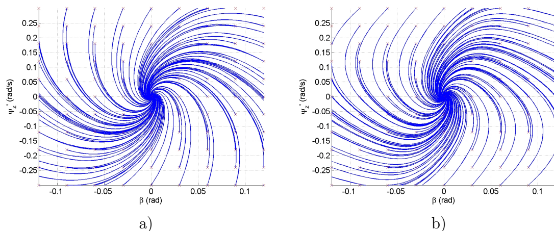
Figure 3.10: Plan de phase d'un véhicule sous-vireur à vitesse v_x = 20 m/s et angle au volant \delta_{swa} = 0 , \times sont les conditions initiales : a) \mu = 0.75 ; b) \mu = 0.3
