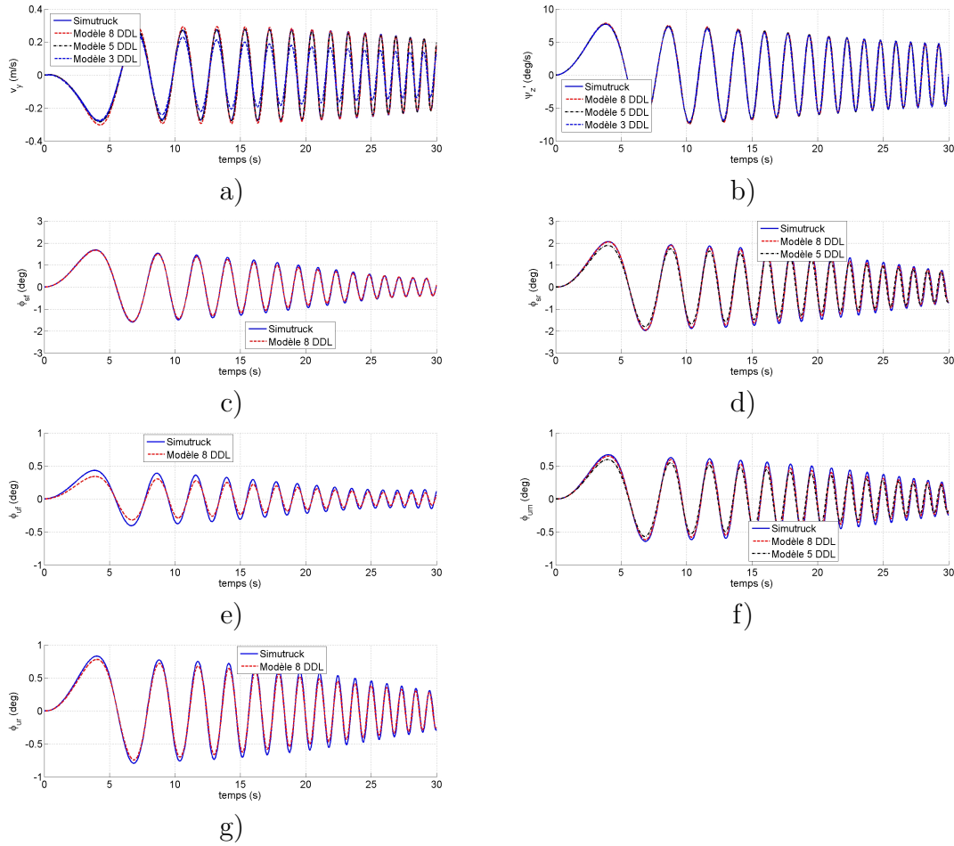
Figure 2.9: Validation de modèles, manœuvre "Sinus balayé" : a) vitesse latérale ; b) vitesse de lacet ; c) angle de roulis de la partie avant du châssis ; d) angle de roulis de la partie arrière du châssis ; e) angle de roulis de l'essieu avant ; f) angle de roulis de l'essieu milieu ; g) angle de roulis de l'essieu arrière.
