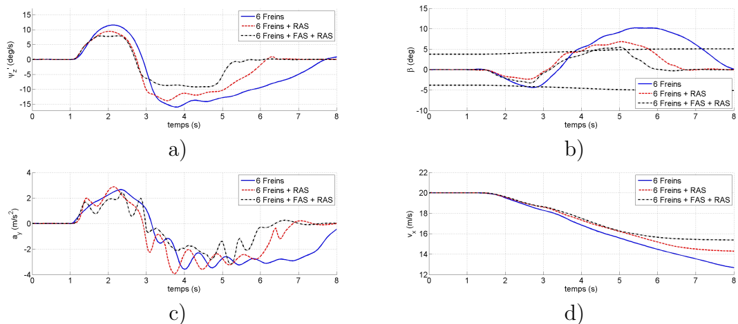
Figure 5.6: Résultats de simulation pour la manœuvre de type "sine with dwell" (amplitude commande braquage avant = 0.1 rad) avec la vitesse initiale de 20 m/s : a) vitesse de lacet ; b) angle de dérive ; c) accélération latérale ; d) vitesse longitudinale
