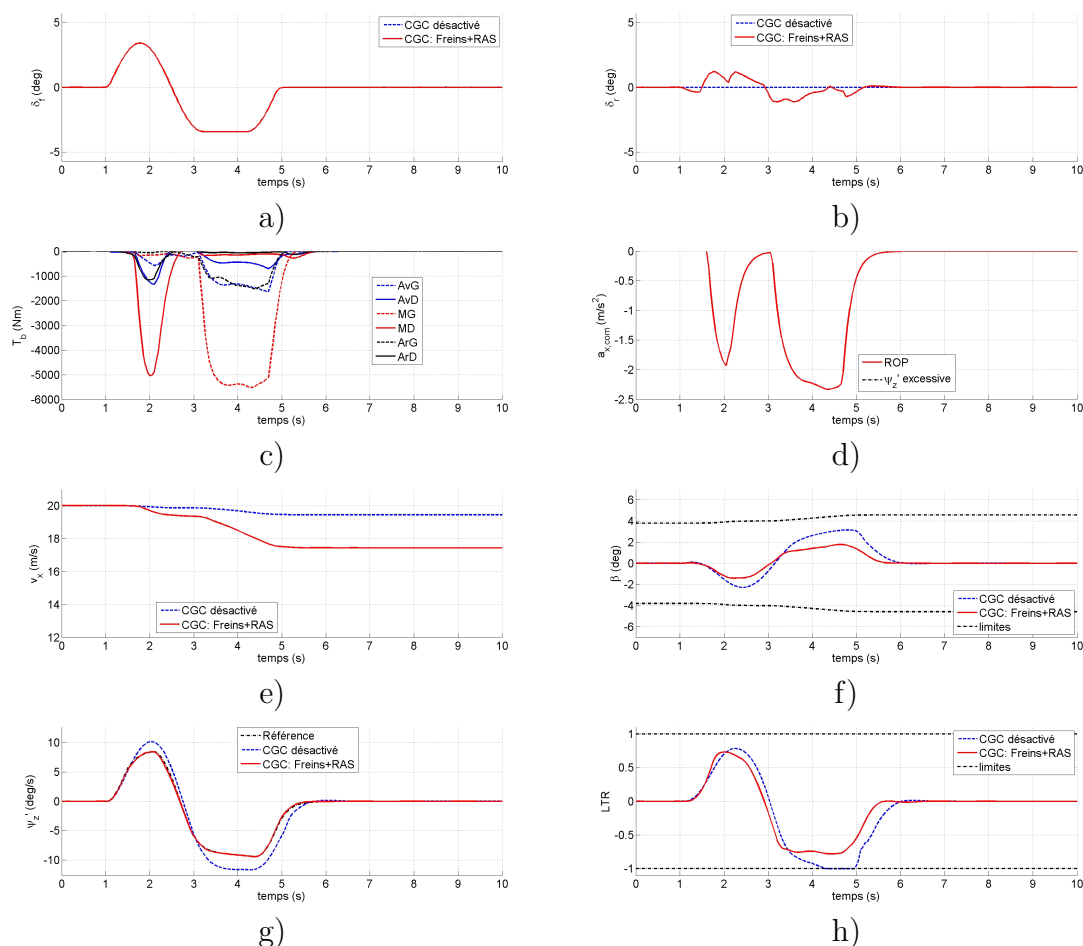
Figure 4.4: Résultats de simulation pour la manœuvre "Sine with dwell" sur forte adhérence pour le véhicule avec CGC basé sur la structure de commande avec l'allocation de contrôle (activé et désactivé) : a) angle de braquage des roues de l'essieu avant ; b) angle de braquage des roues de l'essieu arrière ; c) couple de freinage ; d) commande de l'accélération longitudinale ; e) vitesse longitudinale ; f) angle de dérive du véhicule ; g) vitesse de lacet ; h) LTR_{mr}
