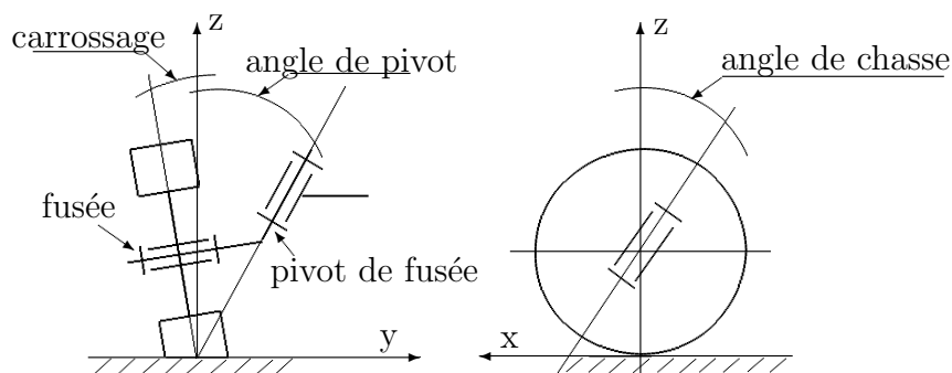
Figure 2.5: Angle de pivot, angle de chasse, angle carrossage
