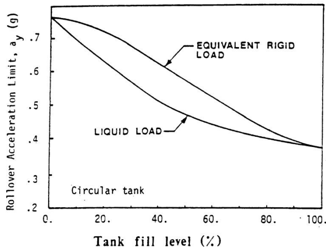
Figure 3.4: Comparaison des seuils de renversement entre un camion-citerne (citerne avec une section circulaire) et un véhicule avec une charge fixée de manière rigide [RAN 89b]
