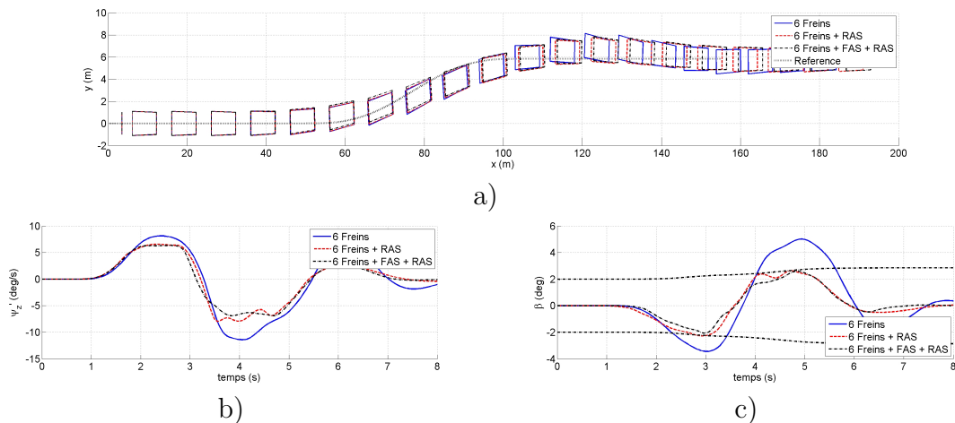
Figure 5.10: Résultats de simulation pour la manœuvre de type "changement de file" avec la vitesse initiale de 25 m/s, le déplacement selon y est de 5.8 m, \mu = 0.35 : a) trajectoire du véhicule ; b) vitesse de lacet ; c) angle de dérive
