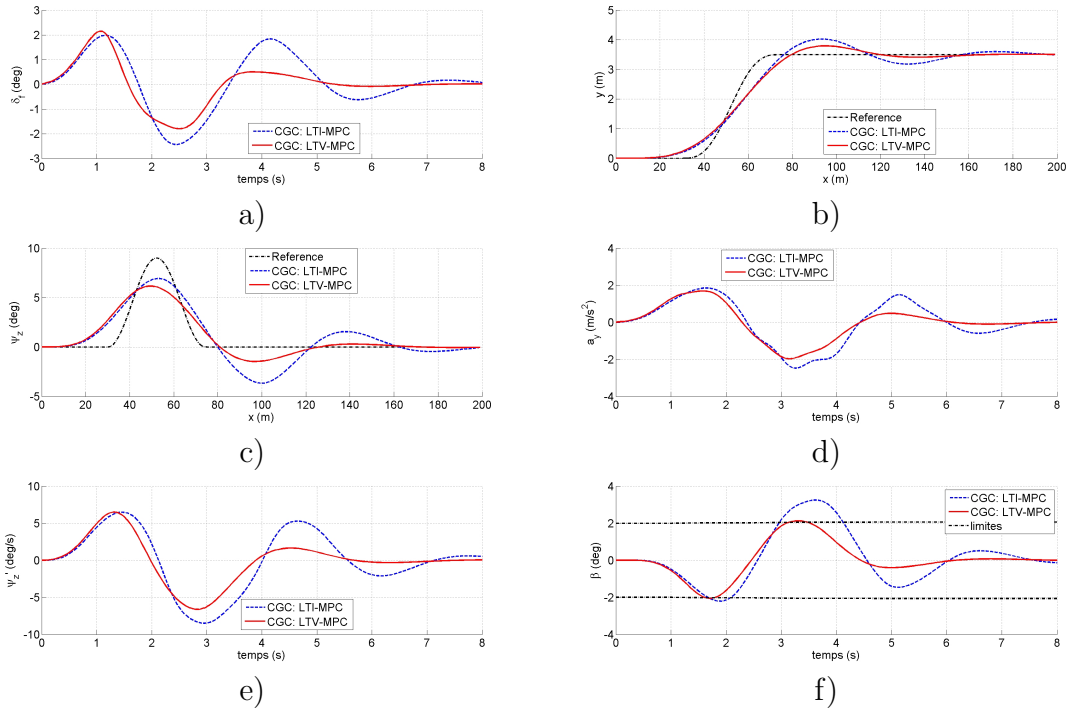
Figure 5.2: Comparaison LTI-MPC et LTV-MPC, changement de file à vitesse de 25 m/s : a) braquage avant ; b) trajectoire du véhicule x - y ; c) trajectoire du véhicule x - \psi_z ; d) accélération latérale ; e) vitesse de lacet ; f) angle de dérive du véhicule
