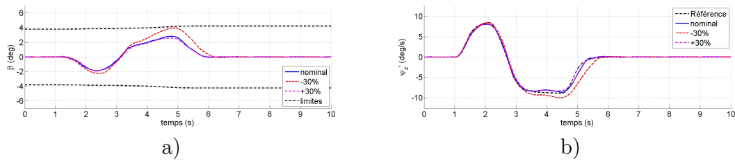
Figure 4.5: Etude de robustesse du contrôleur (CGC, allocation de contrôle) par rapport à la variation de la masse totale du véhicule : a) angle de dérive du véhicule ; b) vitesse de lacet
