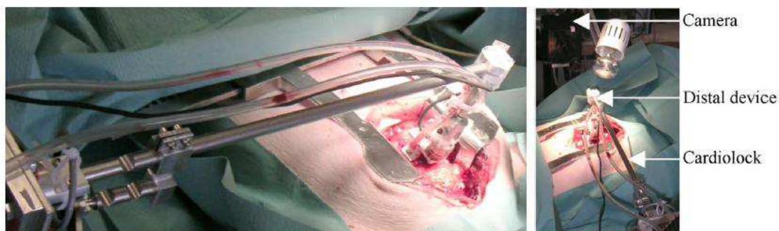
FIG. 1.12 – Le système Cardiolock [Bachta 2008] est positionné sur le cœur d'un cochon pour une compensation active des battements cardiaques.
