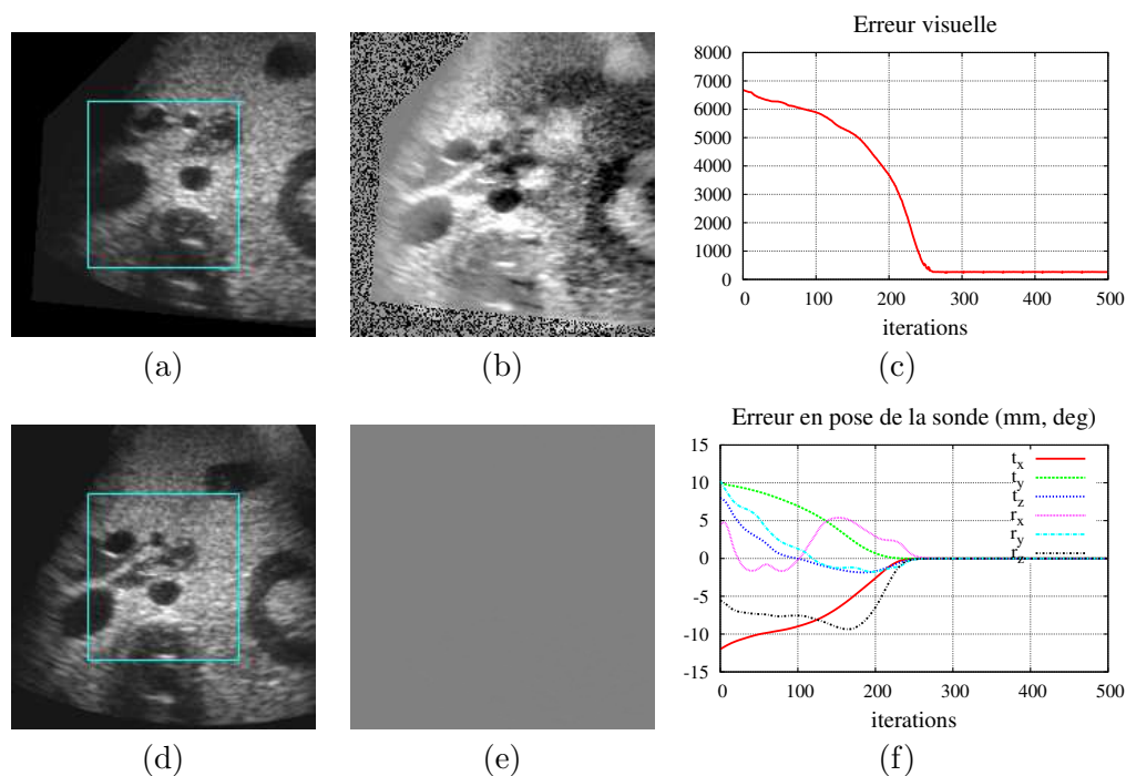
FIG. 4.13 – Simulation de positionnement avec une sonde 3D. Vues initiale (a) et finale (d) de la sonde avec les images de différence associées (b,e). Évolution de l'erreur d'image (c) et de pose (f) au cours de l'asservissement.
