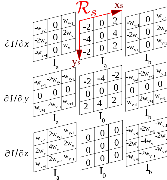
FIG. 4.6 – Modèle du filtre gradient 3D pondéré pour tenir compte de l'orientation entre les images considérées.
