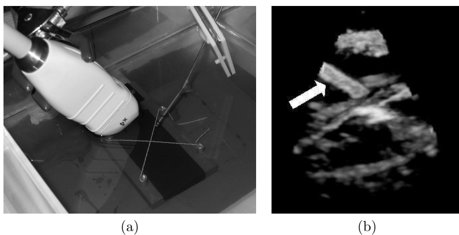
FIG. 2.13 – Positionnement d'un outil sur une cible par asservissement visuel [Novotny 2007]. (a) Environnement expérimental. (b) Détection de l'outil dans l'image échographique.
