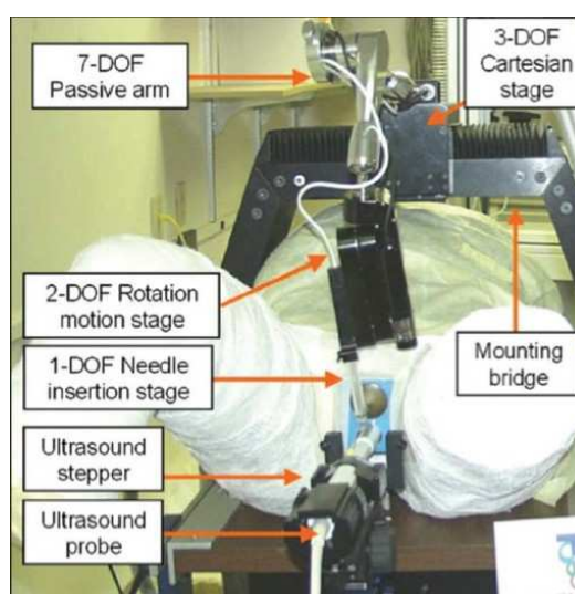
FIG. 1.9 – Un système robotique d'insertion d'aiguille développé pour réaliser une biopsie de la prostate [Fichtinger 2002].
