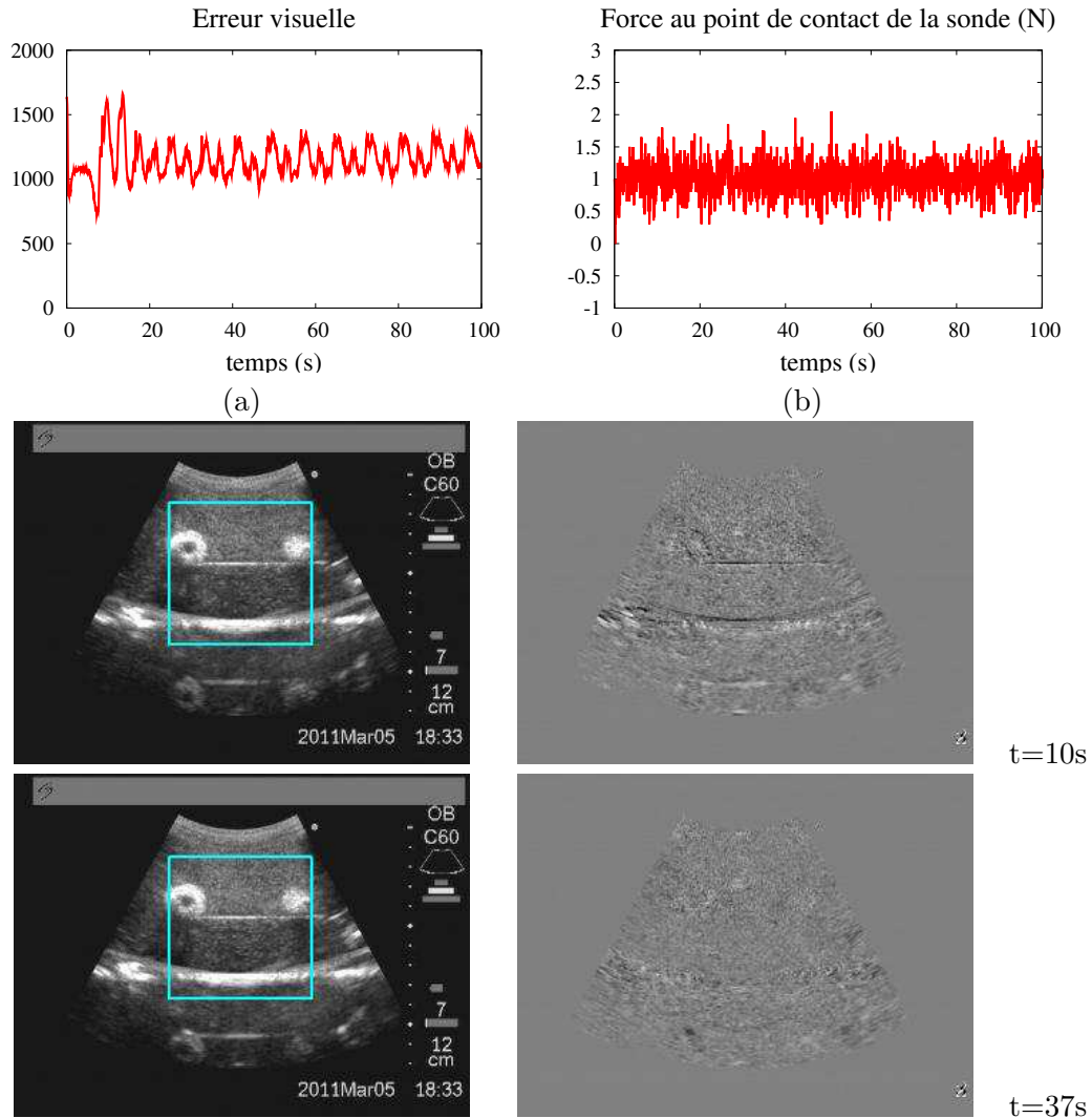
FIG. 5.16 – Suivi d'une coupe du fantôme en gélatine, contenant deux olives.
