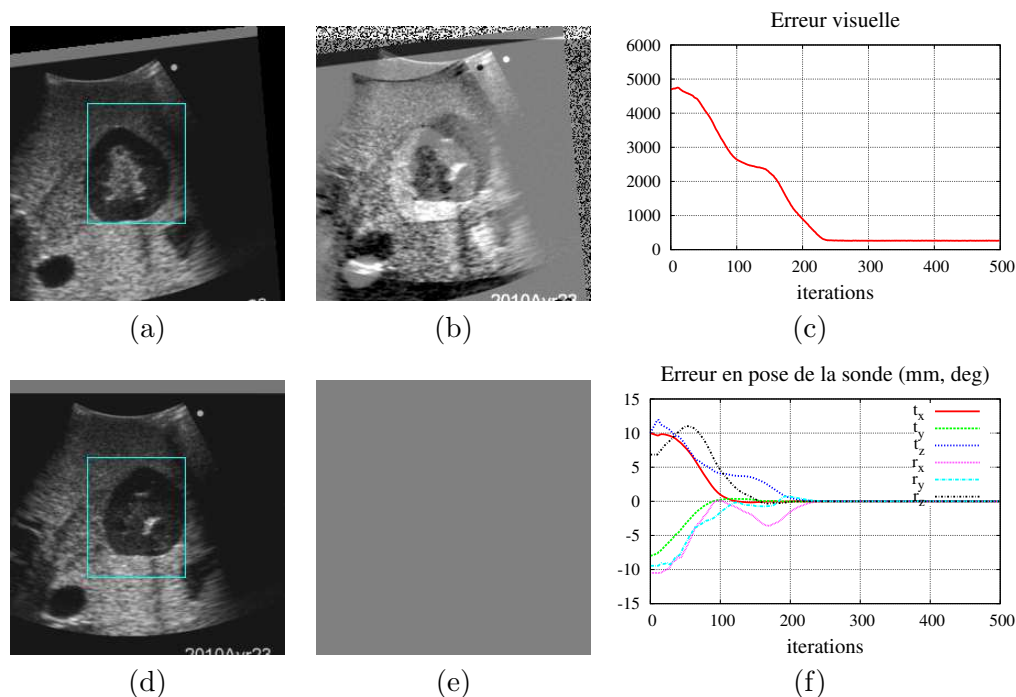
FIG. 4.12 – Tâche de positionnement avec la sonde 2D en présence de bruit de mesures. Les images (a) et (d) représentent les vues initiale et finale de la sonde. Les images de différence associées (b) et (e) permettent de visualiser le succès de la tâche de positionnement. Enfin les courbes (c) et (f) correspondent à l'évolution de l'erreur visuelle et à l'erreur en pose au cours de l'asservissement visuel.
