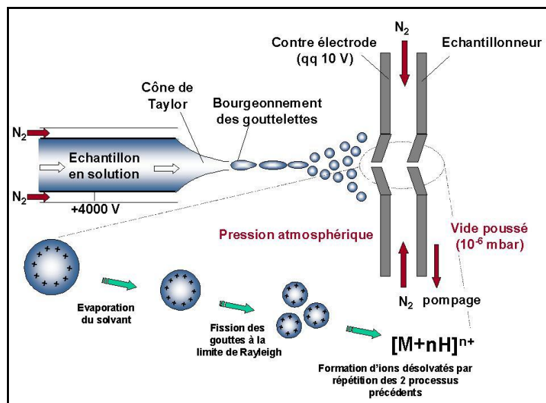
Figure 14 : Schéma d'une source électrospray
