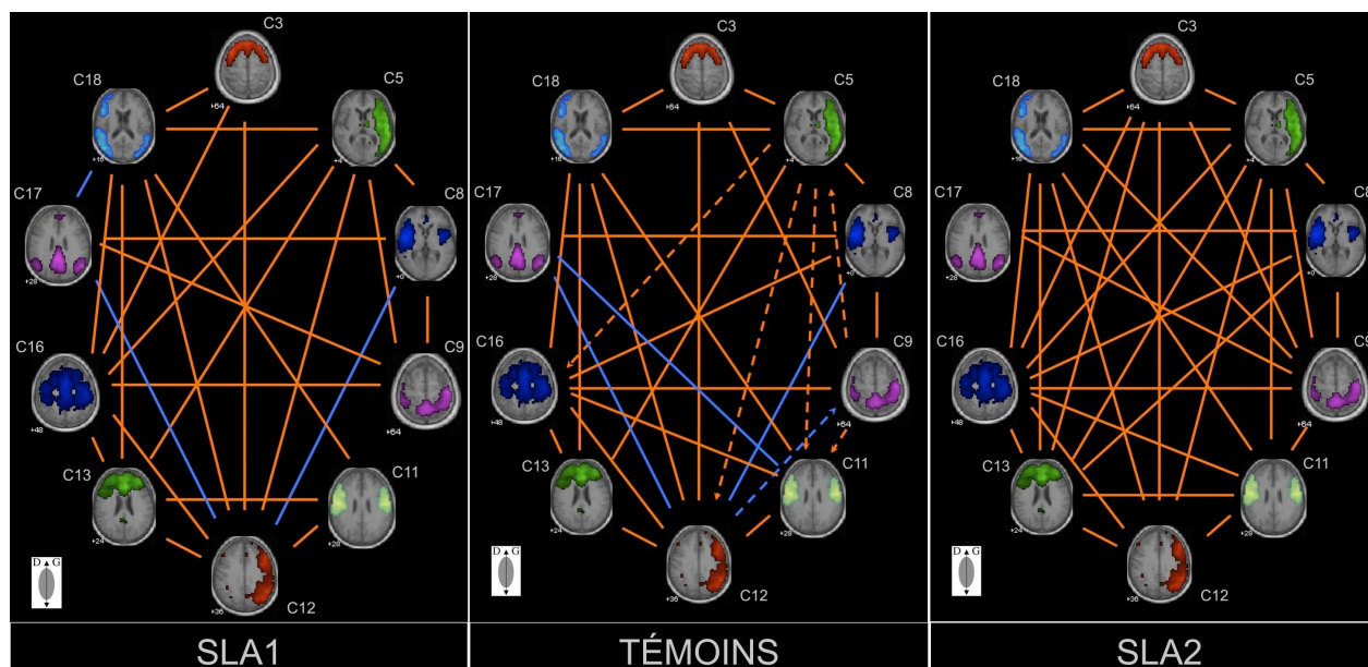
Figure 21 : ensemble des corrélations entre les composants dans les groupes SLA1, Témoins et SLA2. Trait orange: corrélation positive. Trait bleu : corrélation négative (anti-corrélation). Trait pointillé : décalage temporel
