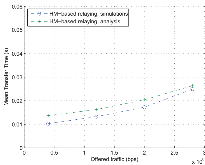
FIGURE 5.2 – Temps moyen de transfert global
