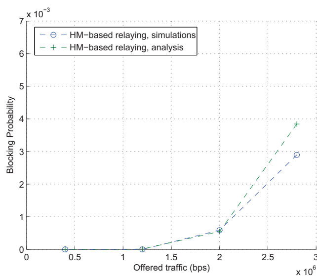
FIGURE 5.3 – Probabilité de blocage
