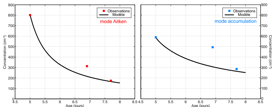
FIGURE 4.21 – Evolution en fonction du temps de la concentration des modes Aitken (à gauche) et d'accumulation (à droite), observés et simulés en ne prenant en compte que la coagulation.
