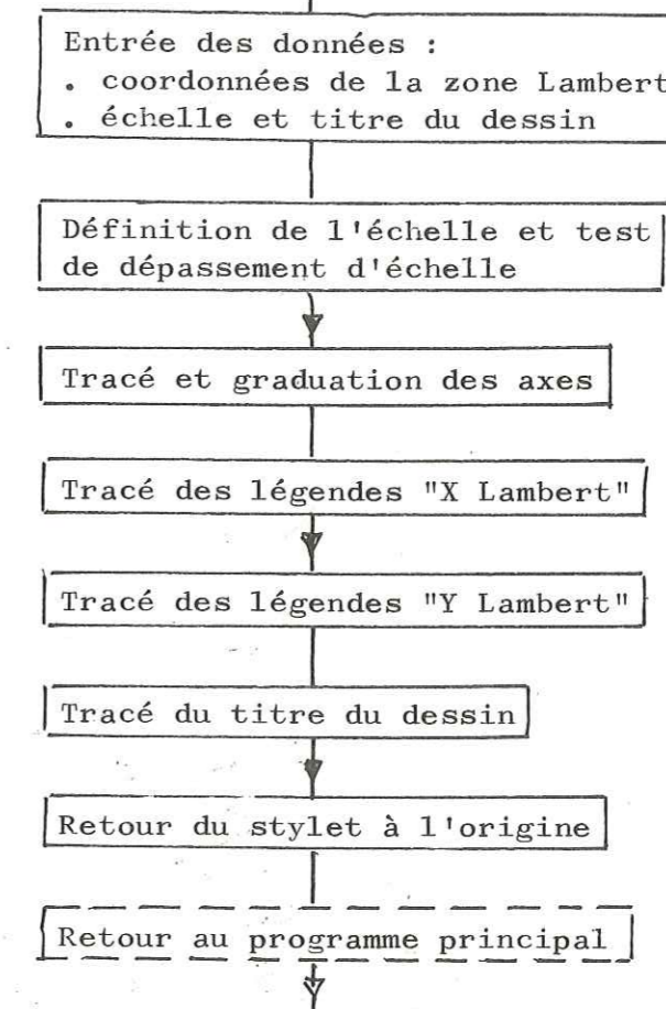
Figure 26 : Fonctionnement général du sous-programme DRAW1
