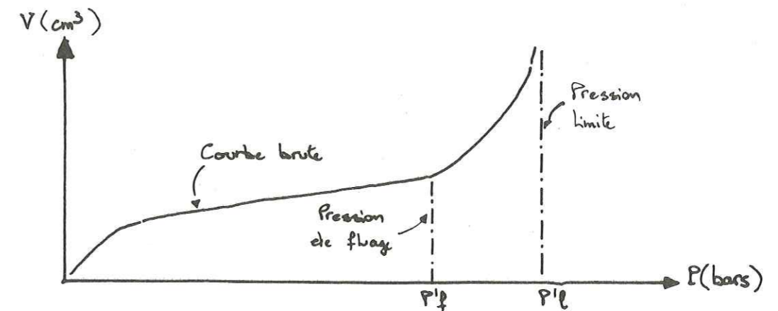
Figure 2 : Courbe pressiométrique (variations du volume de la cellule pressiométrique en fonction de la pression appliquée après une minute).
