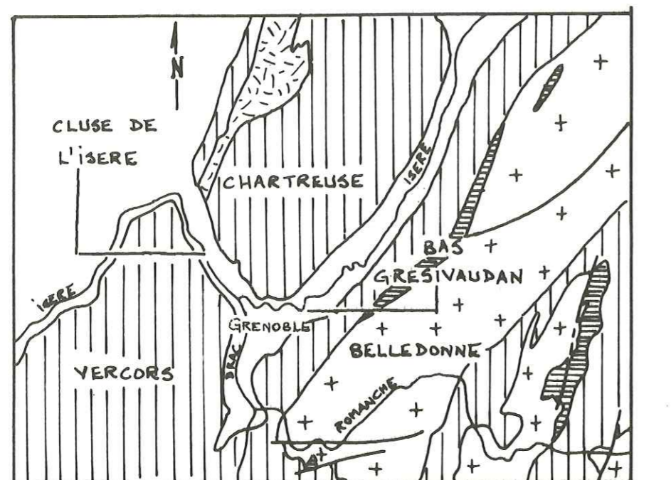
FIGURE 33 , CADRE GÉOGRAPHIQUE ET GÉOLOGIQUE RÉGIONAL.
