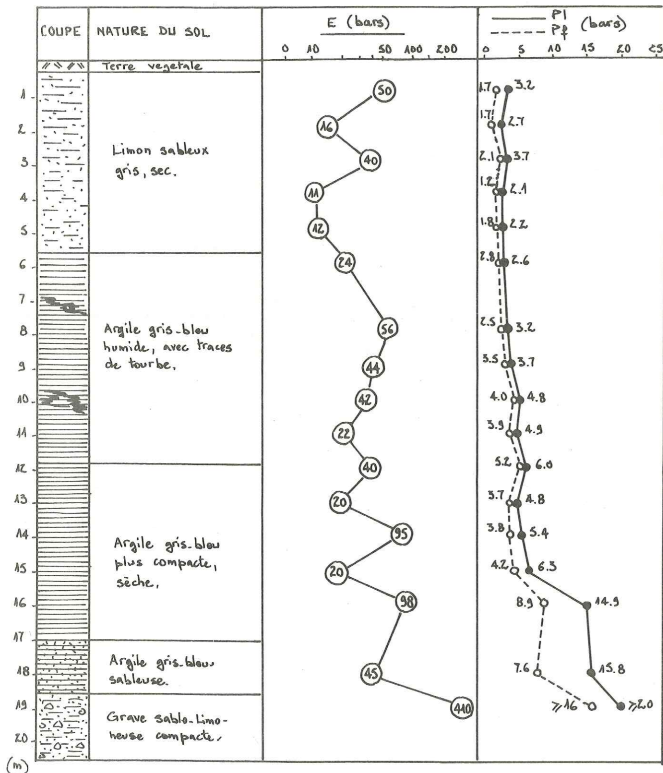
FIGURE 11. PRESENTATION DES RESULTATS D'UN SONDAGE PRESSIOMETRIQUE,
