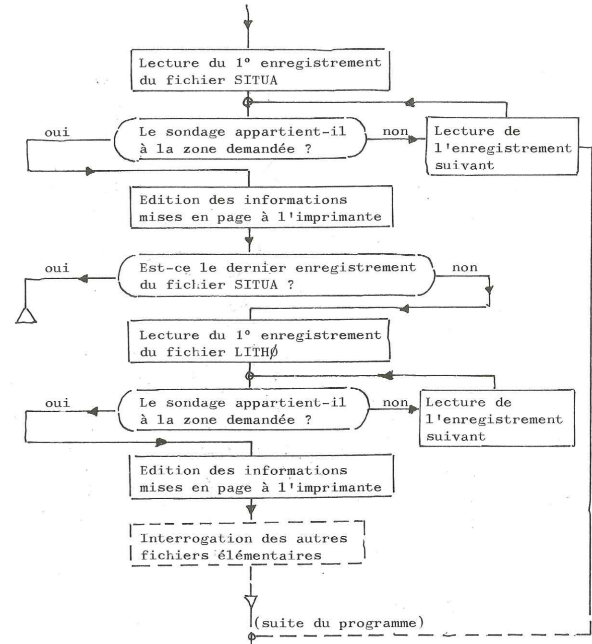
Figure 23 : Fonctionnement général du programme EDITN (interrogation des fichiers SITUA et LITHØ)
