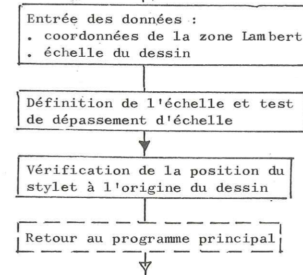
Figure 27 : Fonctionnement général du sous-programme DRAW3
