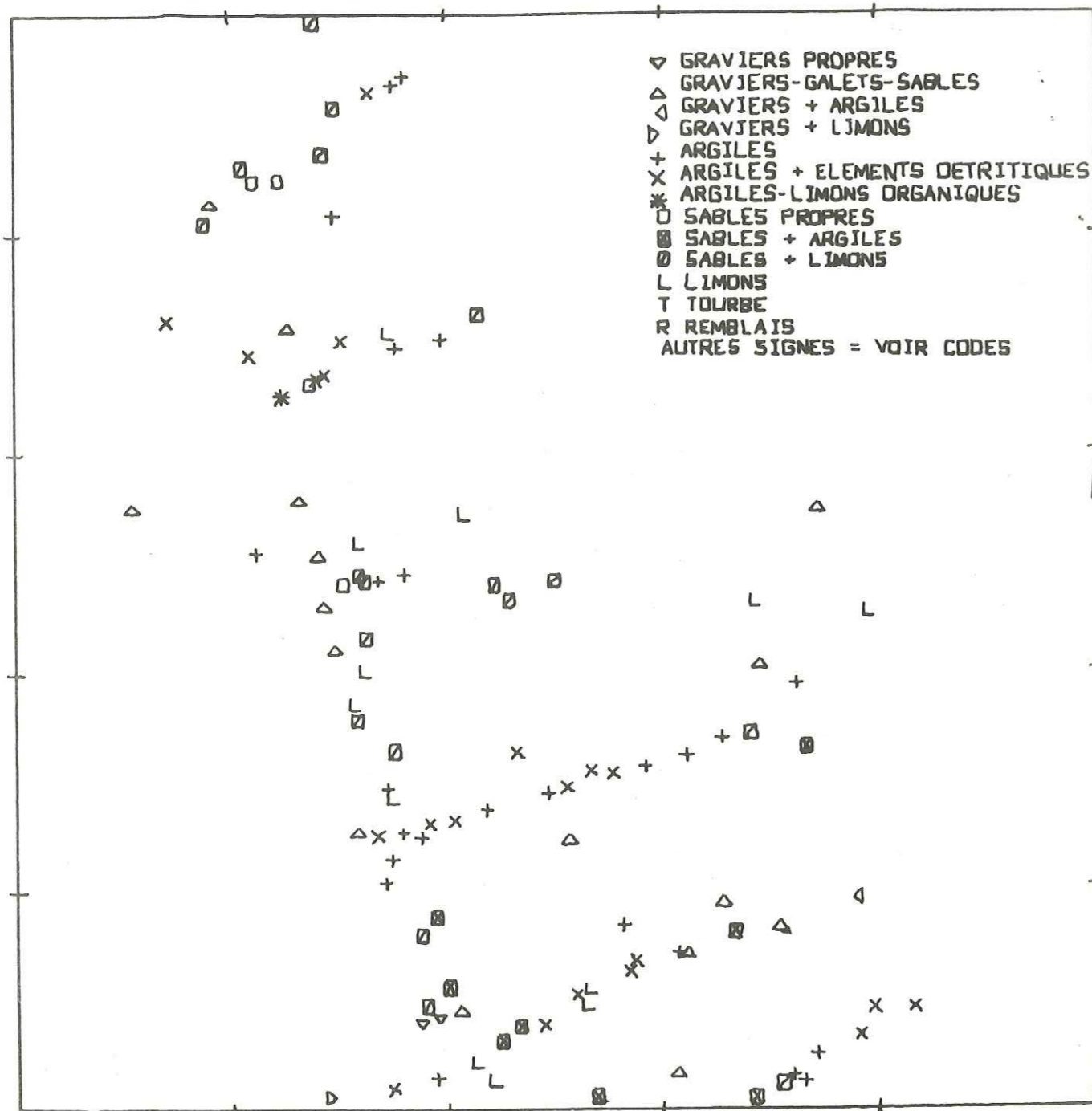
Figure 30 : Exemple d'édition graphique réalisée par le programme GEOL : nature du sous-sol sous la terre végétale aux environs de Voreppe entre les coordonnées Lambert : X = 856. - 861. (Km) Y = 335. - 340. Echelle 1/25 000
