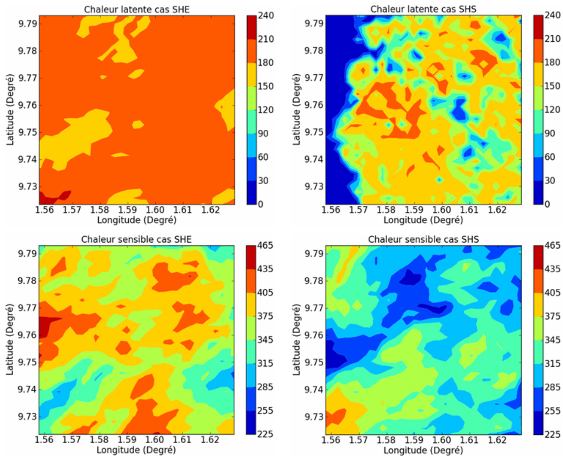
FIGURE 5.12 – Chaleur sensible E ( W.m^{-2} ) et sensible H ( W.m^{-2} ) en cas humide.
