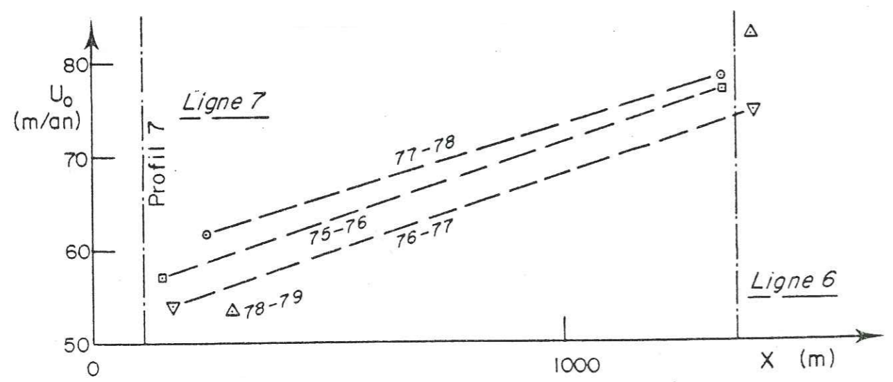
FIG. 18 : Vitesses moyennes (lignes 1-2 et 5) ou centrales (lignes 6 et 7) suivant l'axe longitudinal du glacier
