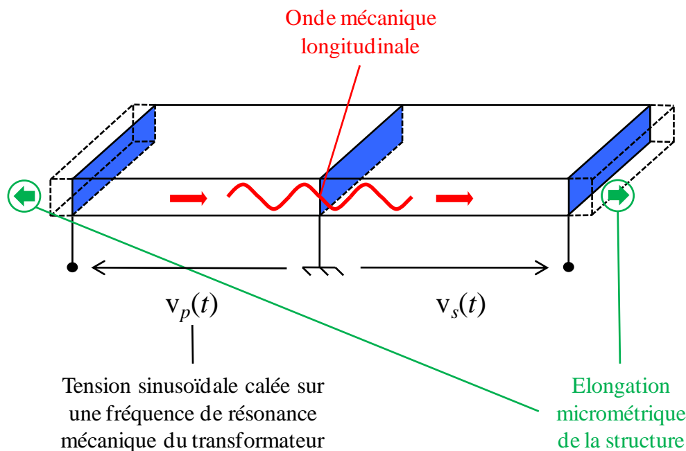
FIGURE 1.8 – Principe de fonctionnement d'un transformateur piézoélectrique
