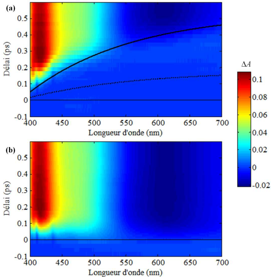
Figure 29 : Prétraitement de donnée spectrocinétiques acquises sur le SA dans l'acétonitrile et excité à 384 nm. (a) Données brutes, les retards \tau_{BK7}(\lambda) sont représentés en trait discontinu et les retards \tau_{GVD}(\lambda) en trait plein épais, (b) données prétraitées.
