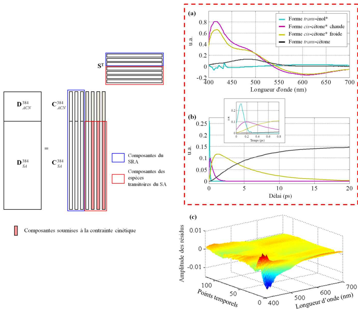
Figure 57 : Résultats de la décomposition par HS-MCR de la réponse spectrocinétique du SA (matrice de données augmentées [ D_{ACN}^{384} ; D_{SA}^{384} ]). (a) Spectres et (b) profils de concentration des composantes spécifiques à la matrice D_{SA}^{384} , (c) résidus D_{SA}^{384} - C_{SA}^{384} \cdot S^T .
