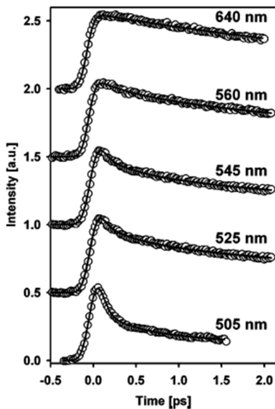
Figure 10 : Étude du SA excité à 385 nm dans l'acétonitrile par le groupe de Peon (profils temporels de fluorescence) [49].
