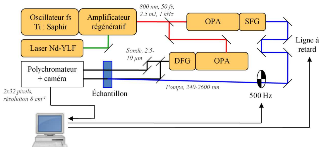
Figure 71 : Schéma de l'installation de spectroscopie d'absorption transitoire femtoseconde IR.
