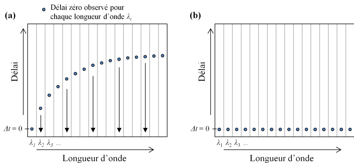
Figure 20 : Illustration du prétraitement numérique de correction de GVD. (a) Données brutes et (b) données prétraitées (algorithme proposé dans la référence [177]).
