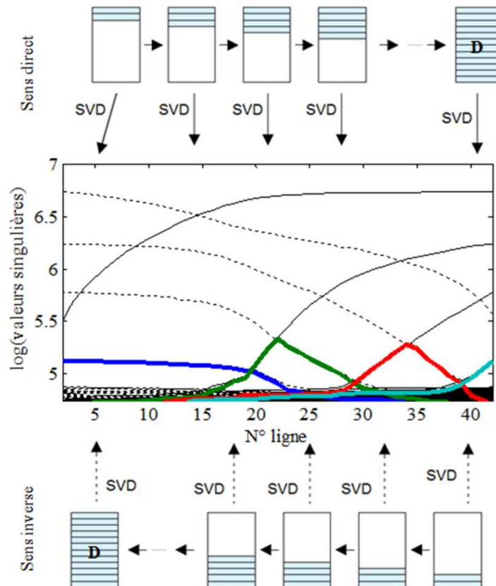
Figure 74 : Principe de l'EFA. Les tracés continus et discontinus désignent l'évolution des valeurs singulières respectivement dans les sens direct et inverse. Les tracés épais et colorés représentent les estimations initiales C_0 de la matrice C .
