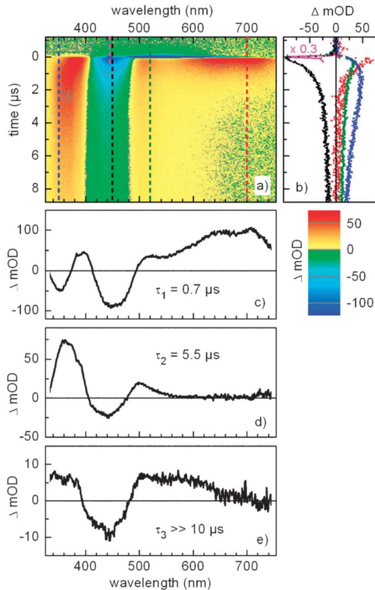
Figure 18 : Exemple de résultats d'analyse globale de déclin d'après [159]. (a) Données spectrocinétiques en représentation bidimensionnelle, (b) variations temporelles d'absorbance pour quelques longueurs d'onde, (c) à (e) DADS associés aux temps caractéristiques.
