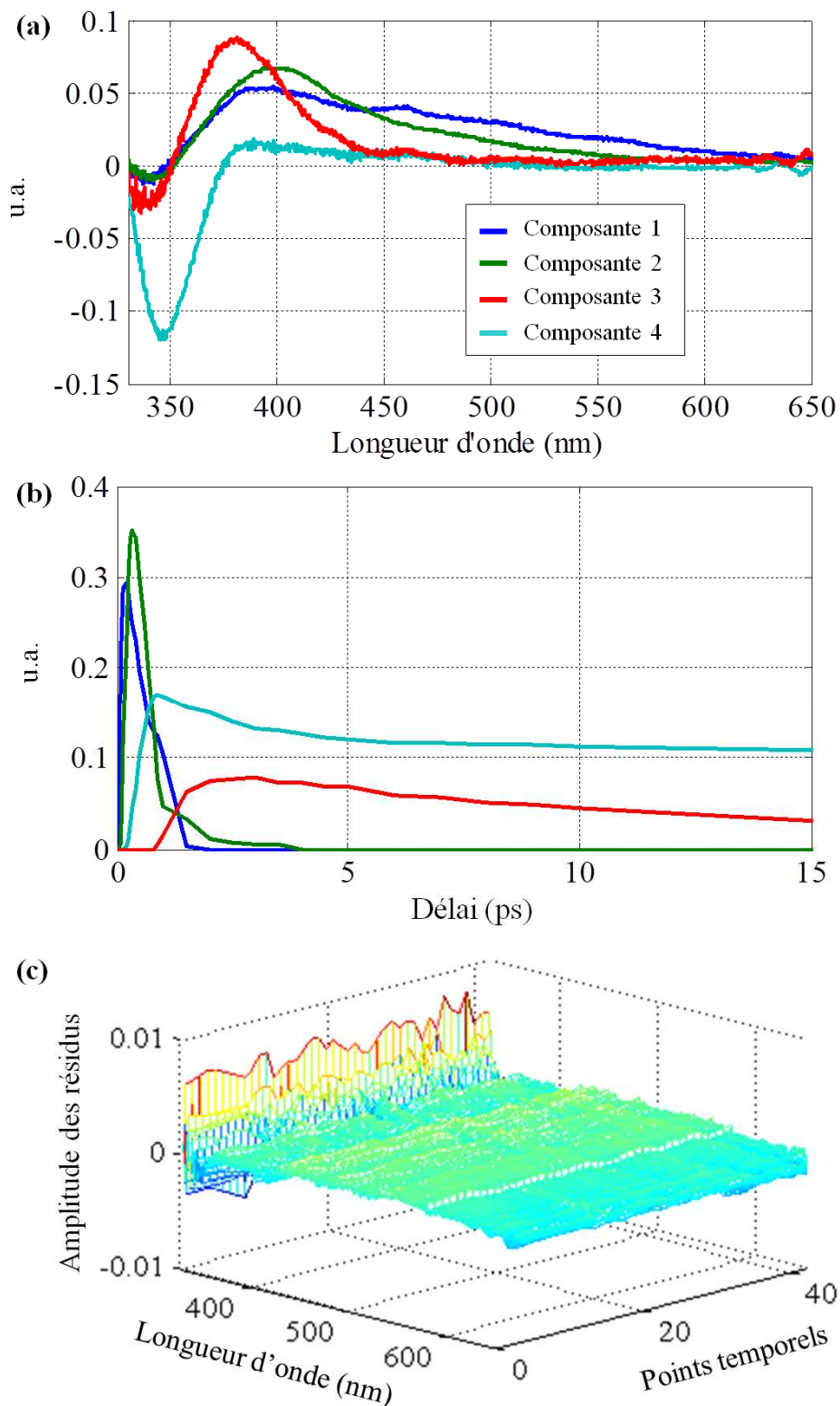
Figure 59 : Résultats de l'analyse exploratoire de réponse spectrocinétique du SAOMe (matrice \mathbf{D}_{SAOMe}^{266} ) par MCR-ALS. (a) Spectres et (b) profils de concentration représentés entre 0 et 15 ps des quatre composantes décrivant ces données, (c) résidus de la modélisation.
