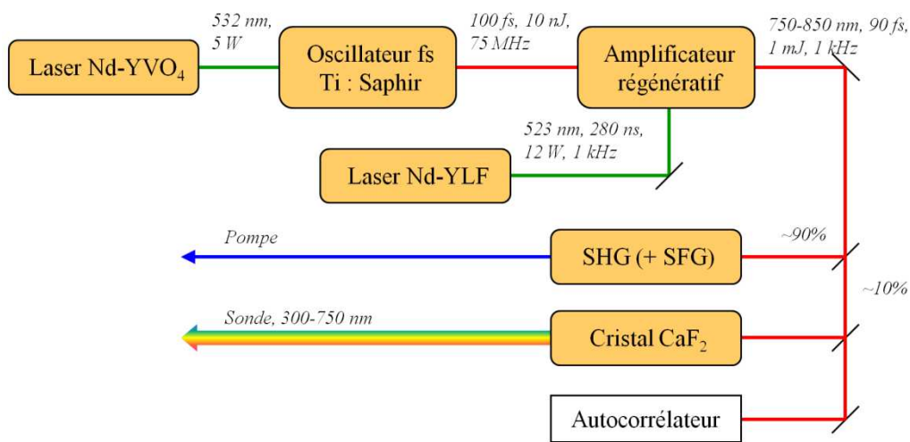
Figure 69 : Génération des faisceaux de pompe et de sonde en spectroscopie d'absorption transitoire femtoseconde UV-visible.
