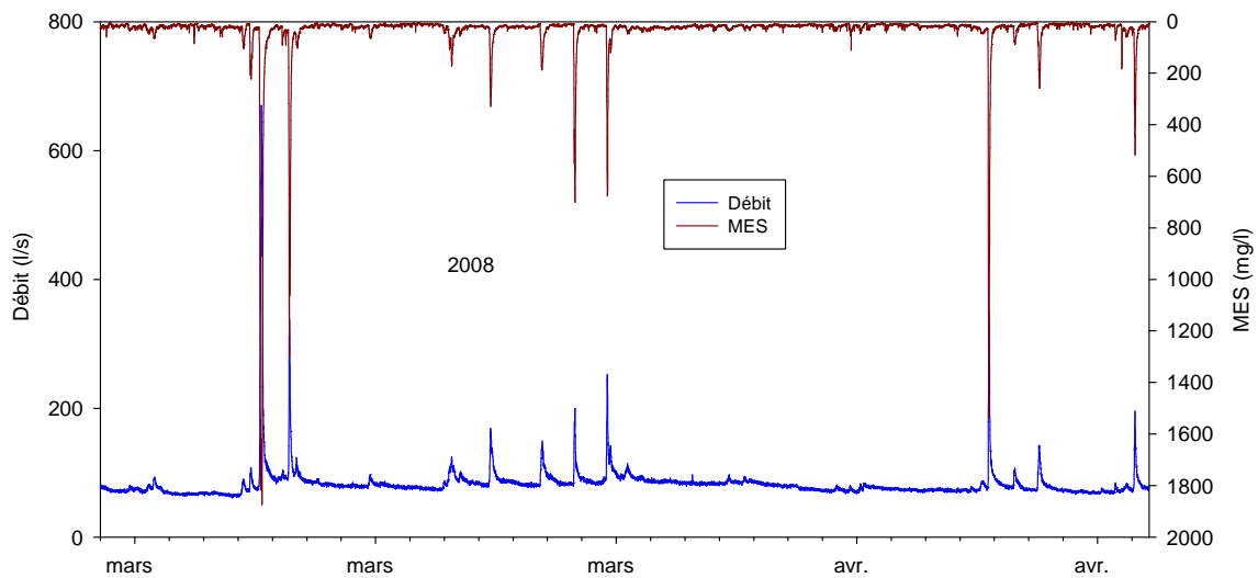
Figure 7.2 : Variabilité temporelle du débit et des concentrations de MES en mars et avril 2008
