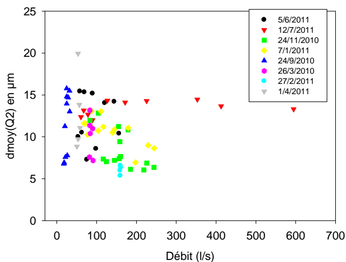
Figure 4.17 : Diamètre moyen, d_{moy}(Q_2) , en fonction du débit
