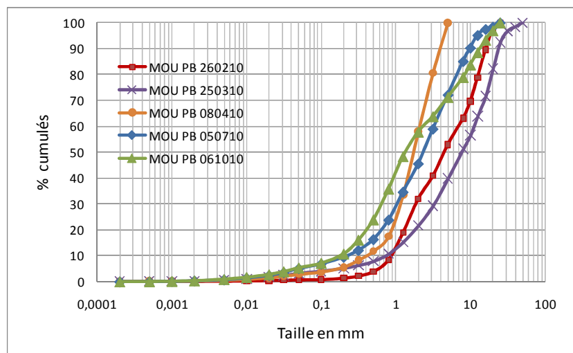
Figure 3.8: Courbes granulométriques cumulatives des échantillons piégés durant des crues (26/02/2010, 25/03/2010, 08/04/2010, 05/07/2010 et 06/10/2010).
