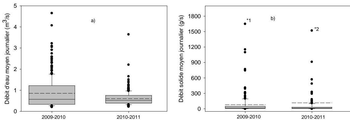
Figure 8.13 : Distribution en box-plots : a) des débits moyens journaliers, et b) des débits solides moyens journaliers pour chaque année hydrologique 2009-2010 et 2010-2011
