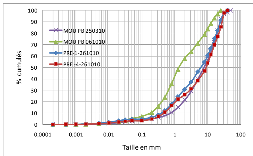
Figure 3.9 : Comparaison des courbes granulométriques des sédiments du Moulinet piégés (25/3/2010, 6/10/2010) et prélevés (26/10/2010).
