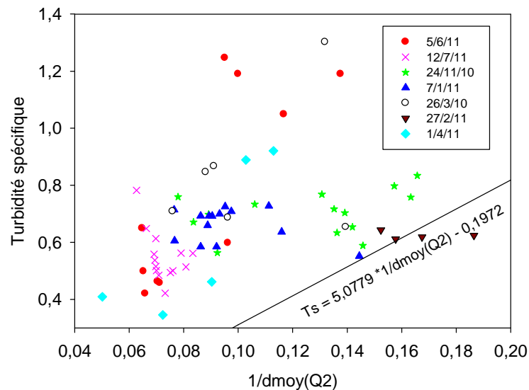
Figure 4.18 : Relation entre la turbidité spécifique et 1/\text{dmoy}(Q2) des MES pour les prélèvements réalisés au cours des crues en 2010 et 2011
