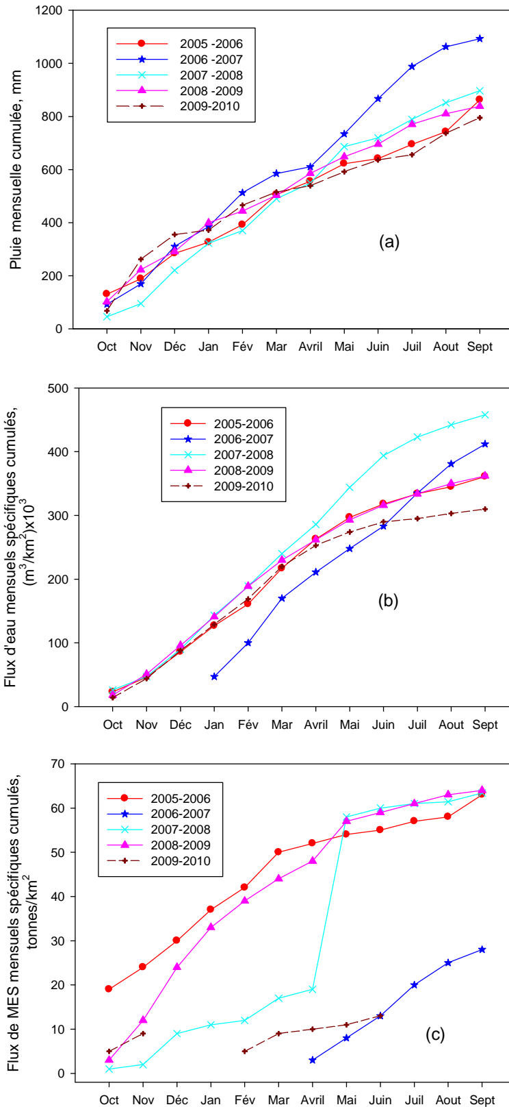
Figure 5.1 : Courbes cumulées de la pluviométrie (a), du flux d'eau (b) et du flux solide (c) mensuels pour chacune des années hydrologiques étudiées
