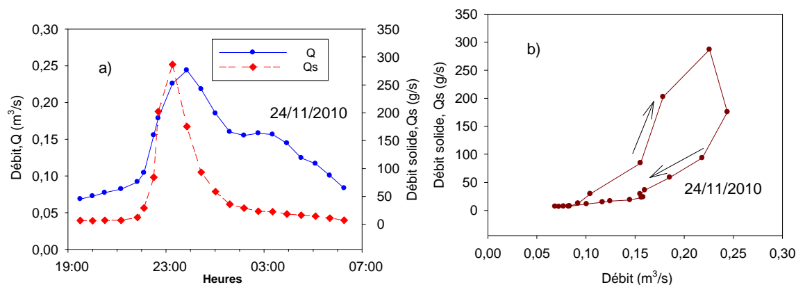
Figure 6.3 : Crue à hystérésis horaire asymétrique : a) variation temporelle du débit d'eau et du débit solide ; b) relation Q_s - Q de la crue du 24 /11/ 2010.
