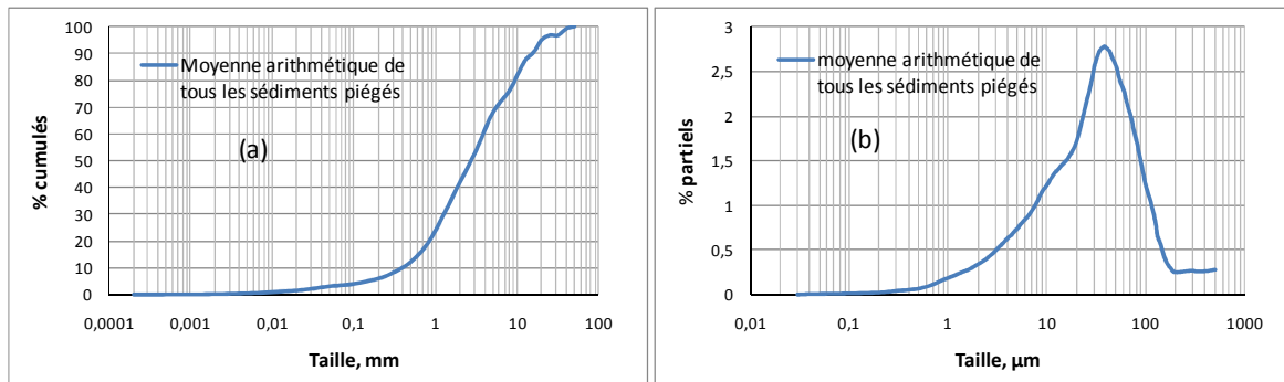
Figure 3.13 : Courbe granulométrique moyenne de tous les sédiments piégés : courbe cumulée (a) ; courbe partielle (b) (< 500 μm).
