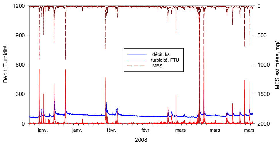
Figure 2.15 : débit et turbidité mesurés, et concentration des MES estimées de janvier à mars 2008 dans le Moulinet.
