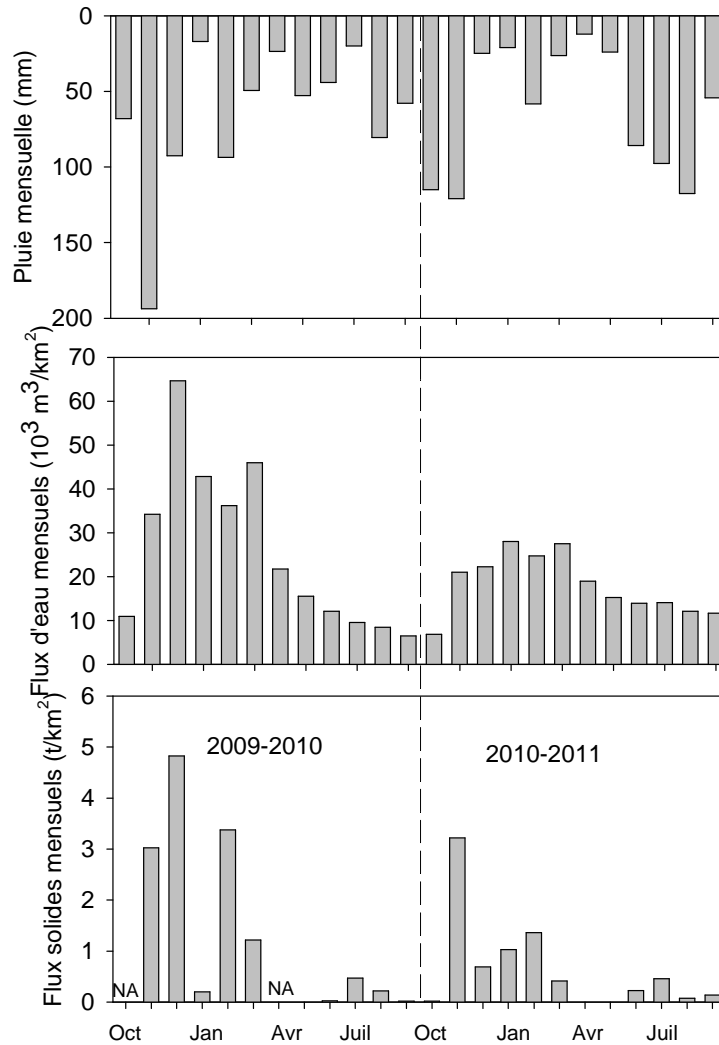
Figure 8.11 : Dynamique mensuelle de la pluviométrie, des flux hydriques et des flux solides
