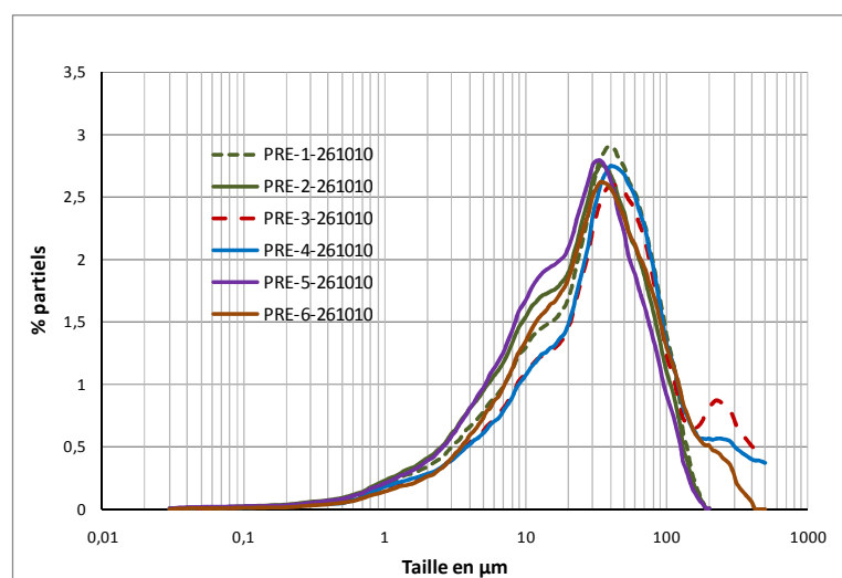
Figure 3.15 : Courbes granulométriques partielles volumiques de la fraction fine (<500 microns) des échantillons prélevés (avec matières organiques) le 26/10/2010.
