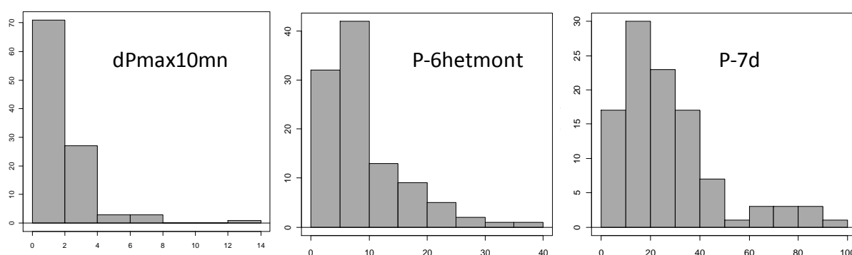
Figure 7.3 : Fréquence de l'augmentation maximale entre deux mesures (dPmax10mn), de la pluie cumulée pendant 6 heures avant le début et pendant la montée de crue (P-6h et mont) et de la pluie cumulée pendant 7 jours avant le début de la crue (P-7d).
