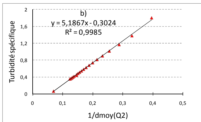
Figure 4.10: Relation entre la turbidité spécifique moyenne (FTU/mg/l) et 1/d_{moy}(Q2) ( \mu\text{m}^{-1} ) pour le sédiment bi-dispersé.
