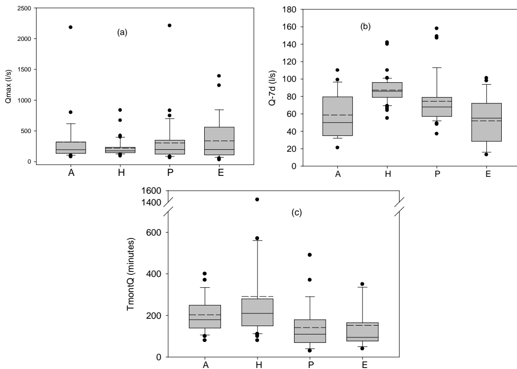
Figure 7.13 : Box plots, en fonction des saisons, du débit maximal ( Q_{max} ) (a), du débit moyen pendant 7 jours avant la crue ( Q_{-7d} ) (b) et du temps de montée du débit ( T_{montQ} ) (c) entre octobre 2005 et septembre 2008.
