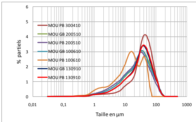
Courbes granulométriques partielles des sédiments piégés entre 30/4/10 ; 20/5/10 et 10/6/2010 et 13/9/2010.
