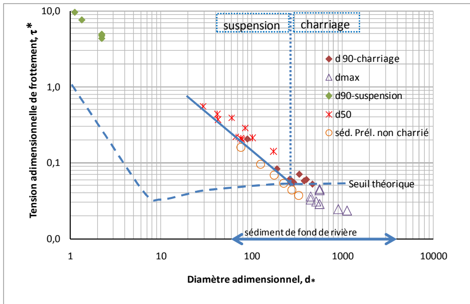
Figure 3.17 : Shields ou tension réduite de frottement, \tau^* , en fonction du diamètre réduit du granulat, d^* , calculé sur le diamètre d_{50} ou d_{90} ou d_{max} du sédiment piégé et d_{grossier} du sédiment prélevé.
