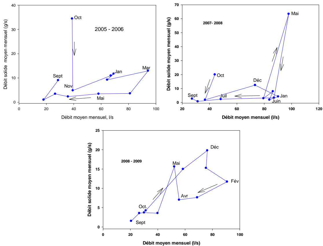
Figure 5.6 : Relation entre le débit solide et le débit moyens mensuels.
