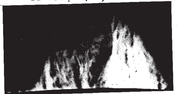
filament quiescent au bord du disque (H \alpha )
