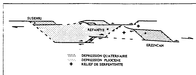
FIG. 4. - Schéma structural interprétatif de la région de Refaye (Refahiye) - Erzincan.
