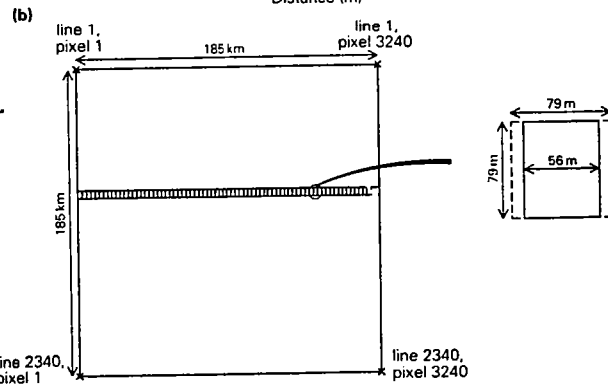
Fig.1.4: Variation de la réflectance sur une scène Landsat-MSS. D'après S.A. Drury (1987).
