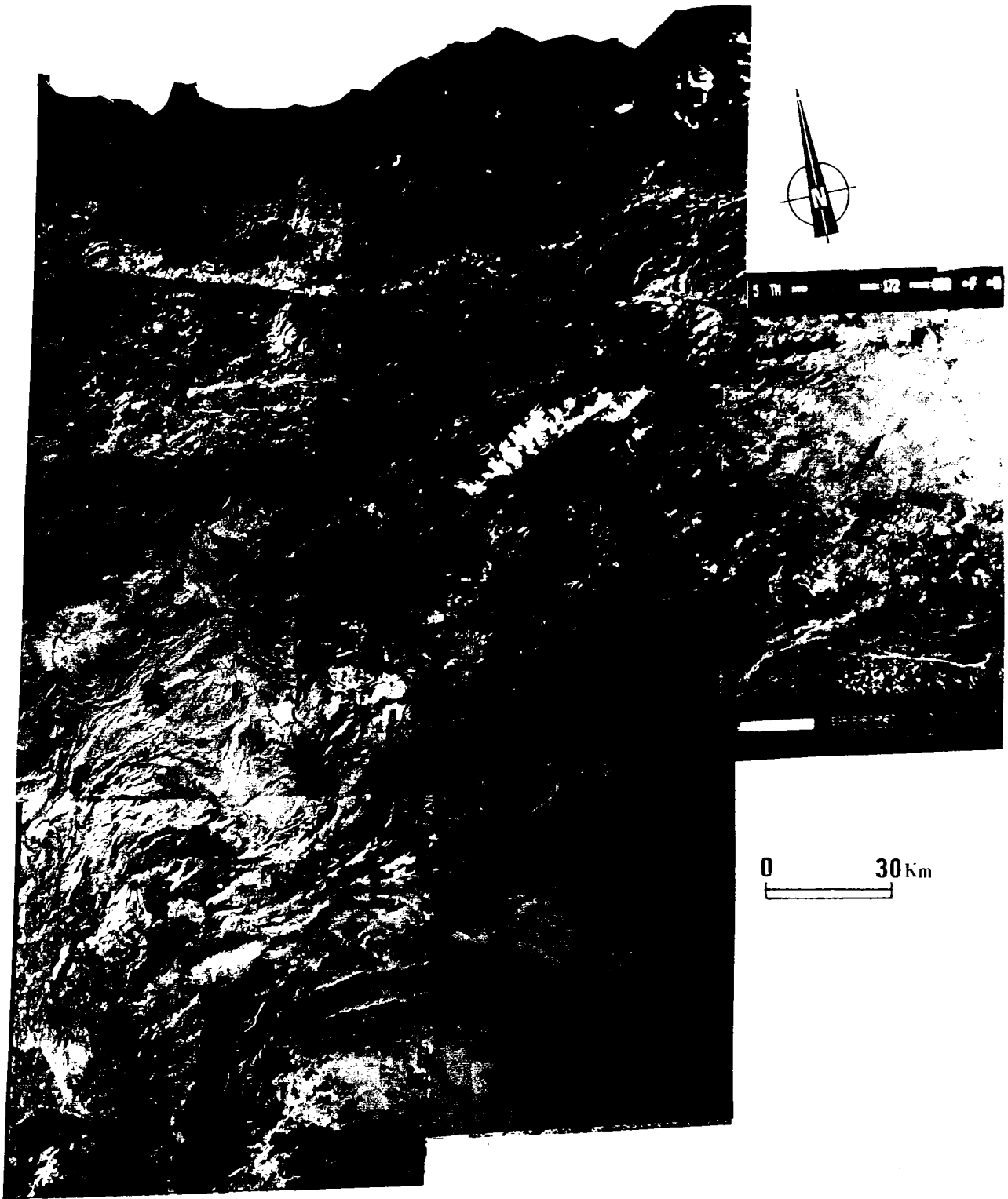
Planche 2: mosaïque de l'Anatolie orientale réalisée à partir d'images Landsat-TM.
