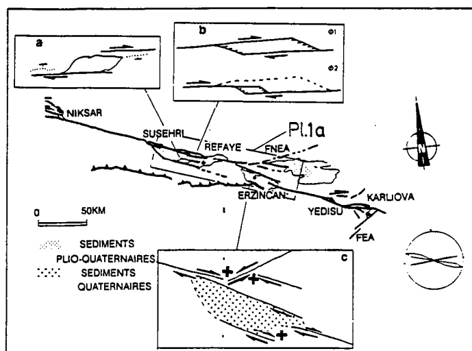
FIG. 3. - Carte structurale du segment oriental de la FNA. La rosace de fréquences correspond aux directions de failles de la région d'Erzincan-Karliova (pour la localisation cf. figure 2).
