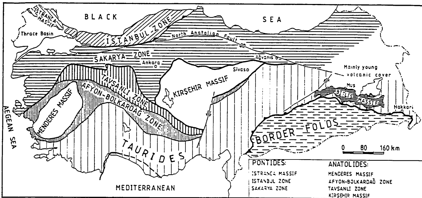
Fig.2.6: carte tectonique de la Turquie montrant les différents domaines tectoniques des Pontides et des Anatolides. La limite entre la zone de Sakaya et d'Istambul correspondrait à la trace d'une paléosuture fermée au Jurassique inférieur. D'après Okay (1986).
