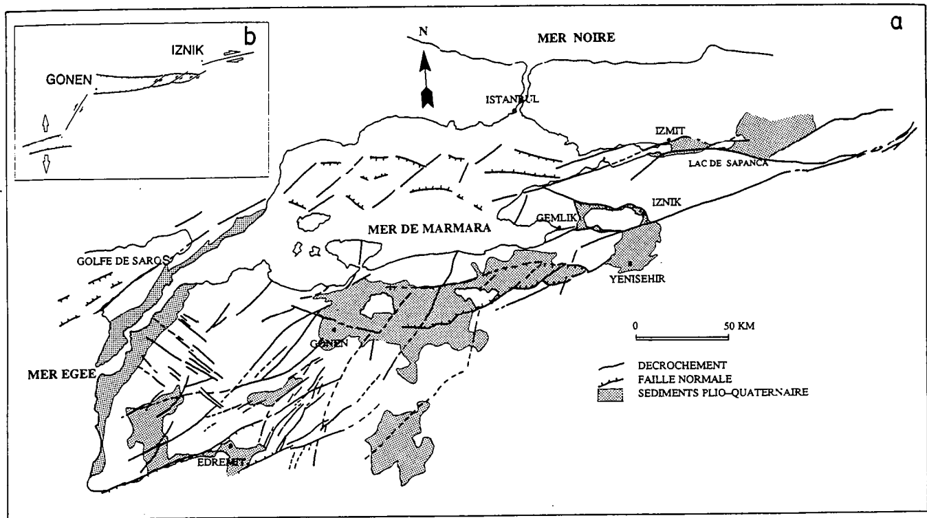
FIG. 8a. - Carte structurale du segment occidental de la FNA (pour la localisation cf. figure 2). 8b. - Transition du mécanisme d'ouverture oblique au sud d'Iznik vers un mécanisme purement extensif dans la région des fossés de Gonen et d'Edremit.
