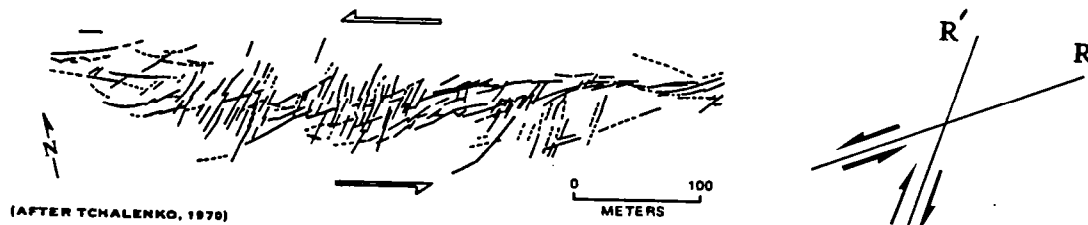
Fig. 1 - 3. Exemple naturel de Riedel R synthétiques et de Riedel R' antihétiques d'un décrochement sénestre. Ces structures ont été créées lors du tremblement de terre de Dash-e Bayaz (Iran) décrit par Tchalenko and Ambraseys (1970), Tchalenko (1970).
