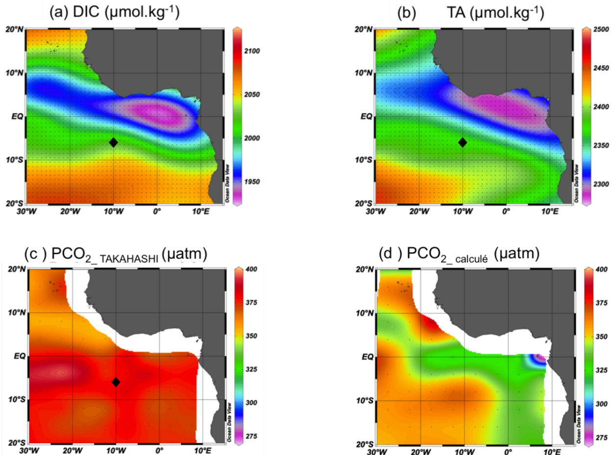
Figure I.10 – Carte issue de la climatologie annuelle [Key et al., 2004] pour DIC(a) et TA (b) et de [Takahashi et al., 2009] pour la \text{pCO}_2 (c). \text{pCO}_2 calculée correspond aux \text{pCO}_2 calculée à partir du DIC et de la TA de la climatologie avec le programme de [Lewis et Wallace, 1998].
