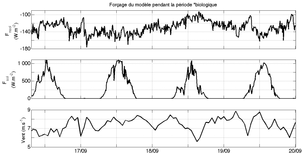
Figure IV.16 – Evolution temporelle du flux non solaire ( F_{n\text{sol}} en \text{W.m}^{-2} ), du flux solaire ( F_{\text{sol}} en \text{W.m}^{-2} ) et de la vitesse de vent ( \text{m.s}^{-1} ).
