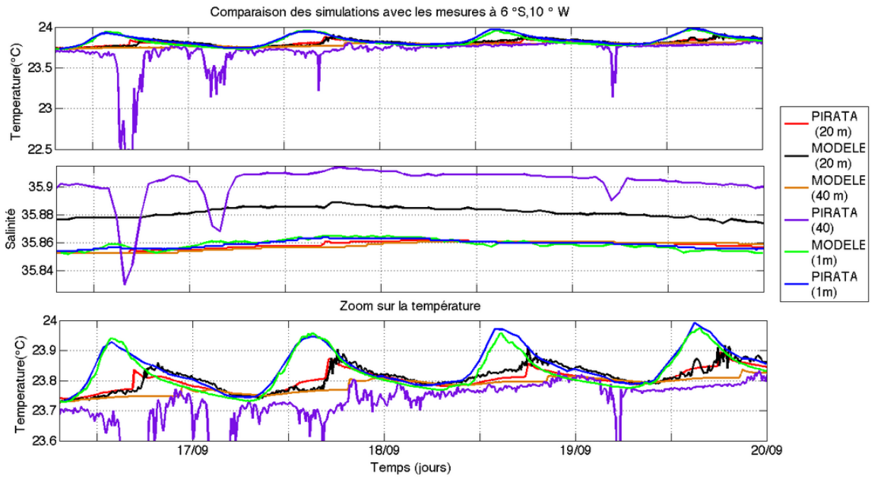
Figure IV.18 – Evolution de température et de salinité simulées et mesurées pendant la période "biologique" à 1 m , 20 m et 40 m. En bas, évolution de la température de 23,5° C à 24° C sur la même période.
