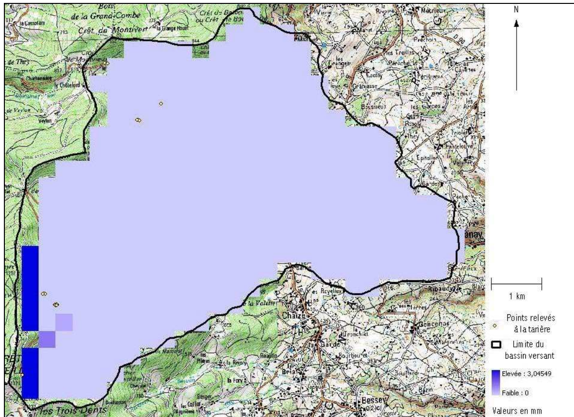
Figure 75 : Valeurs de la Réserve Utile sur le Bassin versant de la Valencize à Chavaignay à la fin du mois d'août - Période 1971-2000 (ATLAS DU PARC NATUREL REGIONAL DU PILAT, INSTITUT GEOGRAPHIQUE NATIONAL, METEO-FRANCE)
