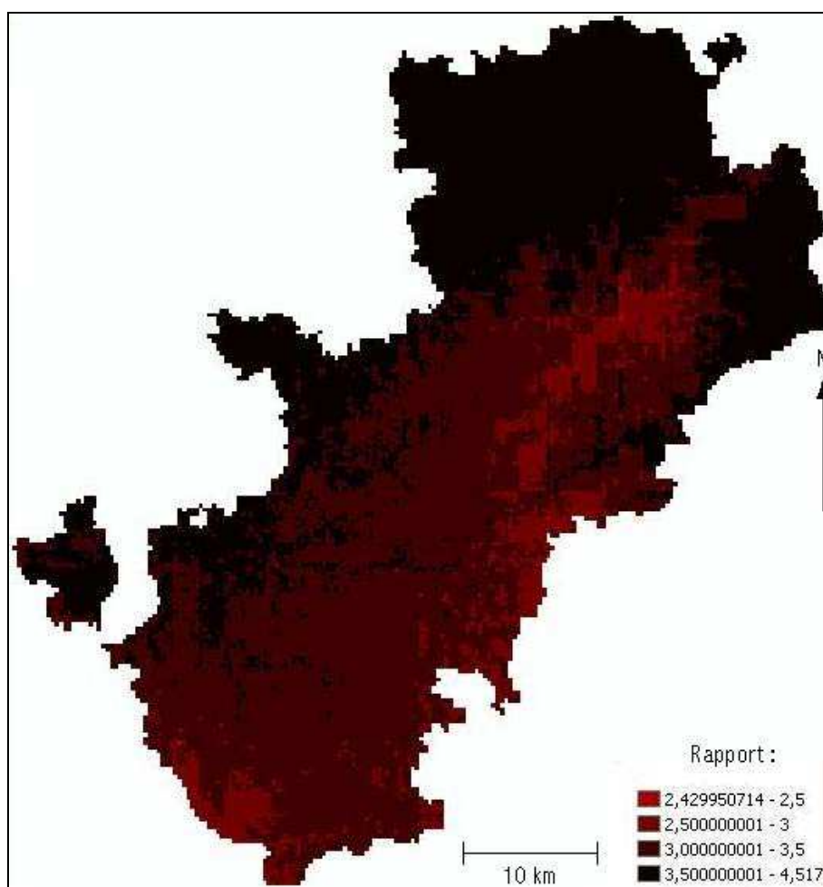
Figure 170 : Rapport entre les températures moyennes d'Avril 2003 à Juin 2003 et les températures moyennes de la période de référence 1971-2000 (METEO-FRANCE)
