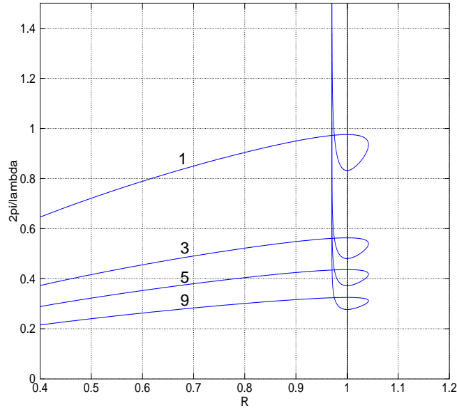
FIGURE 3.21 – Rapport R entre les flux d'énergie à l'intérieur et à l'extérieur de la couche métallique, pour différentes valeurs de |\epsilon_2| , pour |\epsilon_1/\epsilon_2| = 0.98 .
