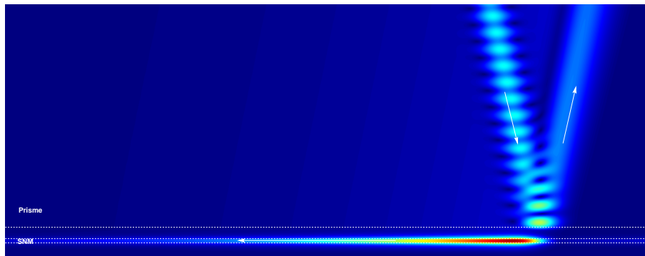
FIGURE 3.27 – Mode de film fin contra-propagatif excité par couplage évanescent par un faisceau incident (angle d'incidence : 64.6^\circ , waist : 5\lambda ) dans un prisme ( \varepsilon = 5 , \mu = 1 ). Le MEN est caractérisé par \varepsilon = -0.5 , \mu = 1 , h_1 = 0.057\lambda et le milieu extérieur par \varepsilon = 1.1 et \mu = 1 .
