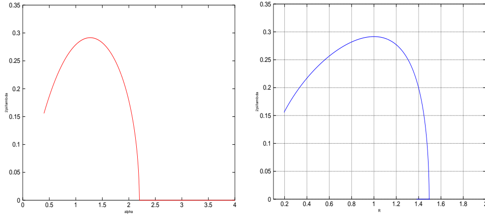
FIGURE 3.24 – Courbe de dispersion d'une couche d'argent ( \varepsilon_{Ag} = -5.51 à 420 nm) d'épaisseur unité, entourée de niobate de lithium ( \varepsilon_1 = 5.5 ).
