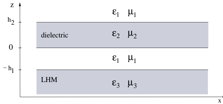
FIGURE 3.15 – Le guide diélectrique et la surface du milieu main-gauche sont séparés par une distance h_1 et plongés dans un milieu caractérisé par \epsilon_1 et \mu_1 .
