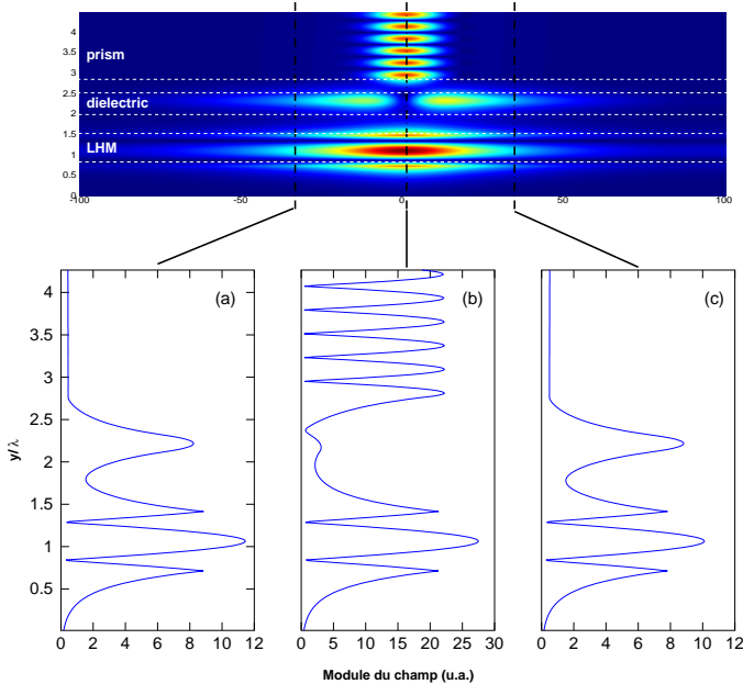
FIGURE 3.4 – Module du champ selon l'axe Ox.
