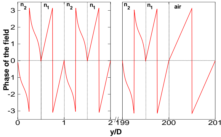
FIGURE 4.10 – Phase du champ électromagnétique du faisceau auto-collimaté considéré à la figure 4.9, en x = 0 .
