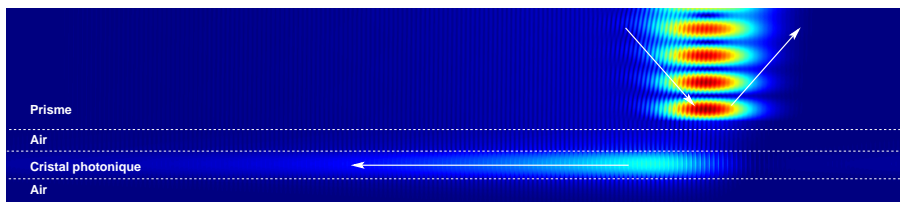
FIGURE 3.31 – Mode guidé contra-propagatif dans une couche de cristal photonique, excitée par couplage évanescent par un faisceau incident (angle d'incidence : 47^\circ , waist : 5\lambda ) dans un prisme ( \epsilon = 9 , \mu = 1 ).
