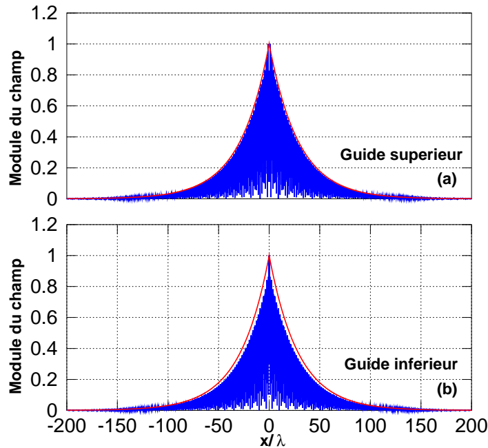
FIGURE 3.8 – Module du champ au centre (a) du guide diélectrique, et (b) du guide gauche. Les courbes bleues sont obtenues d’après la simulation (figure 3.7) et les courbes rouges sont données par le modèle (3.9).
