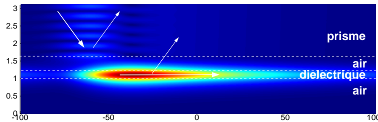
FIGURE 1.9 – Simulation identique à celle de la figure 1.8 mais le prisme est bien plus proche de la couche diélectrique ( 0.4\lambda au lieu de 1.6\lambda ).
