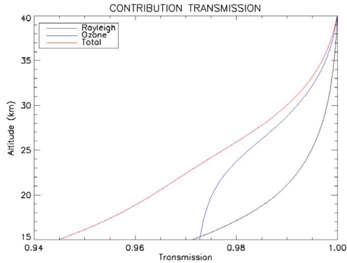
Figure 20. Contribution moyenne entre 20°S-20°N de la transmission double sens due à la diffusion moléculaire (Rayleigh) et à l'absorption par l'ozone durant la période 01-16 août 2006.
