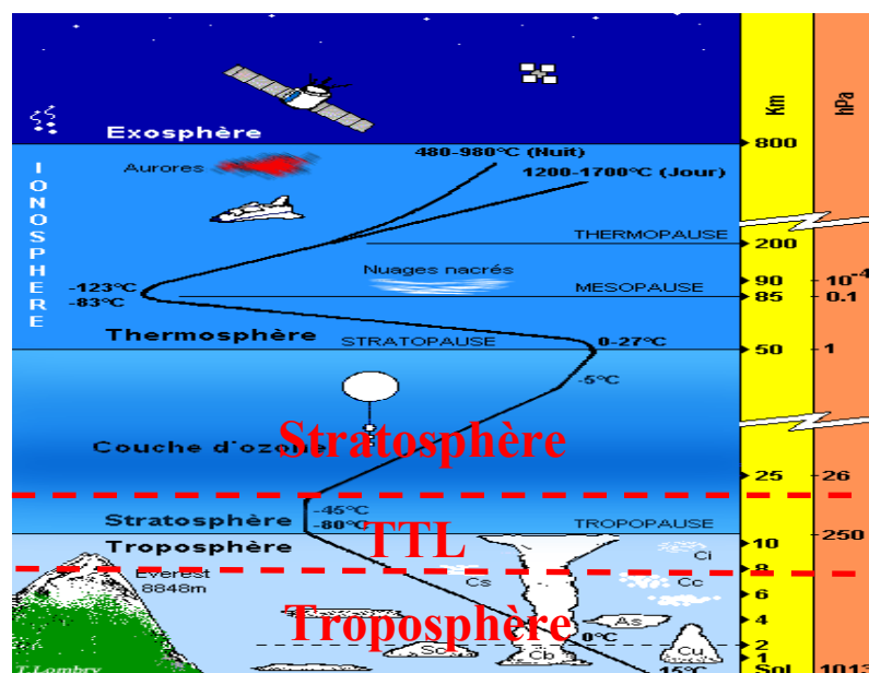
Figure 1. Profil vertical de température en atmosphère standard. Du sol à 12-17 km, se situe la troposphère (gradient thermique négatif). La stratosphère est comprise entre ce niveau et 50 km (gradient thermique positif). TTL en rouge (Tropical Transition Layer), zone de transition entre la troposphère et la stratosphère aux tropiques.
