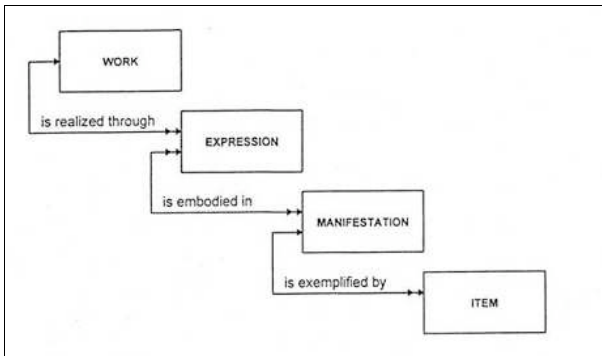
Figure 11 : Entités et relations `rimaires du mod`le IFLA
