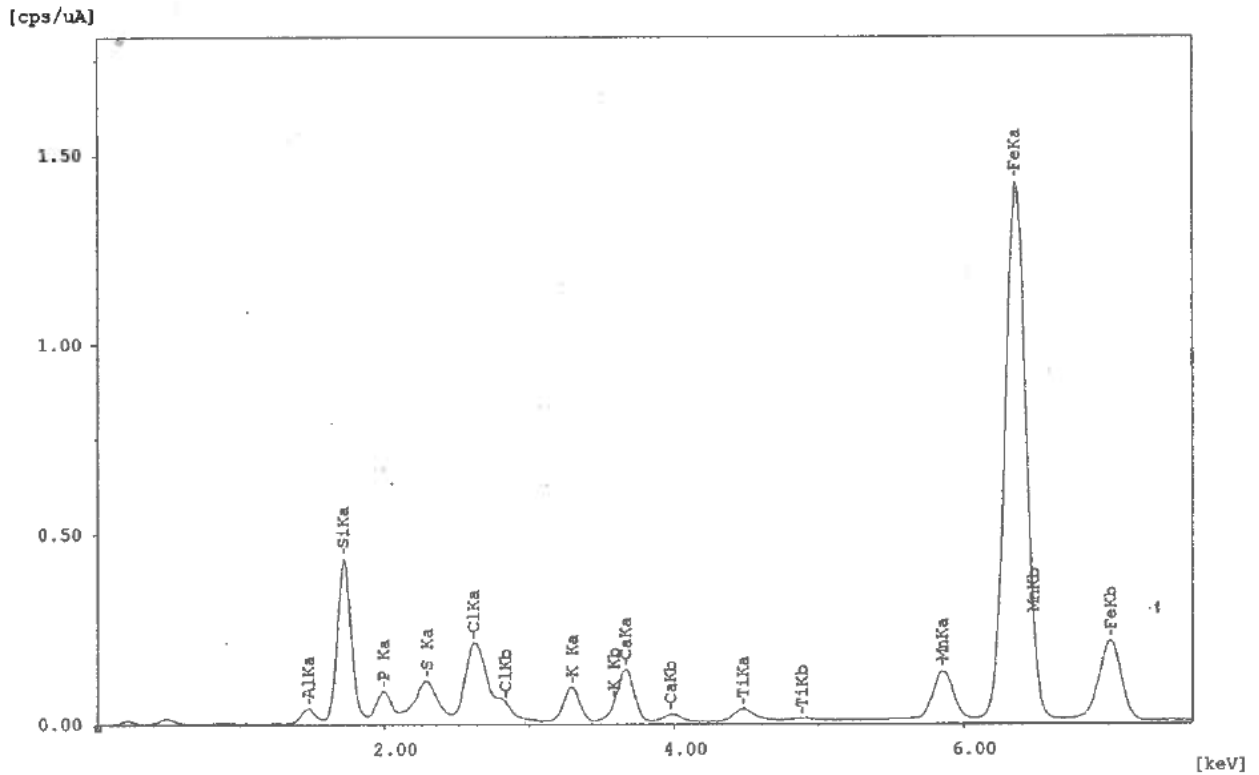
Figure 4-10 Spectre de l'analyse chimique par fluorescence X des particules retenues par le système racinaire des plantes (basse énergie)
