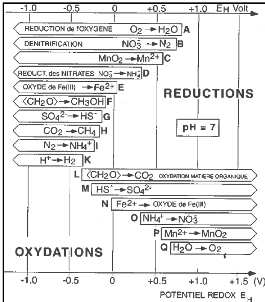
Figure 1-14 Domaines de p_e et de potentiel d'oxydoréduction valables à \text{pH} = 7 pour des réactions catalysées par les microorganismes (Sigg et al., 2000)
