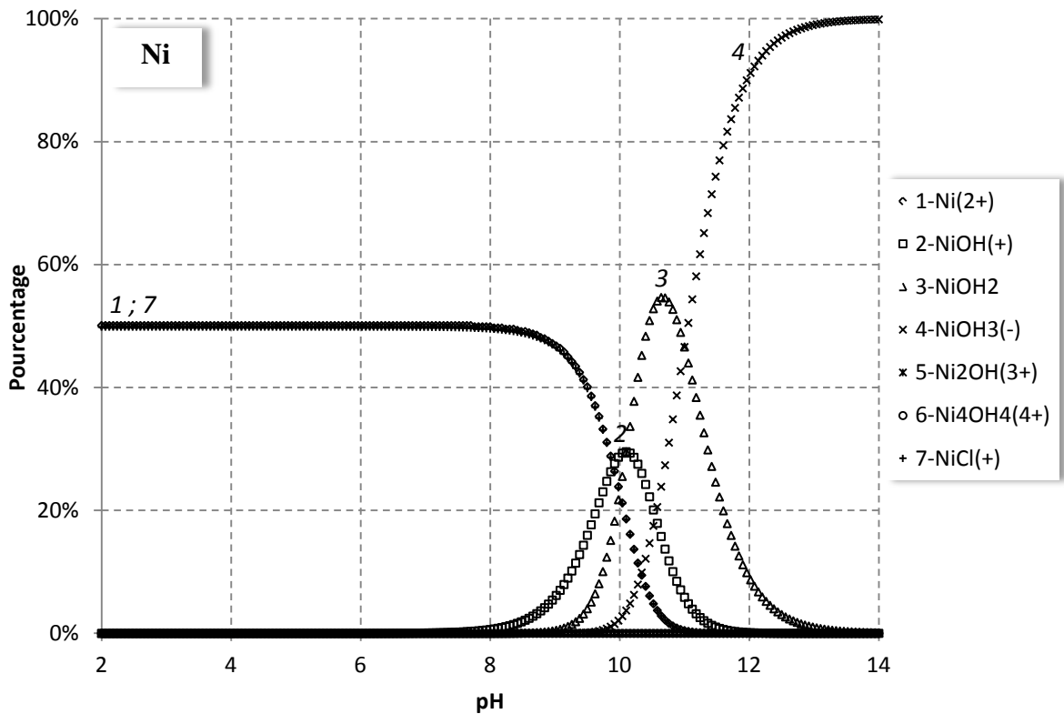
Figure 2-7 Diagramme de spéciation de Ni en fonction du pH, déterminé pour T = 25^\circ\text{C} , I = 0,01 \text{ M} , une concentration en nickel égale à celle mesurée dans le plan d'eau permanent du bassin de rétention ( 1,7 \times 10^{-7} \text{ M} ) et [\text{Cl}^-] = 2,8 \text{ mM}
