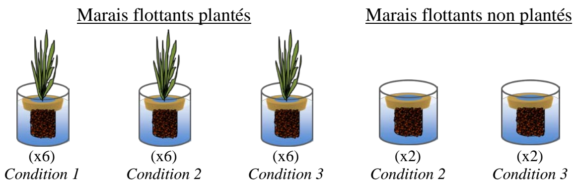
Figure 3-3 Schématisation du dispositif expérimental et des conditions opératoires testées
