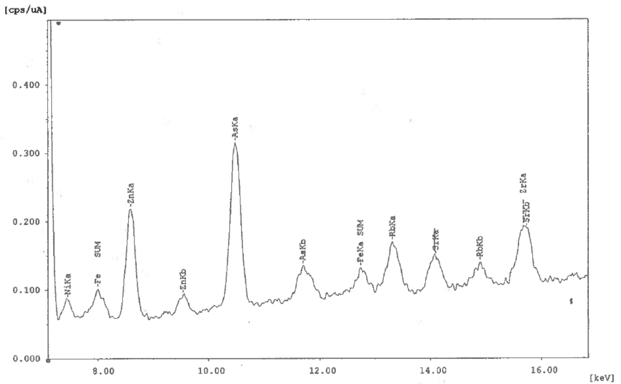
Figure 4-11 Spectre de l'analyse chimique par fluorescence X des particules retenues par le système racinaire des plantes (haute énergie)
