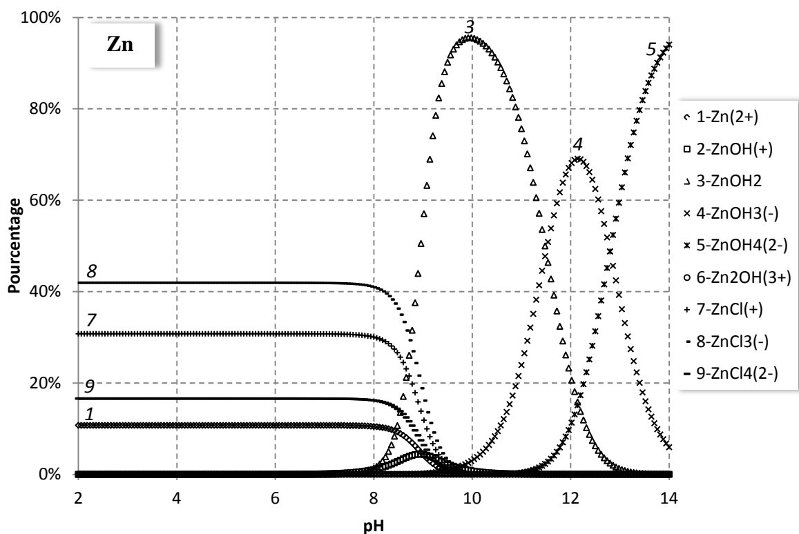
Figure 2-9 Diagramme de spéciation de Zn en fonction du pH, déterminé pour T = 25^{\circ}\text{C} , I = 0,01 \text{ M} , une concentration en cuivre égale à celle mesurée dans le plan d'eau permanent du bassin de rétention ( 6,0 \times 10^{-7} \text{ M} ) et [\text{Cl}^-] = 2,8 \text{ mM}
