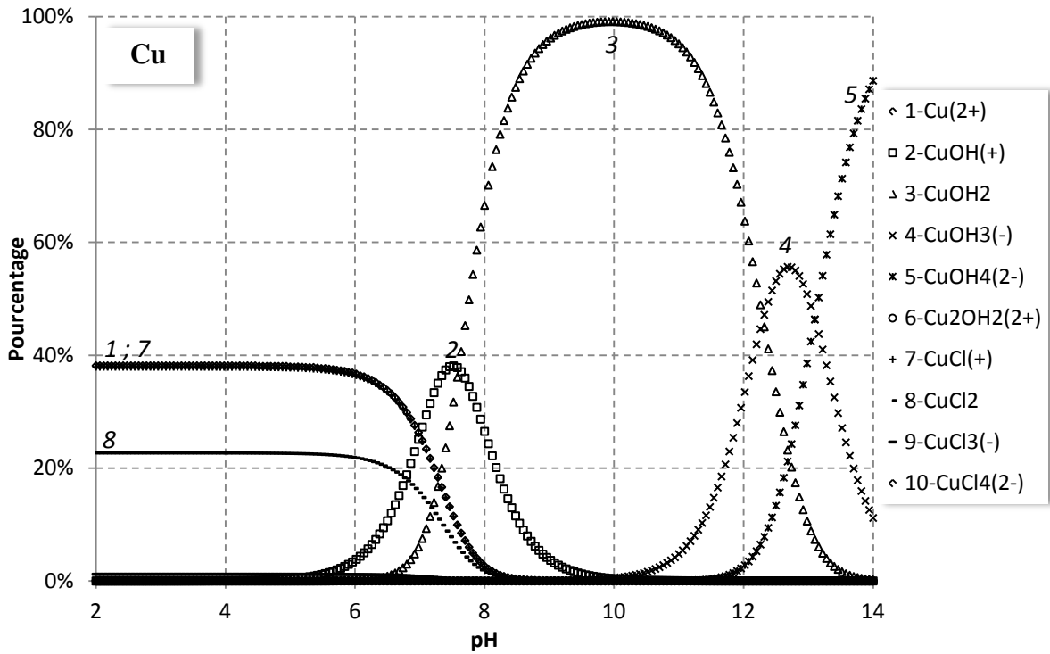
Figure 2-6 Diagramme de spéciation de Cu en fonction du pH, déterminé pour T = 25^\circ\text{C} , I = 0,01 \text{ M} , une concentration en cuivre égale à celle mesurée dans le plan d'eau permanent du bassin de rétention ( 2,5 \times 10^{-8} \text{ M} ) et [\text{Cl}^-] = 2,8 \text{ mM}
