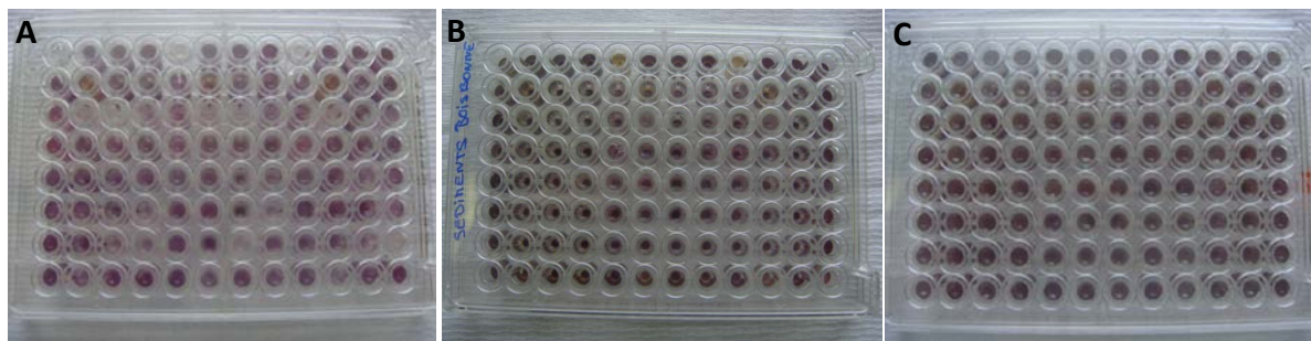
Figure 4-13 Microplaques Biolog Ecoplate inoculées avec l'eau du bassin (A) et les suspensions microbiennes obtenues à partir des sédiments (B) et du biofilm formé à la surface des racines des plantes (C) (exemple de Carex riparia présenté ici)
