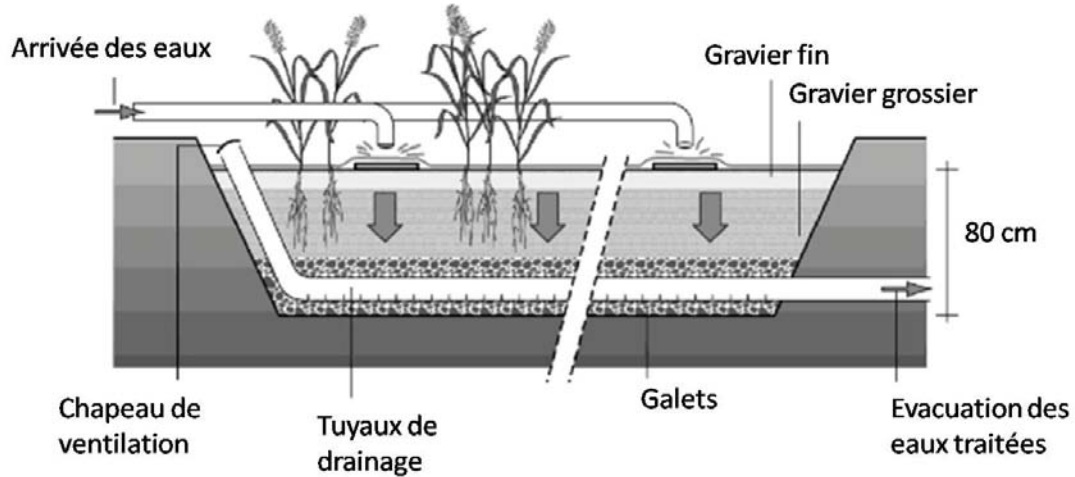
Figure 1-20 Coupe transversale schématique d'un filtre planté à percolation verticale : alimentation par bâchées (Agence de l'Eau Rhône Méditerranée et Corse 1999)
