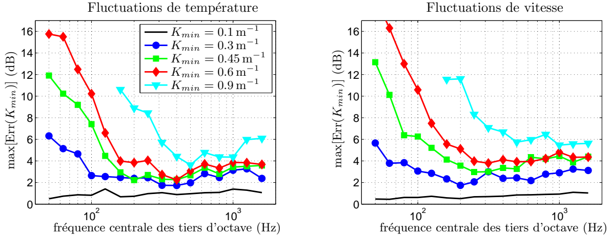
FIG. 1.26 – Spectre en tiers d’octave du maximum de \text{Err}(K_{\min}) pour des fluctuations de température (à gauche) et de vitesse (à droite). En dessous de 125 Hz, le maximum est calculé jusqu’à une distance de 1000 m et une hauteur de 50 m ; au-dessus de 160 Hz, le maximum est calculé jusqu’à une distance de 500 m et une hauteur de 50 m.
