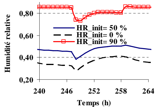
Figure 3. 81 : Humidité relative du local en fonction des conditions initiales.
