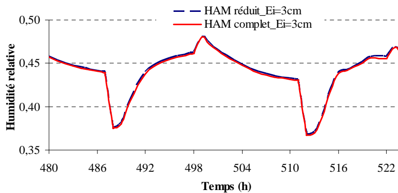
Figure 4.8 : Humidité relative du local pour les deux modèles et pour une couche de l'enduit en chanvre-chaux intérieur de 3 cm.
