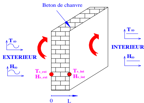
Figure 3. 4: Paroi en béton de chanvre soumise à une condition climatique périodique.
