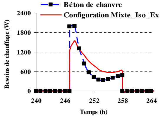
Figure 3.89: Besoins de chauffage en fonction des configurations étudiées pendant un jour.
