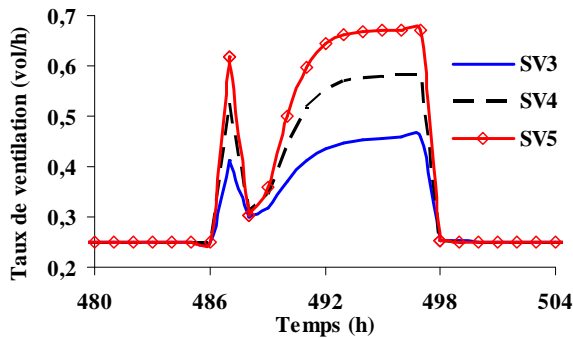
Figure 3. 72 : Variation du taux de ventilation pendant un jour.
