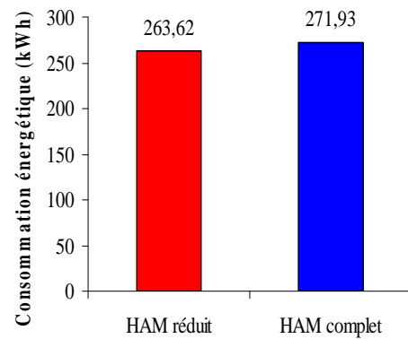
Figure 4.7b : Consommations énergétiques.
