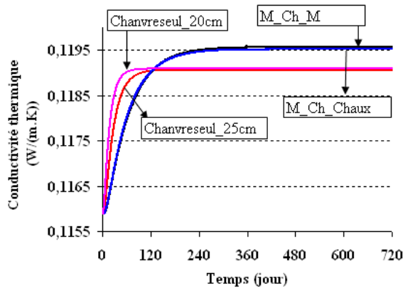
Figure 3. 19 : Conductivité thermique.
