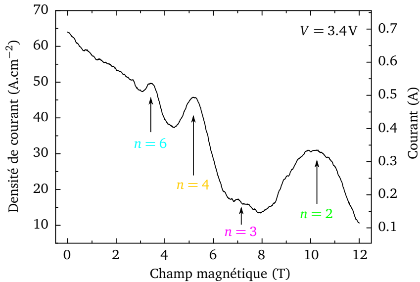
FIGURE 3.25 – Mesure de magnéto-transport sur le ridge. Courant et densité de courant en fonction du champ magnétique à tension constante V = 3.4\text{V} . L'expérience a été réalisée à T = 4.5\text{K} le champ magnétique étant balayé de 0 à 12 T.
