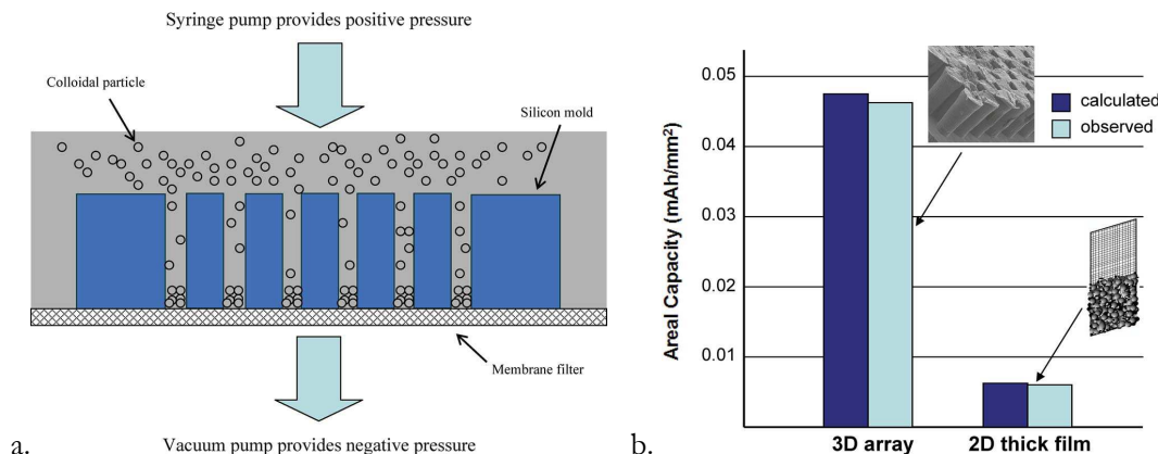
Figure 1-8 : Schéma du procédé de dépôt colloïdal (a), comparaison des valeurs de capacité surfacique calculées et obtenues pour des demi-cellules MCMC en configuration planaire et 3D (b) [10].
