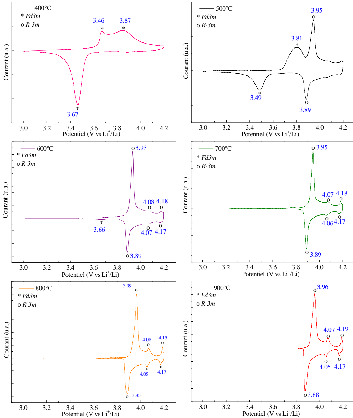
Figure 2-23 : Voltamétrie cyclique des électrodes composites de LiCoO 2 synthétisé entre 400 et 900°C (5 μV.s -1 ).
