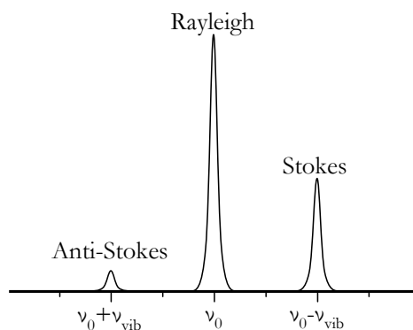
Figure A-9 : Diffusion Raman et Rayleigh à une fréquence d'excitation de \nu_0 et une fréquence de vibration de la molécule de \nu_{vib} .
