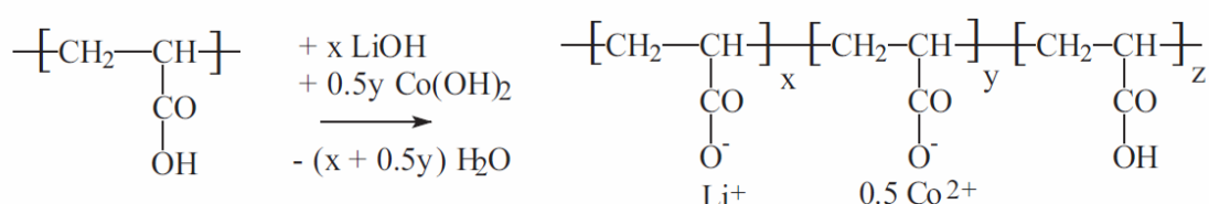
Figure 1-28 : Représentation schématique de la formation du réseau organique à base d'acide polyacrylique PAA et d'hydroxydes métalliques [99].
