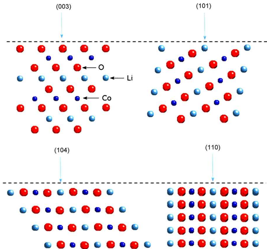
Figure 1-27 : Illustration des orientations préférentielles des grains de LiCoO 2 par rapport à la direction du flux de courant dans le micro-accumulateur [77].
