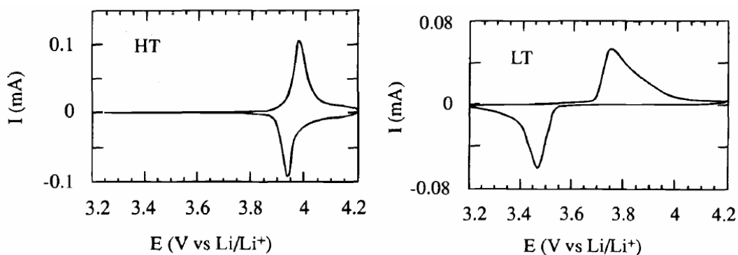
Figure 1-24 : Voltamétrie cyclique obtenue pour les phases \text{LiCoO}_2 R\bar{3}m (HT) et Fd3m (LT) ( 40 \mu\text{V}\cdot\text{s}^{-1} ) [60].
