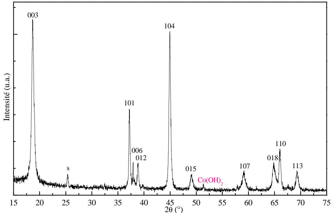
Figure 3-46 : Diffractogramme des rayons X enregistré en incidence rasante du matériau synthétisé dans les conditions B (s désigne le substrat Ti, les réflexions indiquées correspondent à \text{LiCoO}_2 R\bar{3}m ).
