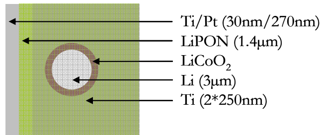
Figure 2-43 : Vue schématique de l'empilement tout solide réalisé.
