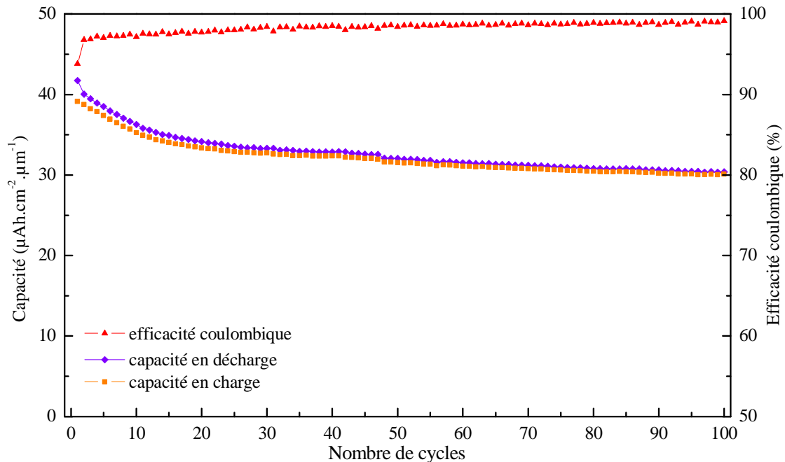
Figure 3-42 : Évolution de la capacité en charge et en décharge et de l'efficacité coulombique pour le film mince synthétisé dans les conditions B.
