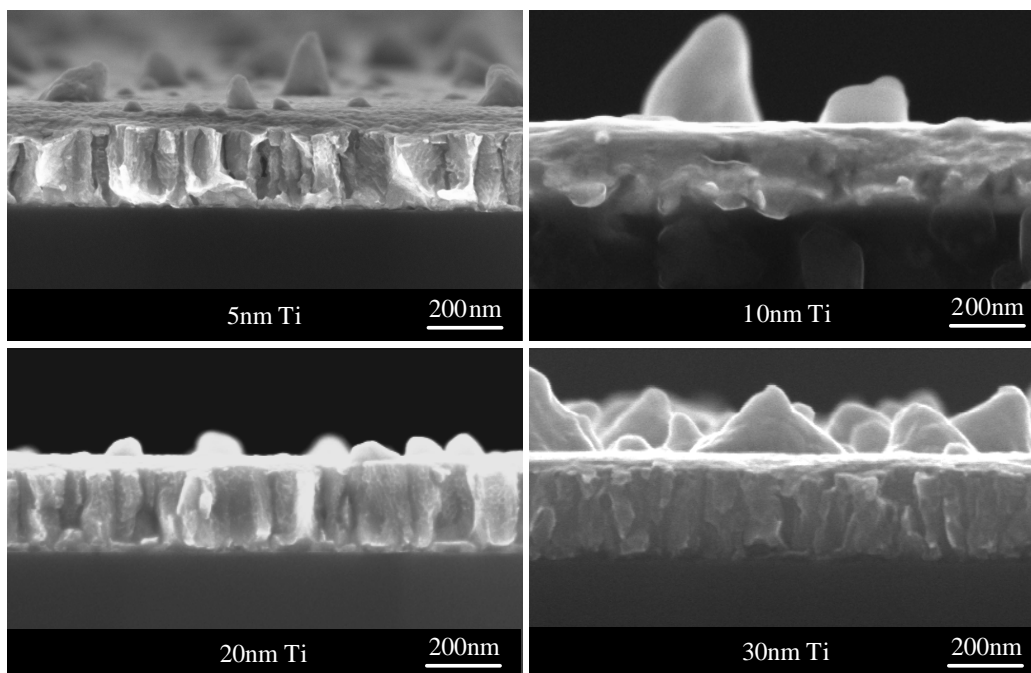
Figure 2-35 : Images MEB des substrats n°1' à 4' ayant subi un recuit à 600^\circ\text{C} .
