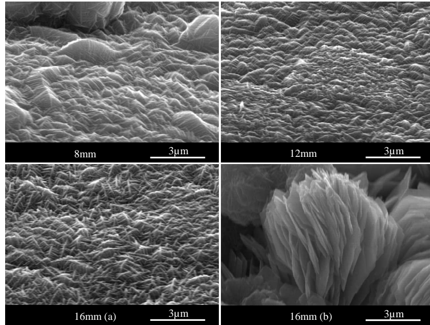
Figure 3-36 : Images MEB de surface de films minces déposés à différents espacements anode/cathode.
