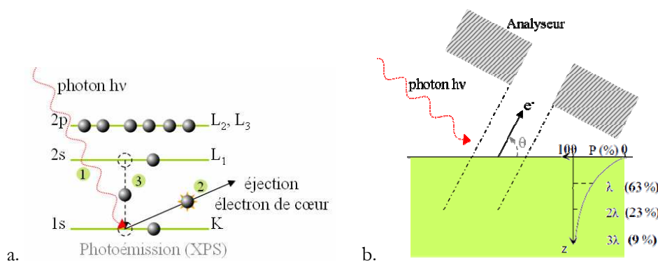
Figure A-5 : Schéma de principe de la photoémission pour la spectroscopie XPS (a), évolution du signal en fonction de la profondeur d'échantillon (b) d'après [1].
