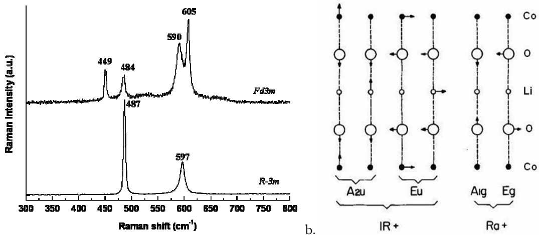
Figure 1-23 : Diagramme obtenu par spectroscopie Raman pour les phases \text{LiCoO}_2 R\bar{3}m et Fd3m (a) [66], déplacements atomiques de la phase rhomboédrique correspondant aux modes actifs en IR et en Raman (b) [63].
