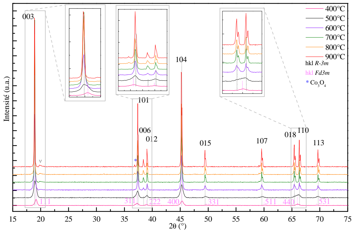
Figure 2-16 : Diffractogrammes des rayons X de poudres obtenues à différentes températures de traitement thermique ( \nu correspond à la fluorescence X du cobalt (cf Annexes), les réflexions indiquées correspondent à \text{LiCoO}_2 R\bar{3}m ).
