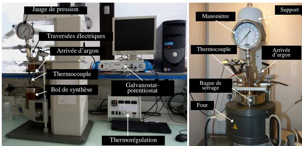
Figure 3-10 : Montage utilisé pour la synthèse par électrodépôt en conditions hydrothermales.
