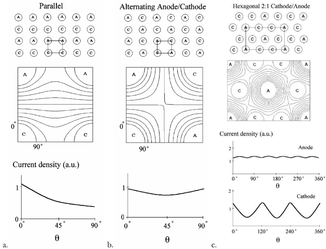
a. Figure 1-9 : Vue schématique d'un accumulateur 3D avec une configuration parallèle (a), une configuration alternée (b) et une configuration hexagonale alternant cathode et anode (c) associée à la répartition des lignes de champs autour des électrodes et à l'évolution de la densité de courant (unité arbitraire) à la surface de l'électrode en fonction de l'angle \theta [11].
