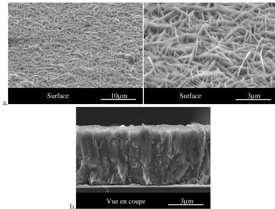
Figure 3-45 : Images MEB en surface (a) et en coupe (b) d'un dépôt réalisé dans les conditions B.
