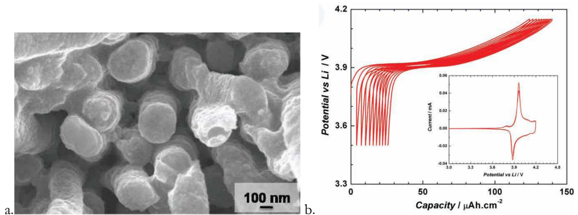
a. Figure 1-10 : Résultats obtenus par dépôt sol-gel de \text{LiCoO}_2 sur des plots d'aluminium : image MEB (a), cyclage galvanostatique (C/10) et voltamétrie cyclique ( 10 \mu\text{V}\cdot\text{s}^{-1} ) obtenus en pile bouton (b) [12].
