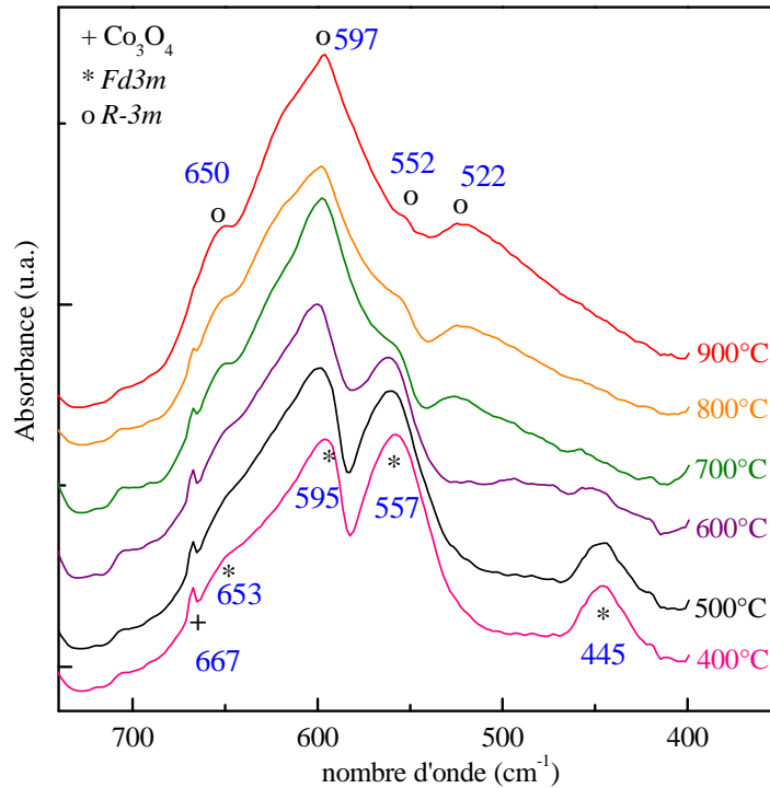
Figure 2-17 : Spectres IR des poudres synthétisées entre 400 et 900°C (1 % en masse dans KBr).
