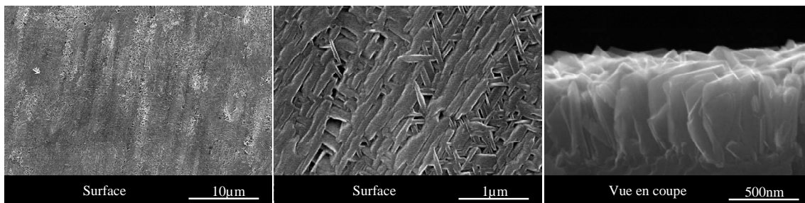
Figure 3-38 : Images MEB de surface et en coupe du dépôt synthétisé dans les conditions A.
