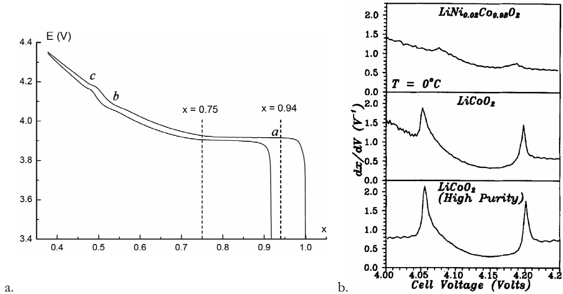
Figure 1-25 : Courbe galvanostatique d'un accumulateur Li/ \text{Li}_x\text{CoO}_2 (a) [69], dérivée de la composition x en fonction du potentiel à proximité des plateaux b et c (b) [70].
