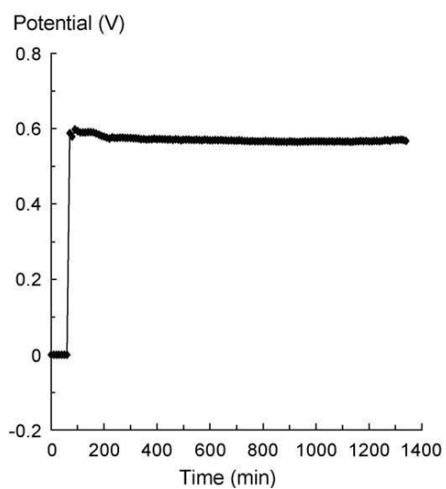
Figure 1-34 : Évolution du potentiel de l'électrode Co (réf. Ag/AgCl) en fonction du temps lors de la synthèse en voie hydrothermale du \text{LiCoO}_2 à 150^\circ\text{C} et 4 \text{ mol.L}^{-1} de \text{LiOH} [153].
