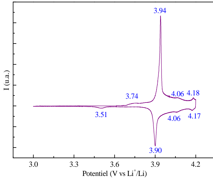
Figure 2-31 : Voltamétrie cyclique d'une électrode déposée par sol-gel sur une feuille d'or avec un recuit à 600°C ( 5 \mu\text{V}\cdot\text{s}^{-1} , en électrolyte liquide).
