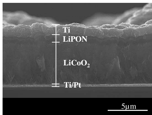
Figure 3-53 : Image MEB en coupe d'un empilement tout solide \text{LiCoO}_2/\text{LiPON}/\text{Ti} .
