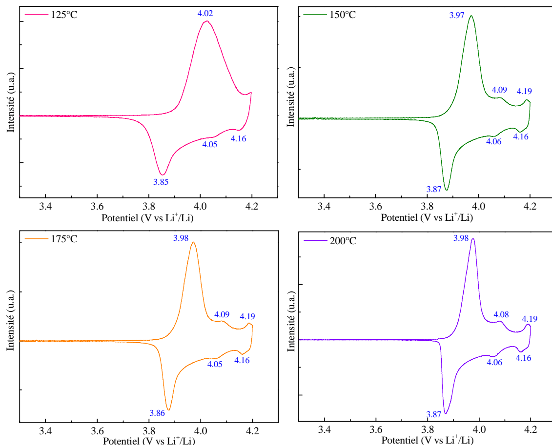
Figure 3-31 : Voltamogrammes obtenus en électrolyte liquide lors du premier cycle pour des films minces synthétisés à différentes températures ( 20\mu\text{V}\cdot\text{s}^{-1} ).
