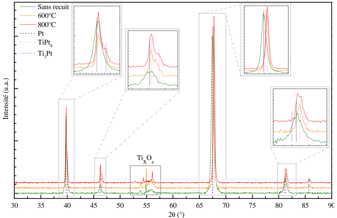
Figure 2-34 : Diffractogrammes des rayons X du substrat 1' sans traitement thermique, recuit à 600^\circ C et 800^\circ C .
