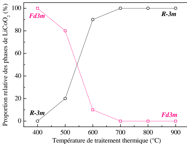
Figure 2-19 : Évolution de la proportion relative des phases \text{LiCoO}_2 Fd3m et R\bar{3}m en fonction de la température de recuit finale.
