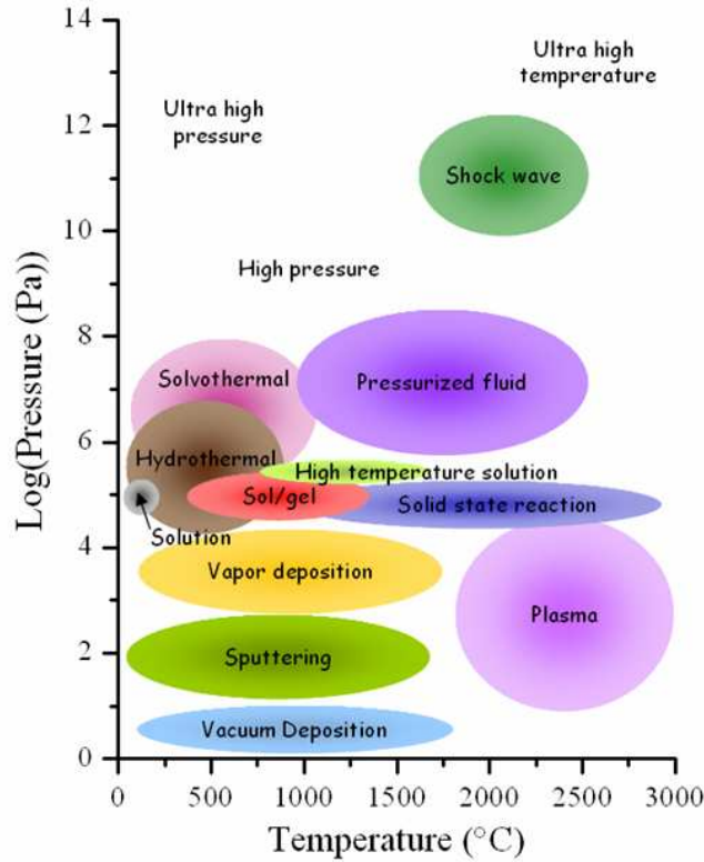
Figure 1-35 : Diagramme schématisé log(P)-T des principales techniques de synthèse de matériaux céramiques d'après [155].
