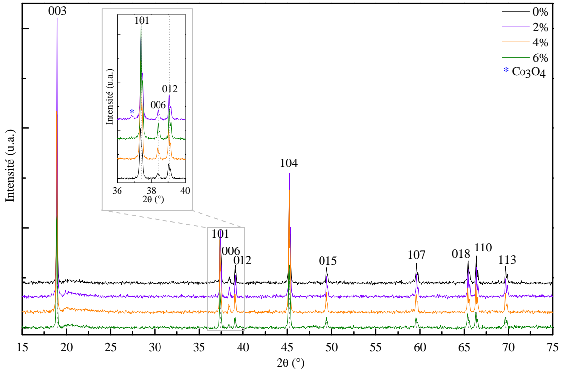
Figure 2-10 : Diffractogrammes des rayons X des poudres obtenues à 800°C à différentes surstoichiométries de lithium (les réflexions indiquées correspondent à \text{LiCoO}_2 R\bar{3}m ).
