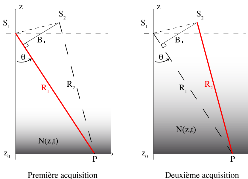
FIGURE 1.5 – Indice de réfraction et acquisition SAR - Schéma présentant l'influence des variations de l'indice de réfraction de l'air N sur les délais zénithaux et le long de la ligne de visée, pour deux acquisitions SAR. Voir figure 1.1 pour la nomenclature.
