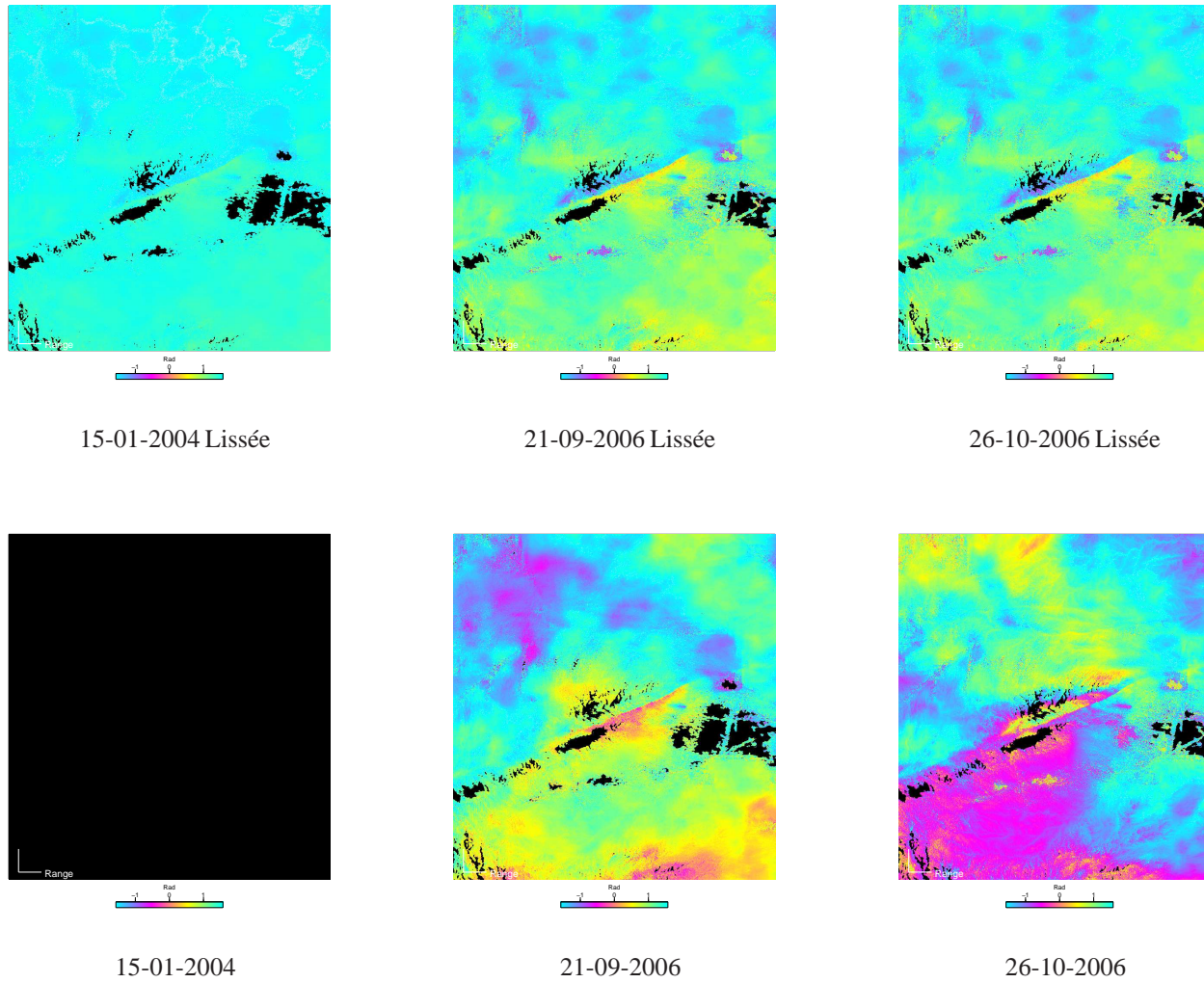
FIGURE B.3 – Série temporelle et effets du lissage gaussien - Résultats de l'analyse en séries temporelle lissée, présentée au chapitre 5. En haut, on peut voir les reconstitution des valeurs de phase lissées, en bas, non lissées.
