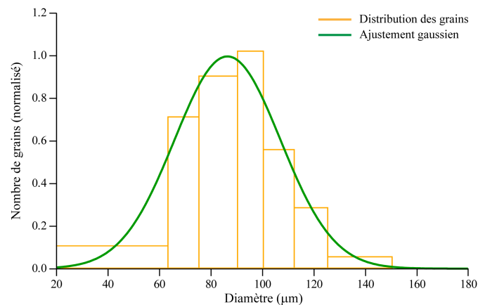
FIG. 3.1: Granulométrie des billes de céramique utilisées pour nos expériences en laboratoire. La gaussienne ajustée à la distribution est centrée sur le diamètre moyen D_{P0} = 87 \mu\text{m} et a pour largeur à mi-hauteur H_{1/2} = 24 \mu\text{m} .
