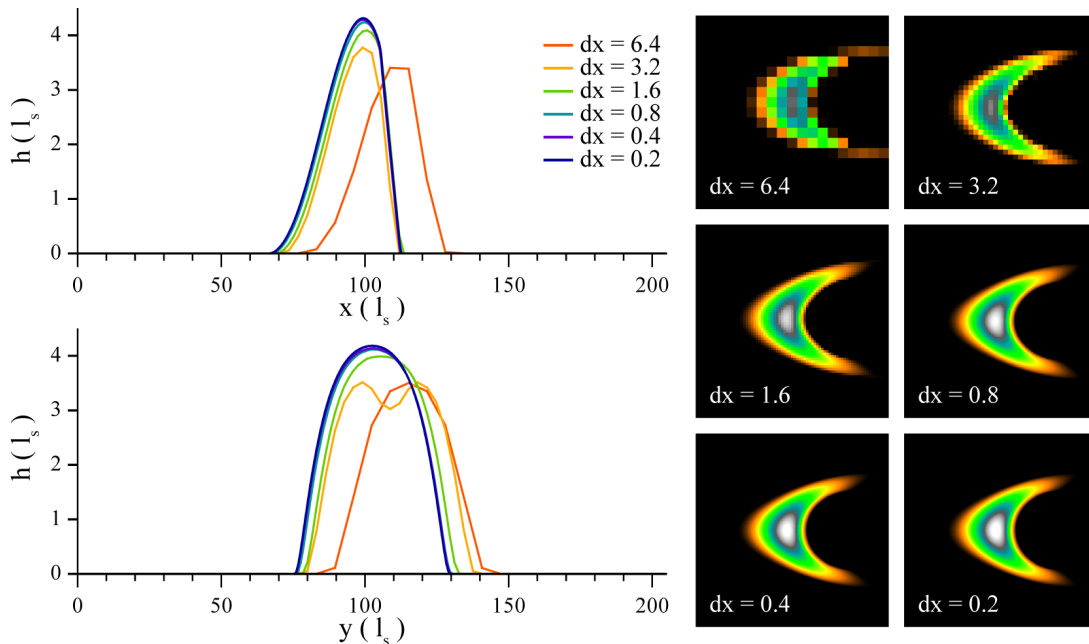
FIG. 2.14: Étude du pas de grille. Une série de simulations numériques est réalisée pour différentes valeurs du pas spatial de la grille de calcul. Nous voyons que pour des valeurs trop grandes de dx les profils de hauteur de la dune barchane obtenue sont forcés par ce dernier.
