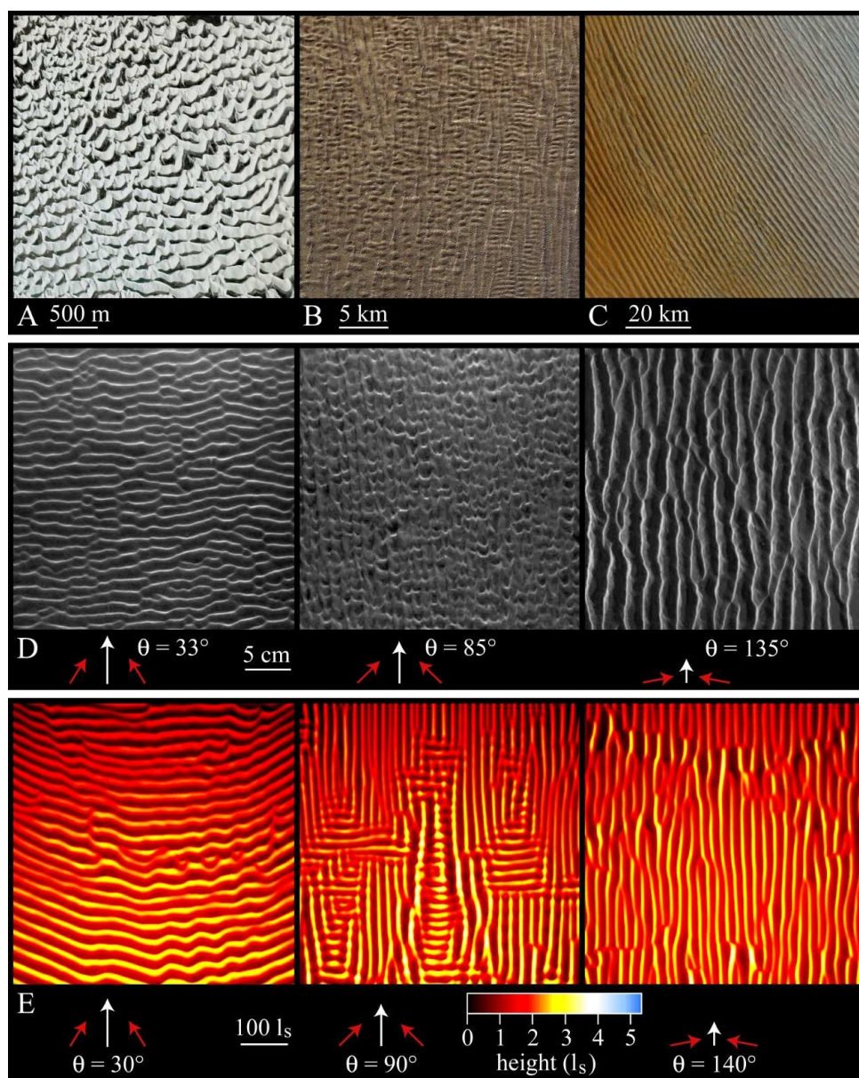
FIG. 6.1: Comparaison avec le terrain. Nous pouvons voir ici trois types de champs de dunes terrestres (A, B, C) associés à leurs analogues expérimentaux (D) et numériques (E).
