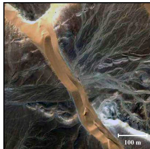
FIG. 1.12: Lee dune dans le désert du Sinai en Egypte. Ce type de dune se forme à l'arrière d'un obstacle (ici en haut à gauche) qui modifie localement l'écoulement du vent. Image Google, coordonnées : 30.471° N, 33.851° E.
