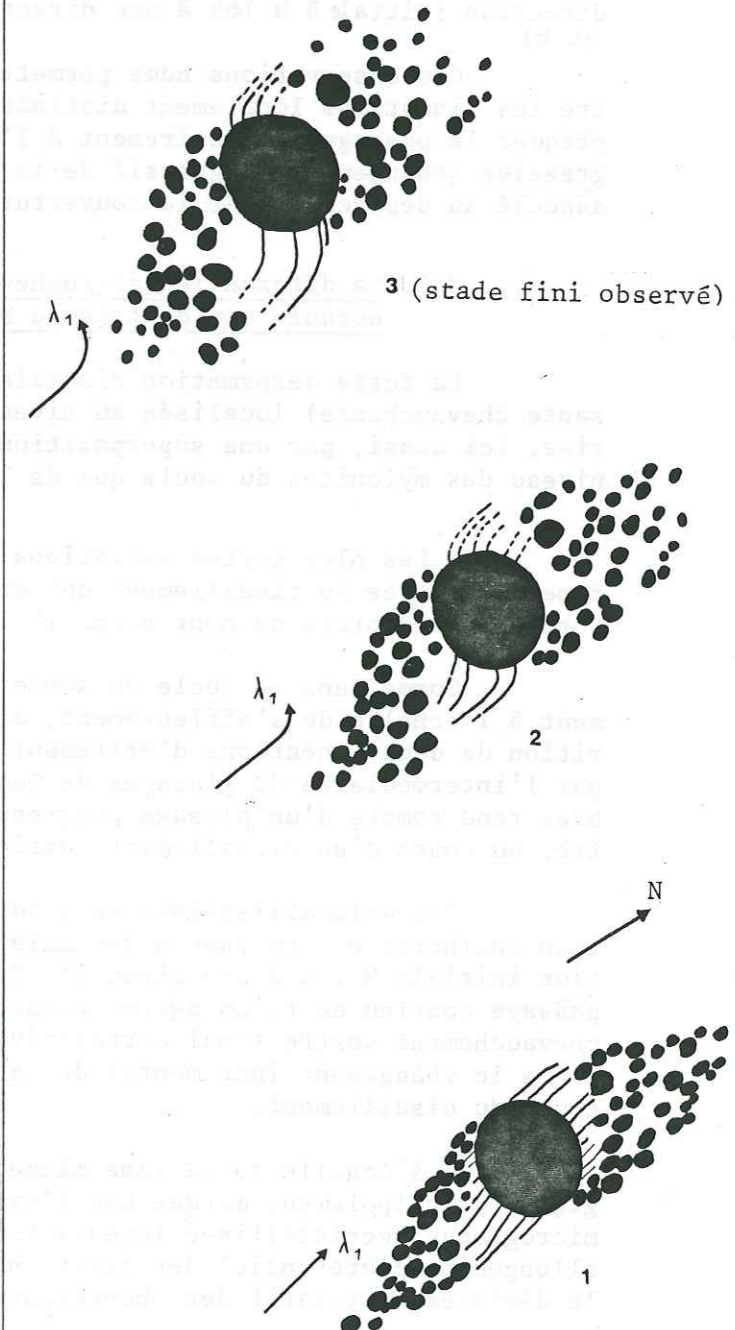
Fig. 30 : Rotation antihoraire de l'étirement principal λ 1 à la base de la nappe du Mont Joly. (croissance anti-axiale des fibres de quartz à partir d'une pyrite)
