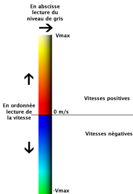
FIG. 2.17 – Echelle pour la traduction des images TDI en vitesse
