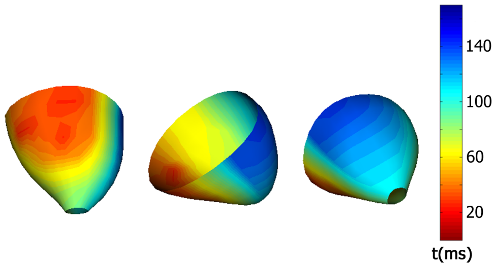
FIG. 4.26 – Une surface triangulée d'un épicaide. Les temps de dépolarisation (codés par la couleur) sont calculés pour chaque sommet après une simulation du potentiel transmembranaire grâce aux équations de Aliev et Panfilov.
