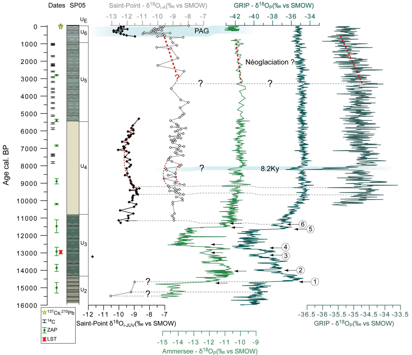
Figure 87. Comparaison et essai de corrélation des enregistrements isotopiques du lac Saint-Point ( \delta^{18}\text{O}_{\text{I-JUV}} et \delta^{18}\text{O}_{\text{I-A}} ), de l'Ammersee et de GRIP (Groenland) ; éléments de datation de la séquence SP05 ; événements climatiques majeurs : 1-Dryas ancien/Bølling, 2-Dryas moyen, 3-oscillation de Gerzensee, 4-Allerød/Dryas récent, 5-Préboréal/Dryas récent, 6-oscillation préboréale (PBO), PAG-Petit Âge Glaciaire.
