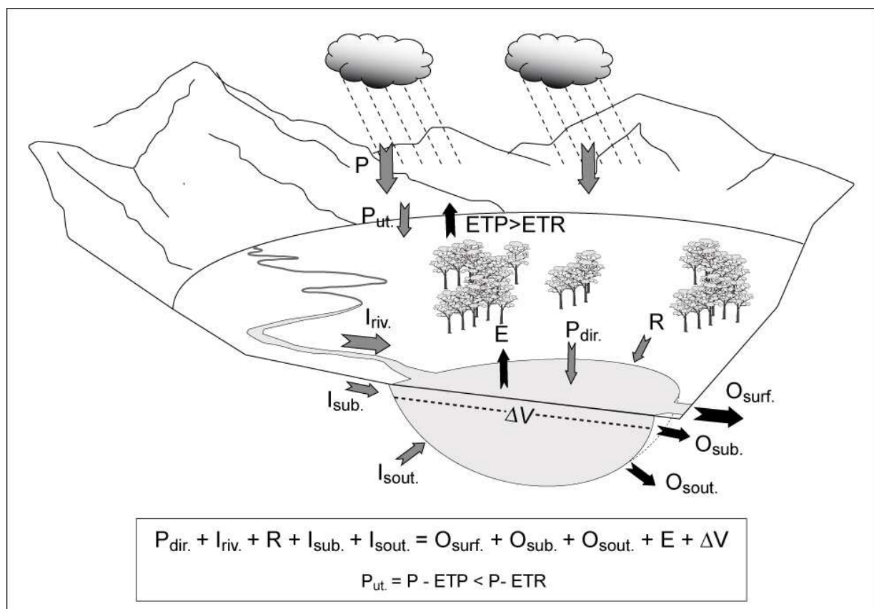
Figure 17. Termes du bilan hydrique ; P_{dir} : précipitations sur la surface du lac ; I_{riv} : apports de surface par les cours d'eau ; O_{surf} : pertes à l'exutoire ; R : ruissellement ; O/I_{sub} : apports de subsurface ; O/I_{sout} : apports/pertes sous-lacustres ; E : évaporation ; \Delta V : variation du volume du lac.
