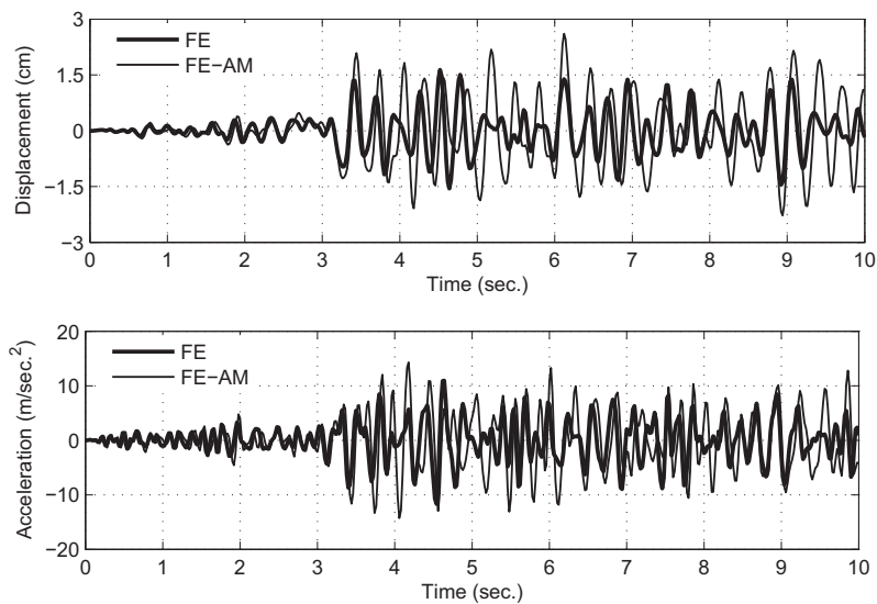
Figure 5.7 : Réponse temporelle des déplacements et accélérations en crête
