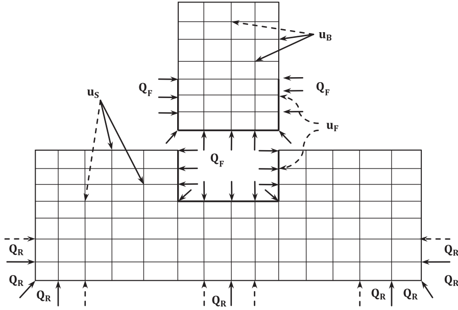
Figure 2.5 : Sous-Structure
