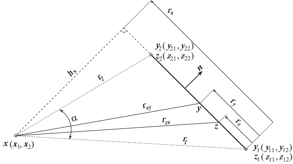
Figure 4.6 : Cas de singularité YZ : élément contenant y et z
