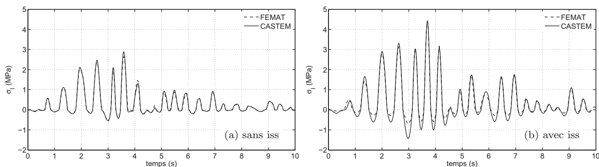
Figure 2.11 : Variations de la contrainte maximale au pied amont du barrage
