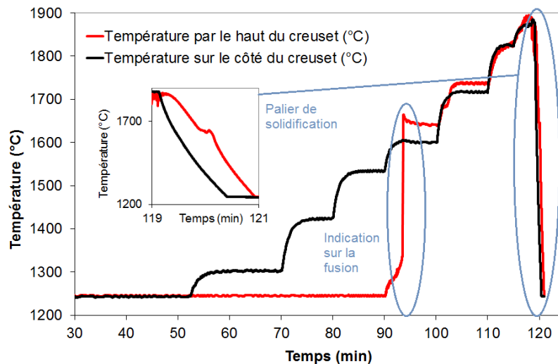
Figure 6-41 : Courbe de températures (température en fonction de la durée de l'essai) enregistrée au cours de l'essai CORSICCA 2_Al_3b relatif à l'interaction 30% UO_2 – 33% Al_2O_3 – 37% Eu_2O_3 (composition massique) dans un creuset en UO_2 . La température maximale de l'essai était de 1870 \pm 35^\circ C . Un palier de solidification est visible au refroidissement.
