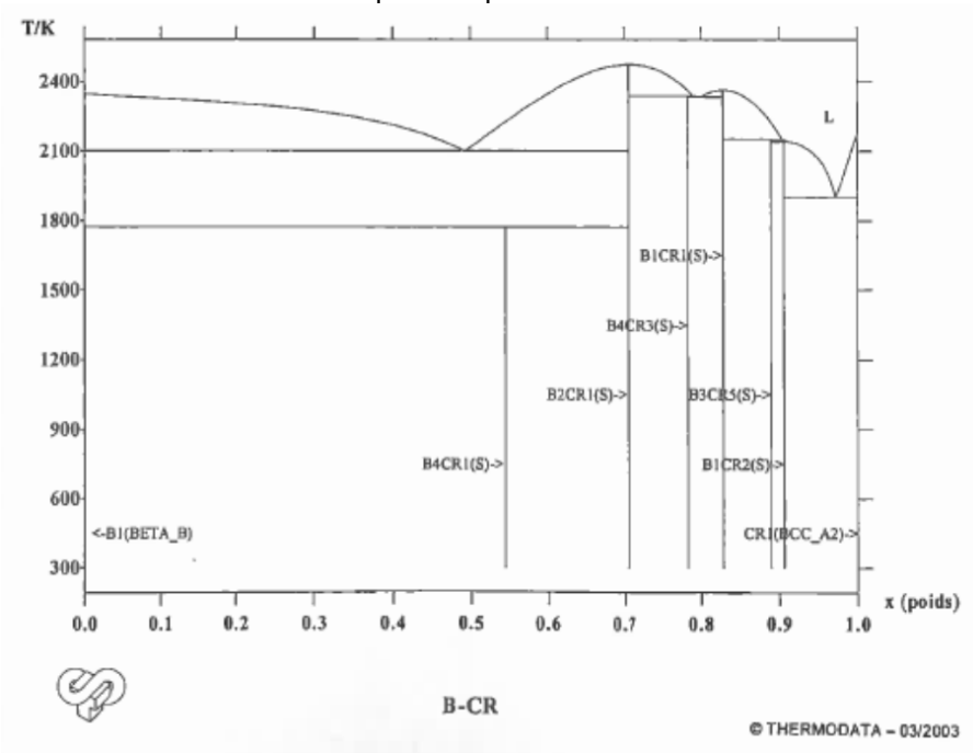
Figure A4-2 : Diagramme de phases B-Cr contenu dans la base de données Nuclea – Critère de qualité = parfait
