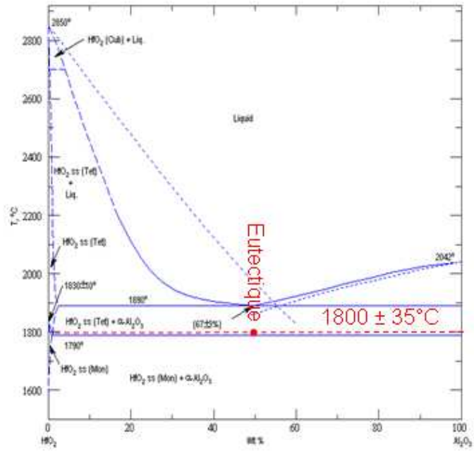
Figure 6-56 : Diagramme de phases binaire \text{HfO}_2 – \text{Al}_2\text{O}_3 modifié à partir de l'essai CORSICCA 2_Hf_1
