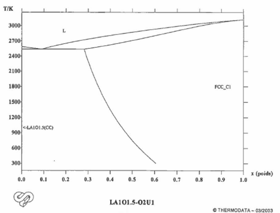
Figure A4-10 : Diagramme de phases La_2O_3 - UO_2 contenu dans la base de données Nuclea – Critère de qualité = acceptable
