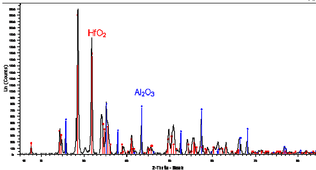
Figure A17-5 : Spectre DRX relatif à l'essai CORSICCA 2_Hf_1a – interaction 50% HfO 2 – 50% Al 2 O 3 en masse dans un creuset en tungstène
