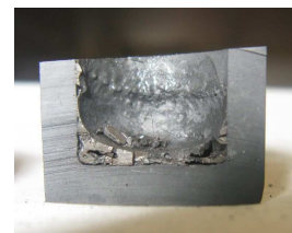
Figure A16-10 : Section longitudinale du creuset en graphite initialement revêtu de ZrC, après l'essai d'étude du mélange 40 wt% Al 2 O 3 + 60 wt% UO 2 . Le revêtement n'a pas résisté à la charge portée à 2000°C (± 35°C). La carburation de la charge a eu lieu.
