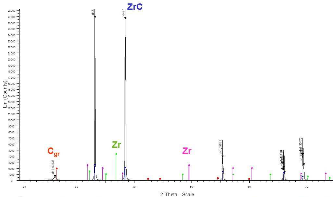
Figure 5-18 : Spectre DRX du revêtement en carbure de zirconium. Le revêtement est du ZrC pur. Il n'y a plus de trace de zirconium : tout le zirconium a réagi.
