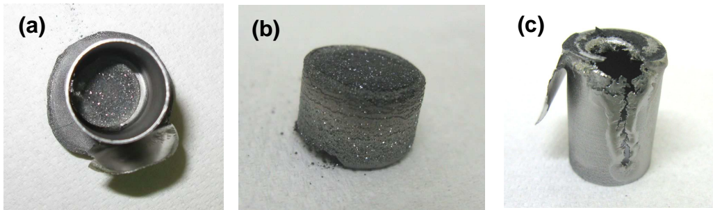
Figure 6-17 : (a) Vue du creuset en tungstène contenant la charge UO_2 - B_4C après le chauffage jusqu'à 2400°C et le refroidissement (b) Charge UO_2 - B_4C correspondante (c) Creuset à l'envers – le fond du creuset a commencé à fondre. Le diamètre externe du creuset est de 20 mm.
