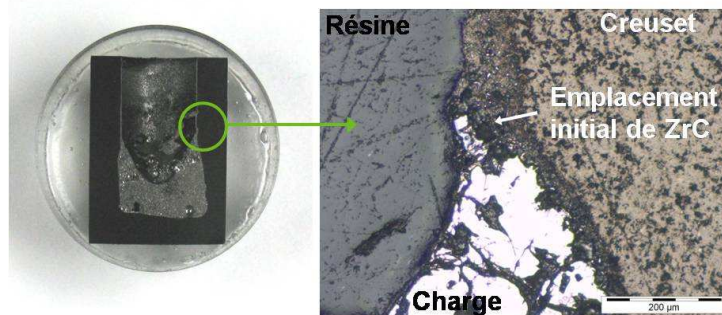
Figure A16-1 : Section longitudinale du creuset en graphite initialement revêtu de ZrC, après l'essai d'étude du mélange Acier inoxydable – B 4 C. Le creuset a été attaqué par la charge.
