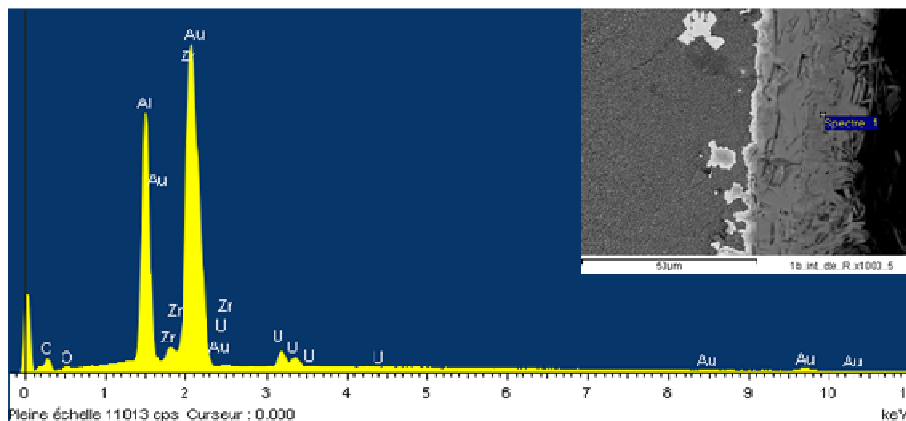
Figure 5-25 : Spectre en énergie de l'analyse de l'interface essai CORSICCA 2_Al_1b (60%wt UO_2 -40%wt Al_2O_3 , creuset graphite + ZrC, métallisation or)
