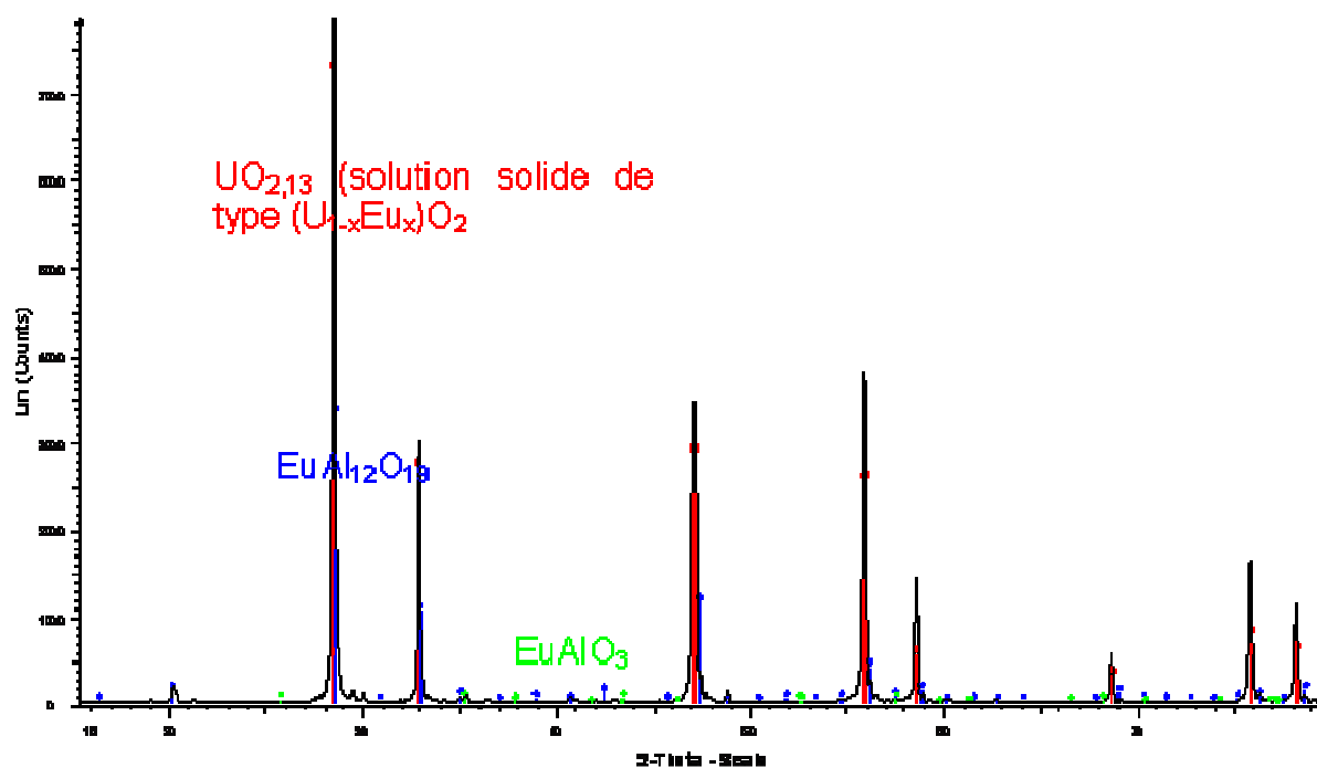
Figure A17-6 : Spectre DRX relatif à l'essai CORSICCA 2_Al_3b – interaction 30% UO 2 – 33% Al 2 O 3 – 50% HfO 2 en masse dans un creuset en UO 2
