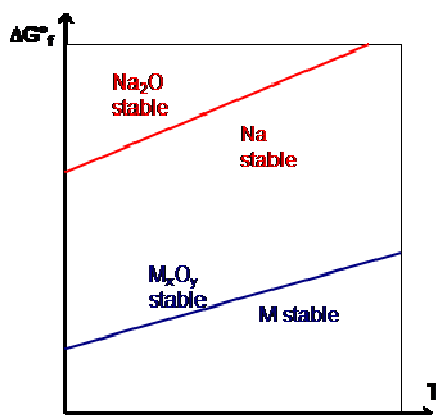
Figure A1-1 : Diagramme d'Ellingham schématisé mettant en évidence la compatibilité sodium – oxyde
