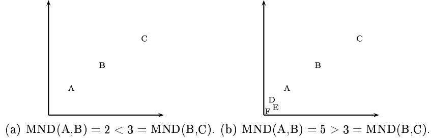
FIG. A.1 – Illustration de l'intérêt de la Mutual Neighbor Distance .
