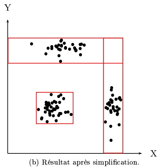
FIG. 5.3 – Exemple de simplification des règles.
