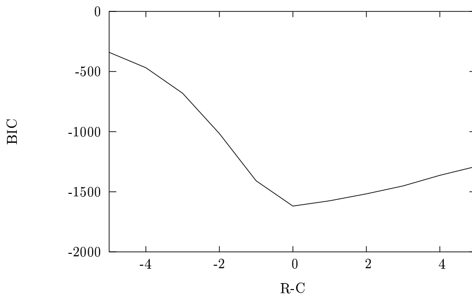
FIG. 7.4 – Évolution de la valeur du critère BIC en fonction du nombre R de dimensions sélectionnées pour chaque cluster.
