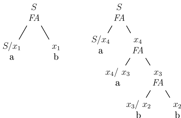
FIG. 5.6 – résultat de la première étape de l’algorithme RG à D = \{ab, aabb\}
