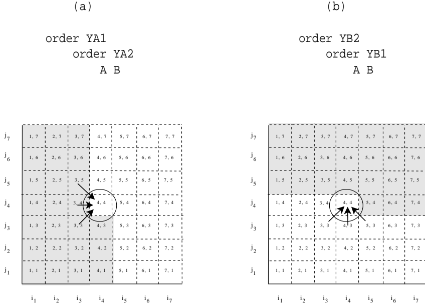
FIG. 4.3 – Parcours donné par deux directives order imbriquées et sa visualisation sur un espace de dimension 7 \times 7 . Le point de grille I = (i, j) = (4, 4) est le point de l'itération courante. La partie de l'espace en gris et celle en blanc représentent respectivement les points de grille calculés et pas encore calculés. Les flèches sont des connexions cohérentes pour (a) et des connexions incohérentes pour (b).
