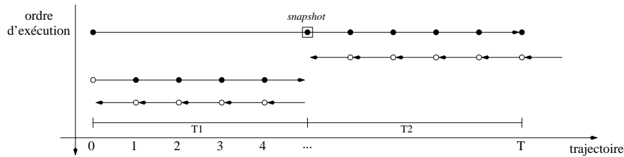
FIG. A.5 – SA avec checkpointing . Nous exécutons des procédures forward jusqu'à la fin de la trajectoire en stockant les états dans la partition de T_2 , puis nous exécutons les procédures backward jusqu'au snapshot . A partir du début de T on recommence l'exécution des procédures forward jusqu'au snapshot en stockant les états de la partition T_1 . C'est à ce moment que nous pouvons calculer les procédures backward de la partition T_1 .
