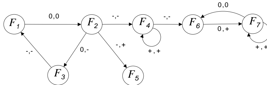
FIG. 5.10 – GDR avec des circuits et des boucles.
