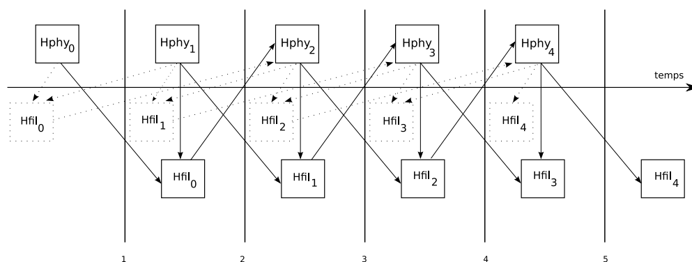
FIG. 3.10 – Décalage de la fonction Hfil d'un pas de temps sur la fenêtre temporelle. En pointillés, la figure montre la fonction Hfil au pas de temps original, en indice nous avons noté le pas de temps. Le même décalage concerne les fonctions Ufil et Vfil .
