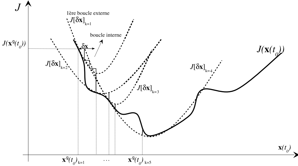
FIG. 2.2 – La courbe en trait plein correspond à la fonction de coût J(\mathbf{x}(t_0)) . Chacune des paraboles en pointillés correspond à la fonction J[\delta\mathbf{x}] initialisée à chaque itération k de la boucle externe . La boucle interne réalise une descente de gradient sur la parabole correspondant à l’approximation. La boucle externe , quant à elle, permet d’avancer en se repositionnant sur la fonction J(\mathbf{x}(t_0)) (courbe pleine) et de faire une nouvelle approximation correspondant à la parabole suivante dans la minimisation.
