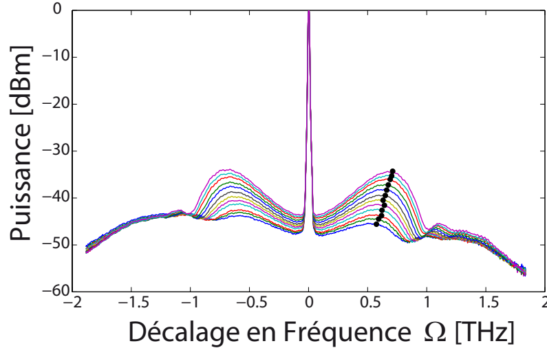
FIGURE 1.21 – Illustration de l'évolution du processus d'instabilité modulationnelle au sein d'une fibre hautement non-linéaire (HNL) pour des puissances de l'onde continue variant de 450 mW à 1 W. Les valeurs théoriques du gain maximal pour chaque puissance est donné par les points noirs.
