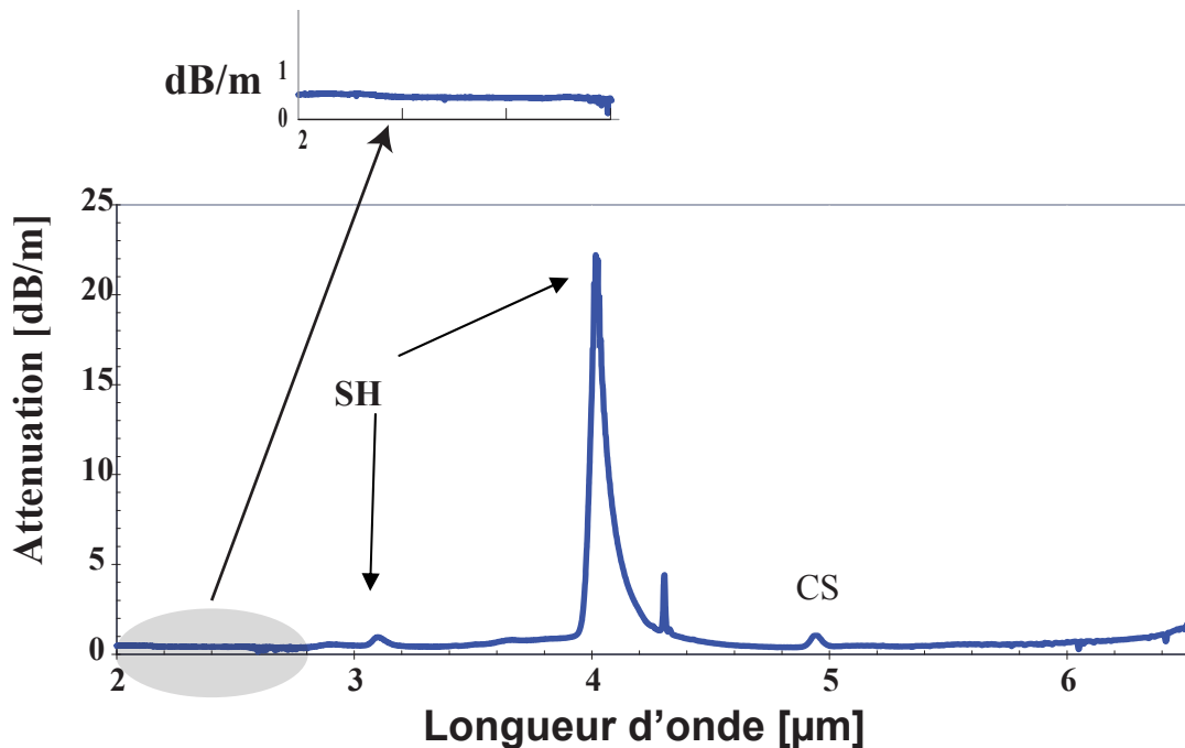
FIGURE 1.14 – Diagramme d'atténuation d'une fibre chalcogénure AS_2S_3 .
