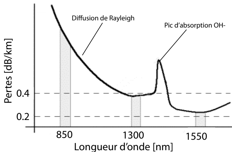
FIGURE 1.5 – Évolution de l'atténuation (dB/km) d'une fibre optique en fonction de la longueur d'onde.
