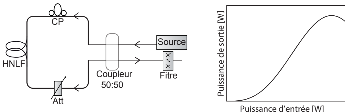
FIGURE 2.3 – Schéma de principe d'un montage basé sur une boucle à miroir non-linéaire (NOLM) associé à sa fonction de transfert typique en puissance.
