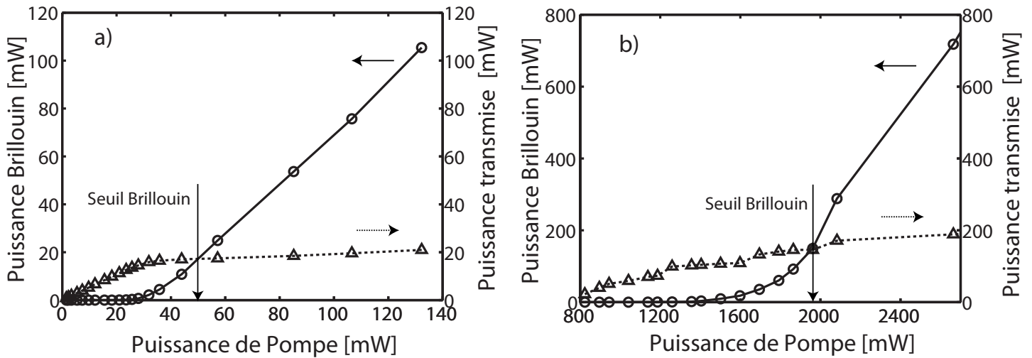
FIGURE 3.21 – Puissance rétrodiffusée ( trait plein ) et puissance transmise ( trait pointillé ) en fonction de la puissance de pompe injectée a) dans la fibre standard et b) dans la fibre GeSbS 2
