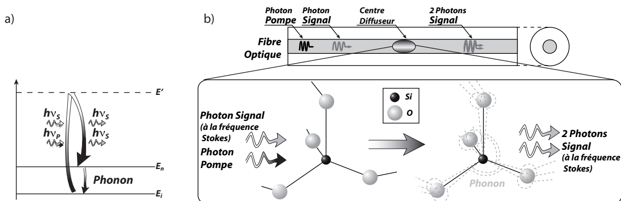
FIGURE 1.26 – Illustration du principe de diffusion Raman au sein d'une fibre optique silice pure [28]. a) Transitions énergétiques à la base de la diffusion Raman stimulée. b) Diffusion Raman stimulée Stokes.
