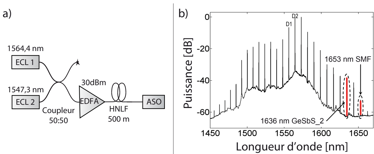
FIGURE 3.26 – a) Montage expérimental pour la création des graines d'amplifications Raman par mélanges à quatre ondes. b) Spectre en sortie de la fibre HNLf : mélanges à quatre ondes multiples. D1 et D2 représentent les longueurs d'ondes des diodes ECL1 et ECL2 du schéma 3.27.
