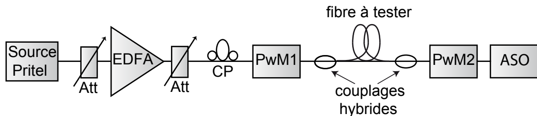
FIGURE 3.32 – Montage expérimental pour la mesure de spectres d'auto-modulation de phase dans la fibre As_2S_3 .
