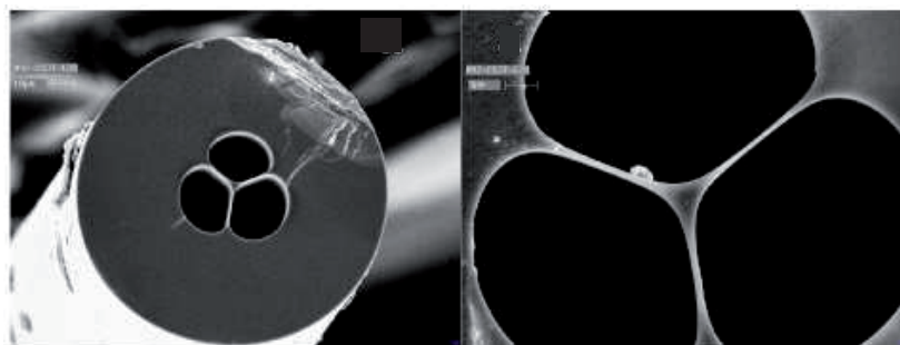
FIGURE 3.30 – Images faites au microscope électronique à balayage de la fibre chalcogénure As_2S_3 à cœur suspendu de diamètre de cœur de 2,6 \mu m .
