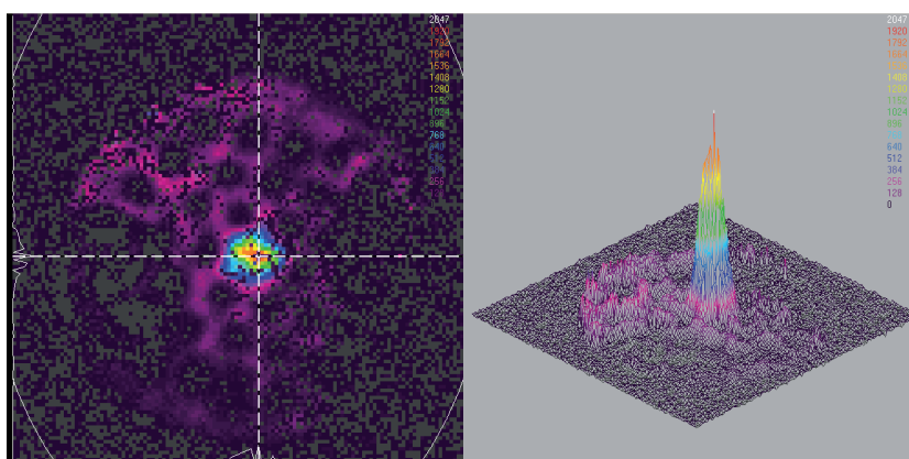
FIGURE 3.13 – Profil de modes d'une fibre chalcogénure microstructurée 3 couronnes \text{Ge}_{15}\text{Sb}_{20}\text{S}_{65} . à gauche : profil de modes ,à droite : représentation du profil de mode en 3 dimensions.
