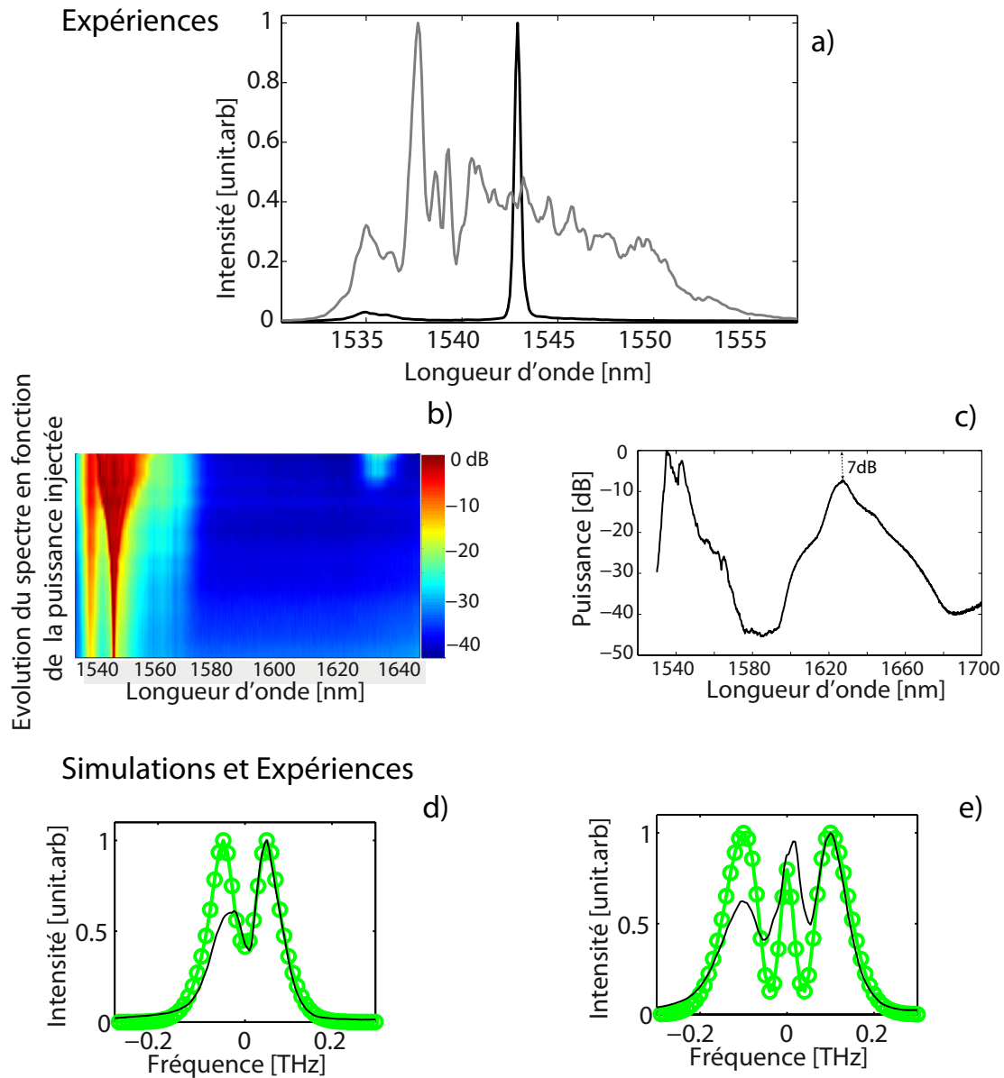
FIGURE 3.33 – Résultats de caractérisation de l'effet de SPM dans la fibre à cœur suspendu \text{As}_2\text{S}_3 a) Spectres expérimentaux : ( courbe noire ) pour une puissance crête de 1,5 W et ( courbe grise ) pour une puissance injectée de 14.5 dBm. b) Évolution des spectres en fonction de la puissance crête variant de 1,5 W à 150 W insert : zoom sur la partie 1520 nm 1580 nm. c) Continuum avec bosse Raman pour une puissance crête de 212 W. d) Comparaison des résultats de simulations ( trace et marqueurs verts ) et expérimentaux ( trace noire ) pour une puissance crête de 35 W et e) 67 W.
