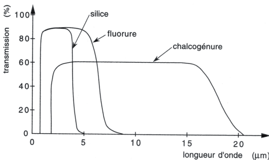
FIGURE 1.9 – Schéma illustrant les différents domaines de transmission pour diverses familles de verres pour un barreau de 10 cm de : silices, fluorures et chalcogénures [15].
