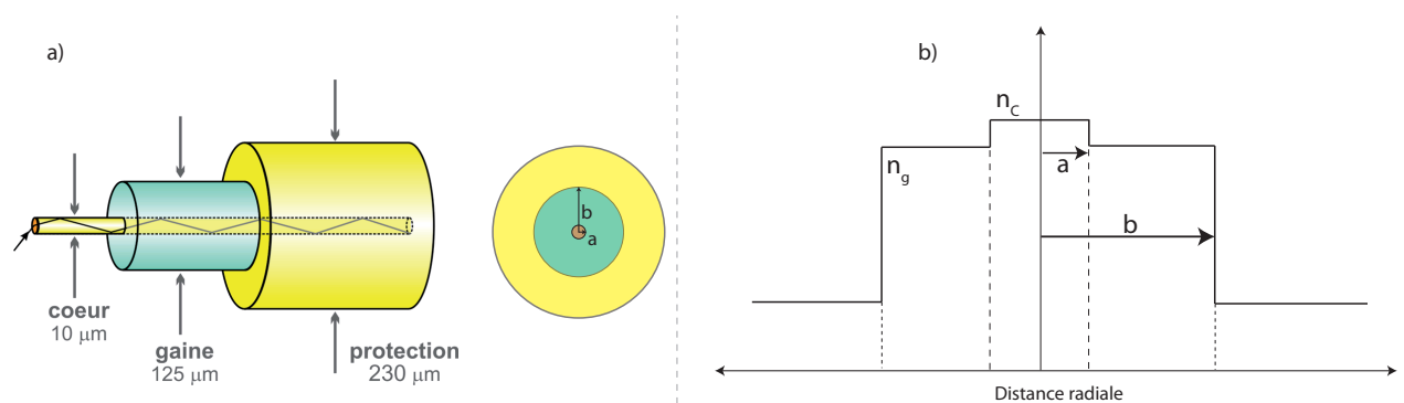
FIGURE 1.2 – a) Schéma d'une structure de fibre optique classique dopée : vue en trois dimensions et vue de face. b) Évolution transverse de l'indice de réfraction pour une fibre à saut d'indice.
