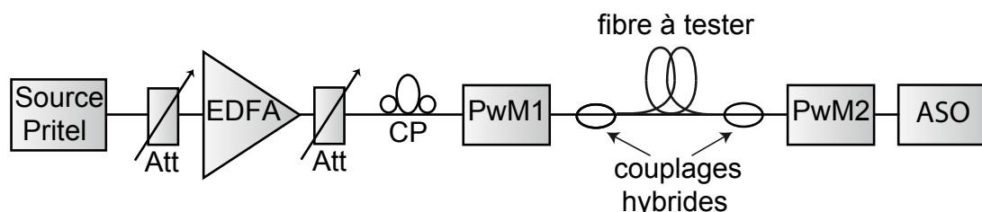
FIGURE 3.17 – Montage expérimental pour la mesure d'auto-modulation de phase dans les fibres chalcogénures microstructurées 3 couronnes à trous \text{GeSbS}_1 et \text{GeSbS}_2
