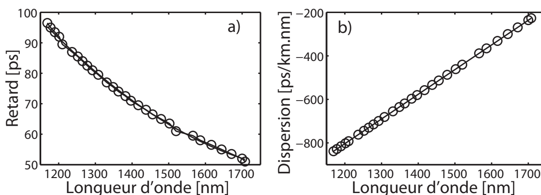
FIGURE 3.16 – Détermination de la dispersion pour la fibre GeSbS 2 . a) Évolution du retard introduit en fonction de la longueur d'onde de la frange centrale b) Valeur de la dispersion chromatique en fonction de la longueur d'onde . rond : points expérimentaux , trait continu : ajustement linéaire.
