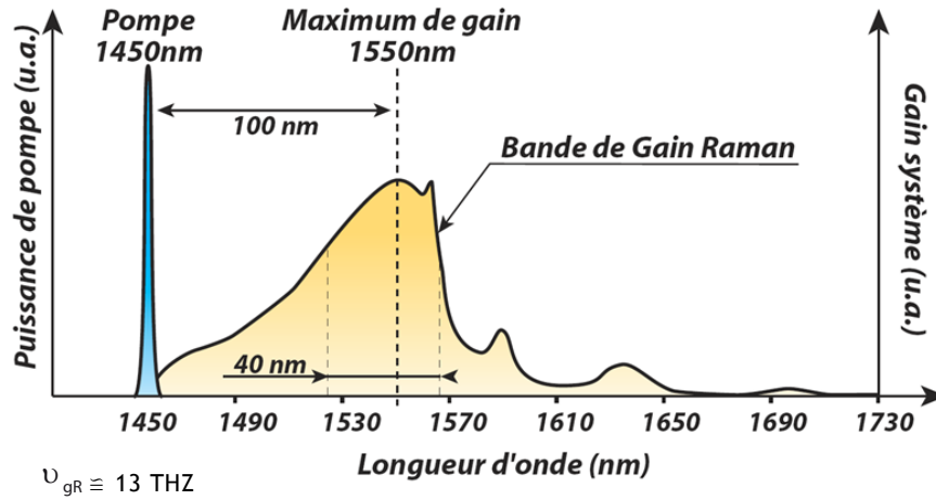
FIGURE 1.27 – Illustration du spectre de gain Raman dans une fibre silice pour une longueur d'onde de pompe de 1450 nm [28, 29].
