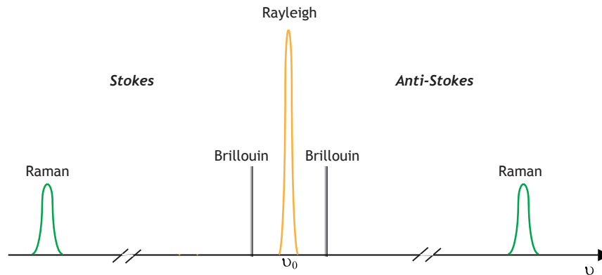
FIGURE 1.23 – Représentation fréquentielle conventionnelle des diffusions spontanées générées dans un milieu diffusant.
