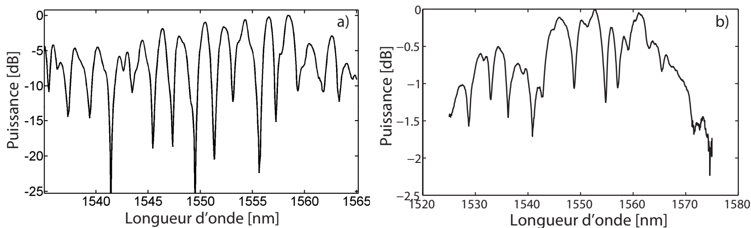
FIGURE 3.15 – Mesure du DGD a) fibre GeSbS 1 b) fibre GeSbS 2
