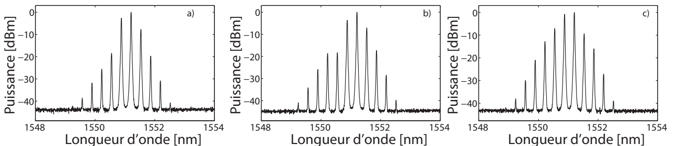
FIGURE 4.14 – Etudes des spectres optiques en sortie du circulateur pour différentes puissances injectées sur le dispositif AS-1 pour un train d'impulsions de largeur à mi-hauteur 5 ps. a) 15 dBm, b) 18 dBm, c) 20 dBm.
