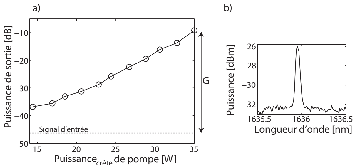
FIGURE 3.29 – Évolution de la puissance du signal de sortie en fonction de la puissance du signal de pompe pour la fibre \text{GeSbS}_2 de 1,5 m de long. b) Spectre du signal de sortie amplifié pour une puissance de pompe de 24,5 W.
