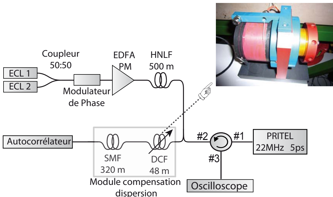
FIGURE 4.23 – Montage expérimental du module de compensation de dispersion.
