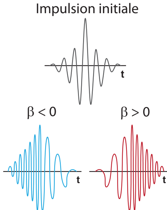
FIGURE 1.20 – Illustration de l'interaction des phénomènes de dispersion et de SPM au sein d'une fibre optique. Évolution du 'chirp' d'une pulsation optique FT, 'chirpée' lors de sa propagation dans une fibre à dispersion normale ( trace bleue ) et anormale ( trace rouge ).
