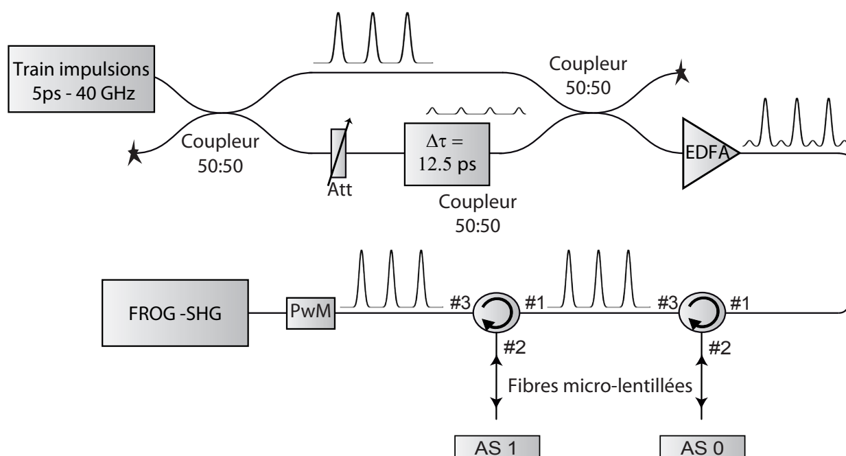
FIGURE 4.20 – Montage expérimental pour la caractérisation de l'association des dispositifs AS-0 et AS-1.
